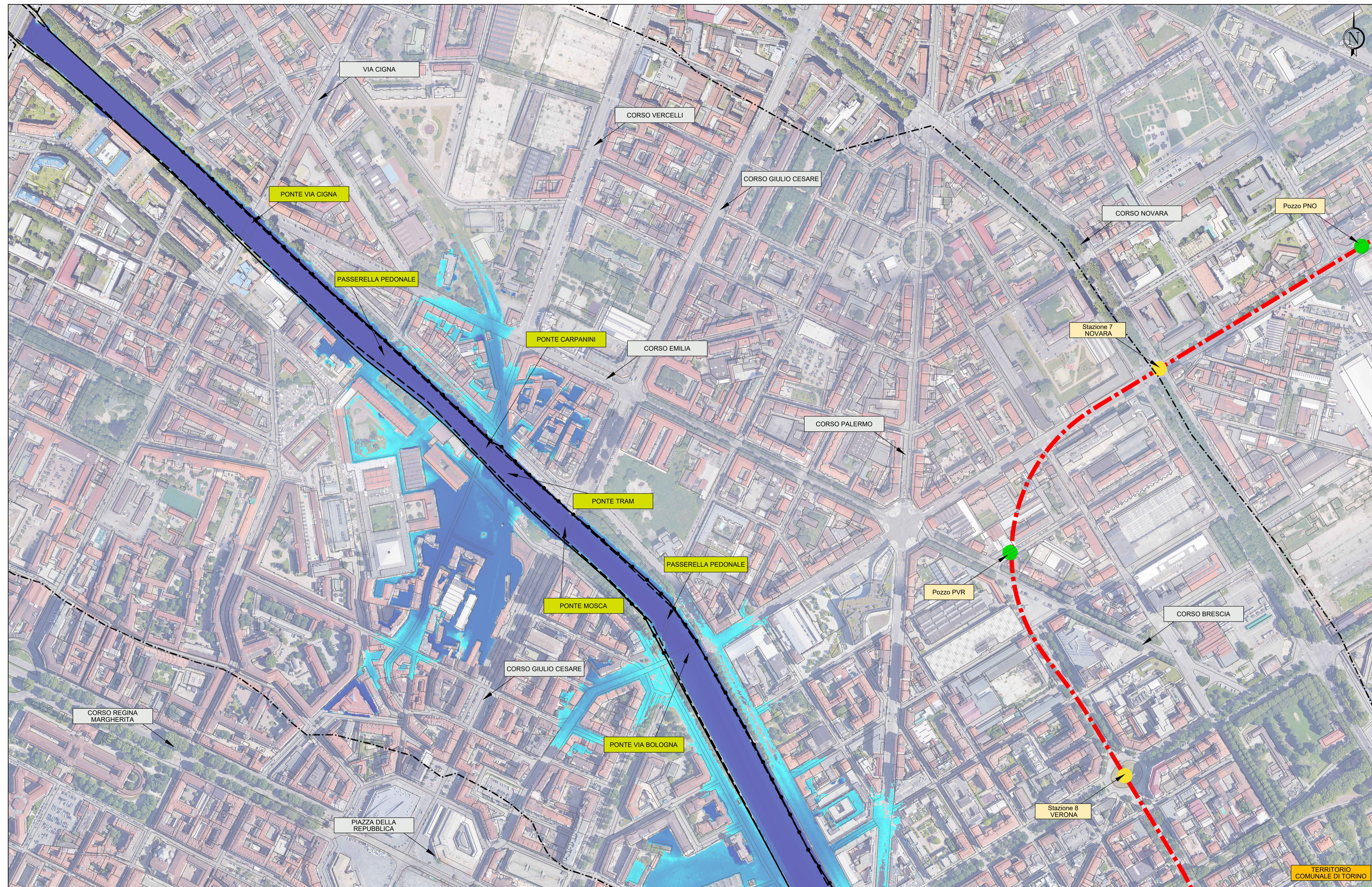
TIRANTI IDRAULICI MASSIMI PER UN EVENTO DI PIENA TR 200 ANNI, IN CONDIZIONI ATTUALI IN ASSENZA DI CASSA DI LAMINAZIONE A MONTE E PARZIALE OSTRUZIONE DEL PONTE DI VIA ROSSINI Base carta: BDTRE Regione Piemonte, Ortofoto Scala 1 : 2.500
