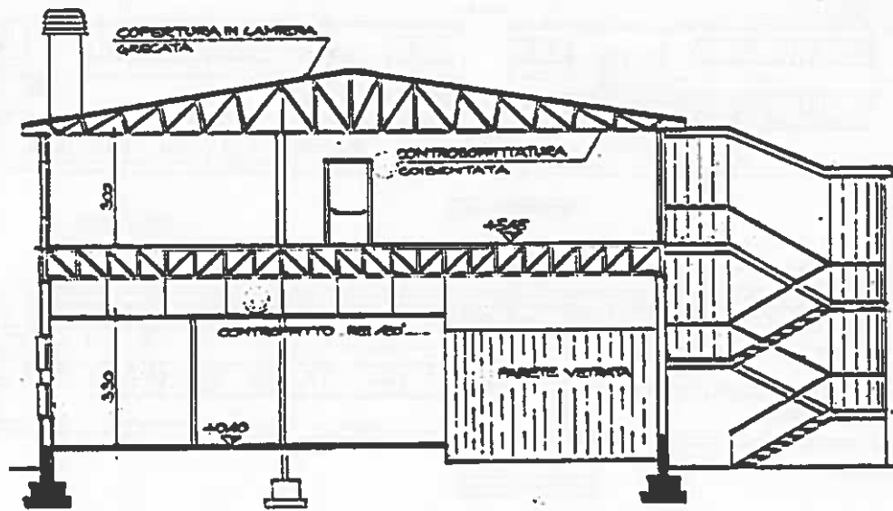
Sezione Trasversale 2
