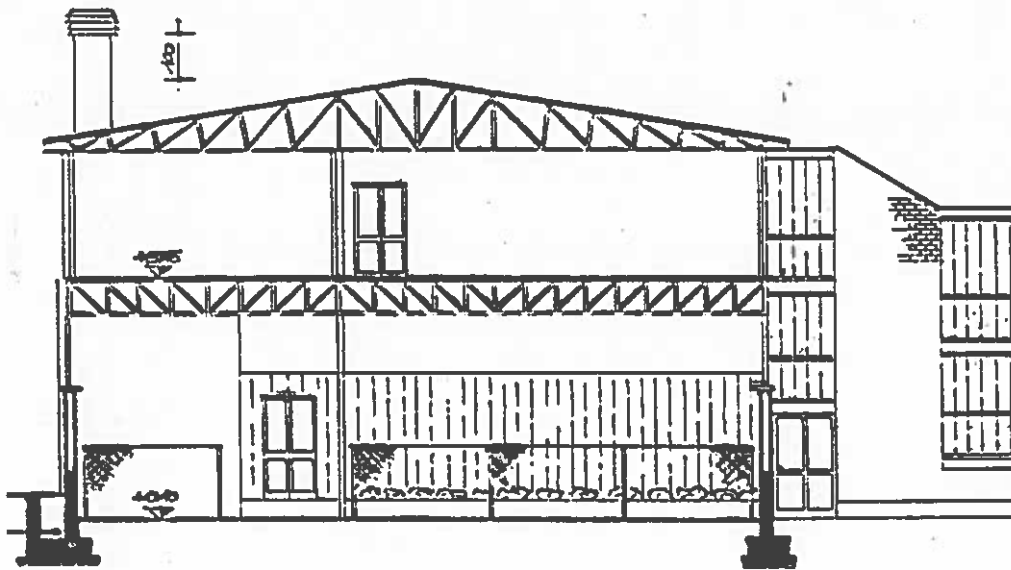
Sezione Trasversale 1
