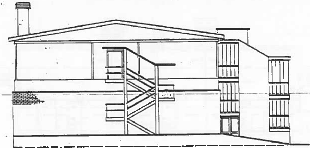
Prospetto SO
