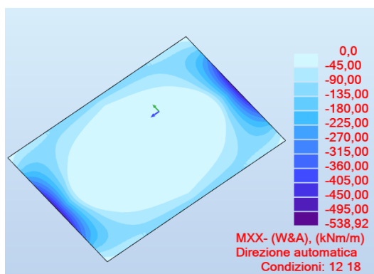
Figura 156. Momento flettente MX Lembo Superiore e MX Lembo Inferiore
