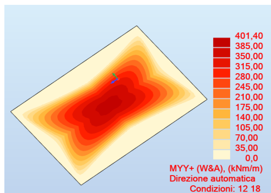
Figura 157. Momento flettente MY Lembo Superiore e MY Lembo Inferiore
