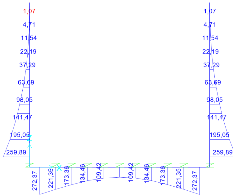
Figura 115. Momento flettente M3-3
