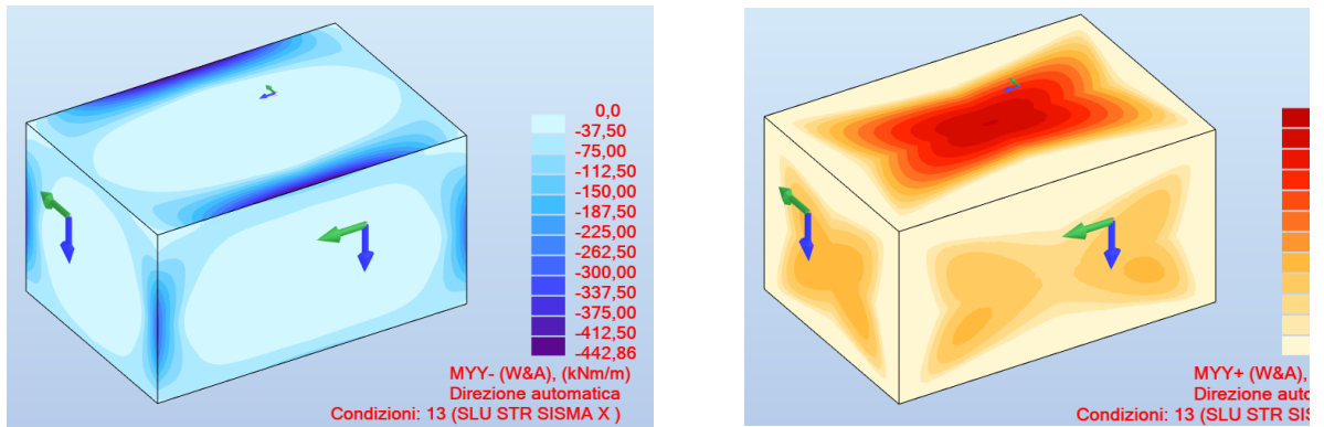
Figura 136. Momento flettente MYY Lembo superiore e MYY Lembo inferiore
