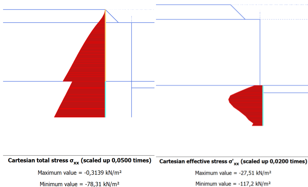
Figura 95. Tensioni orizzontali efficaci paratia - Lato monte e valle – Schema B
