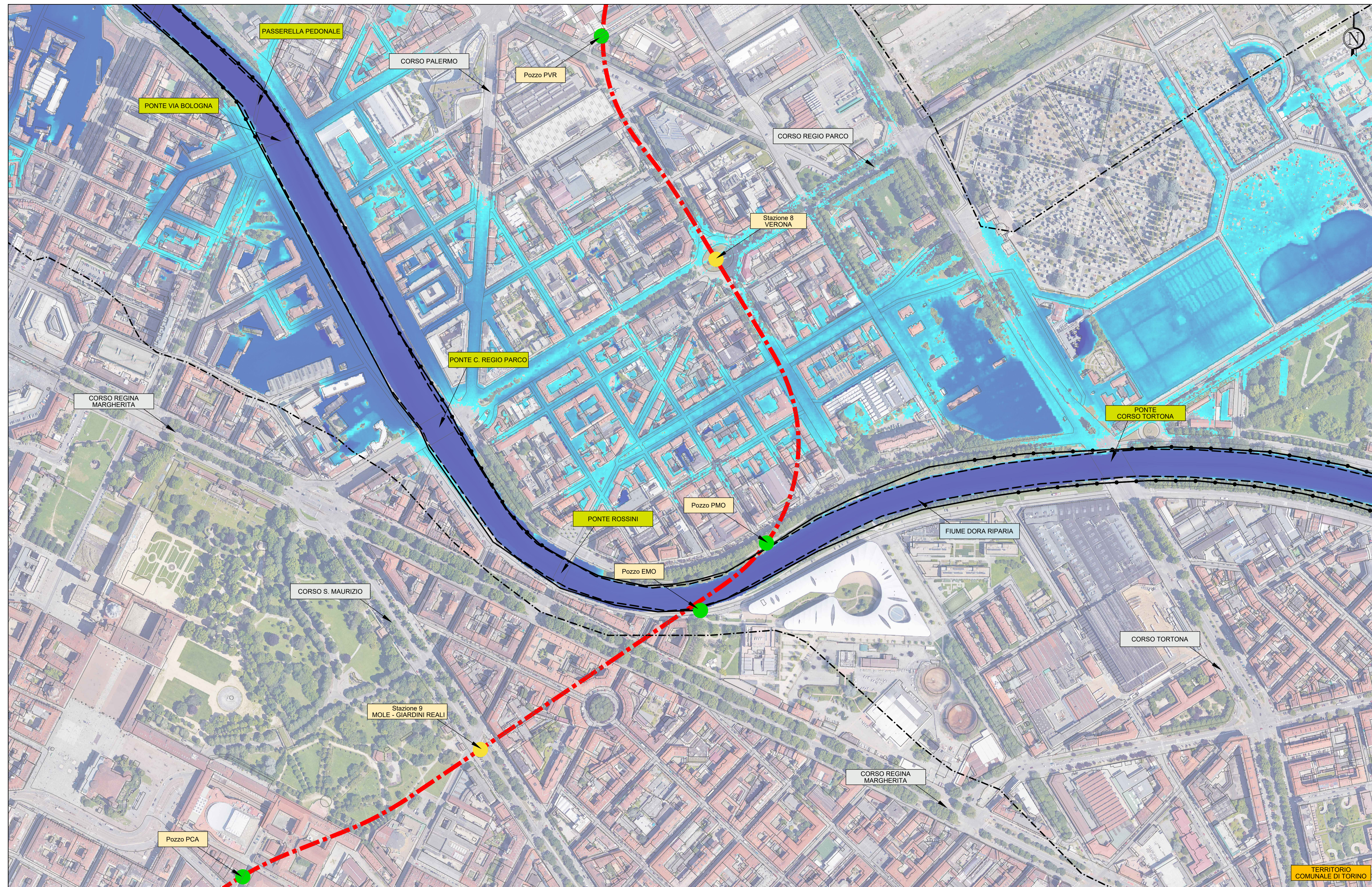
TIRANTI IDRAULICI MASSIMI PER UN EVENTO DI PIENA TR 200 ANNI, IN CONDIZIONI ATTUALI IN ASSENZA DI CASSA DI LAMINAZIONE A MONTE E PARZIALE OSTRUZIONE DEL PONTE DI VIA BOLOGNA Base carta: BDTRE Regione Piemonte, Ortofoto
