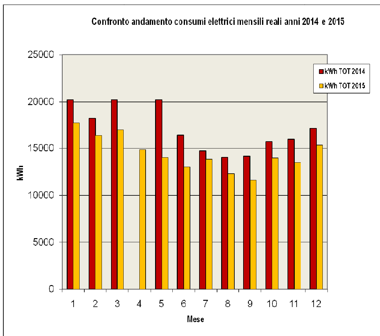
Grafico di confronto consumi mensili reali di energia elettrica per gli anni 2014 e 2015
