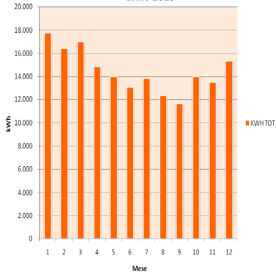
Andamento consumi elettrici mensili reali anno 2015
