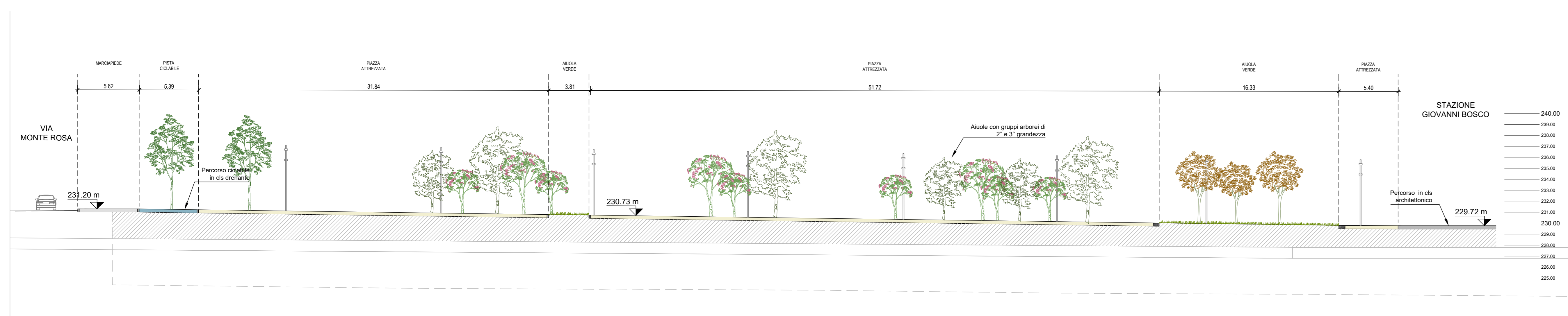
TR 2 - Sezione BB' Da Via Monte Rosa a Stazione Giovanni Bosco | scala 1:200
