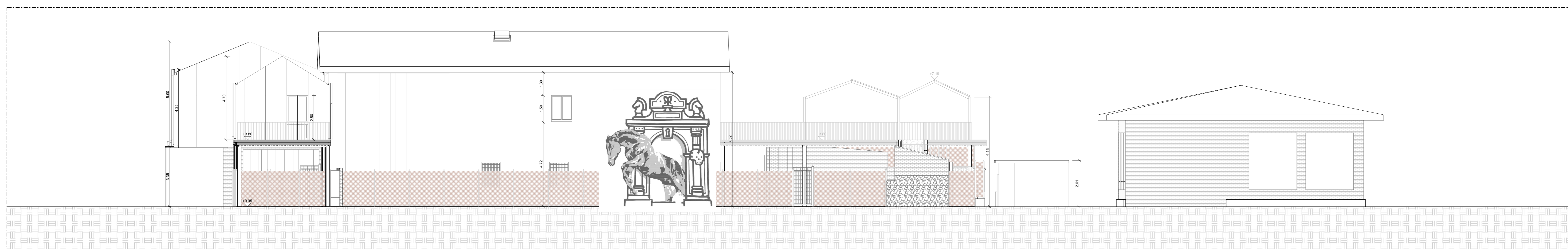
④ Prospetto Ovest_PROGETTO 1:100
