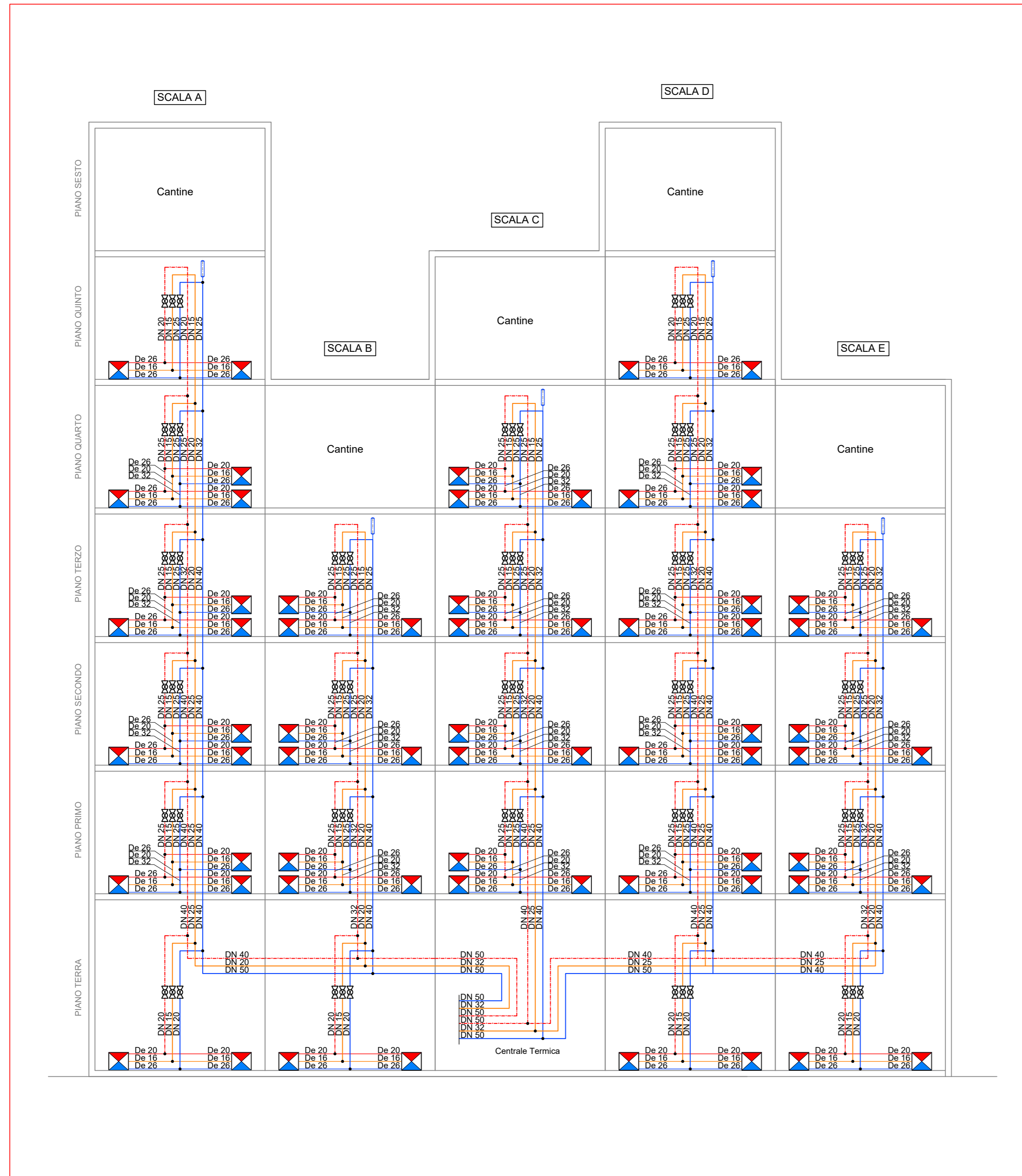
SCHEMA ALTIMETRICO IMPIANTO IDRICO
