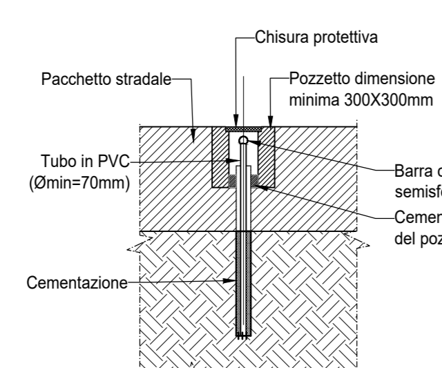
DETTAGLIO 1 PUNTO DI LIVELLAZIONE SUPERFICIALE (CPL)
