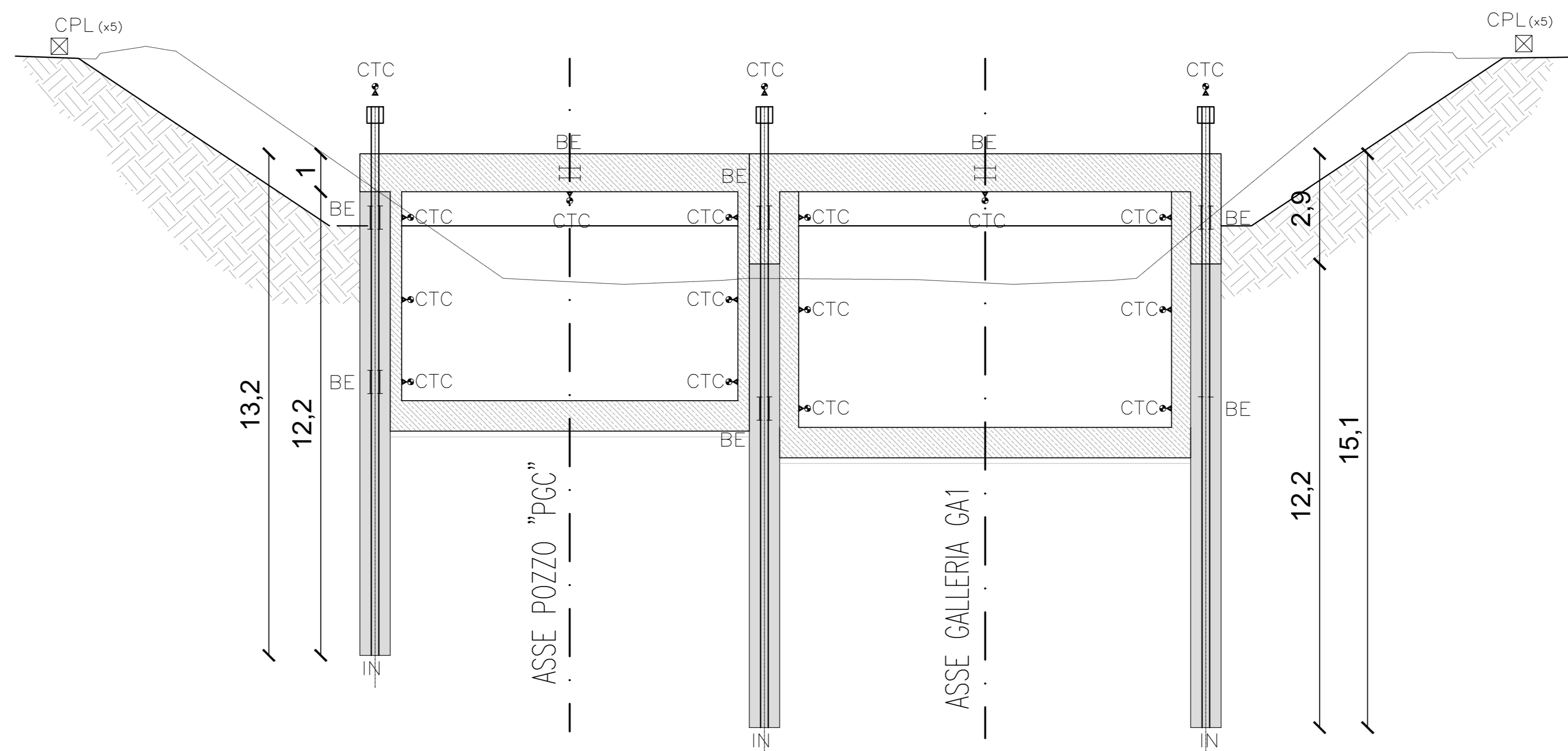
DETTAGLIO 4 SCHEMA DI POSIZIONAMENTO BARRE ESTENSIMETRICHE (BE) E TUBO INCLINOMETRO (IN)
