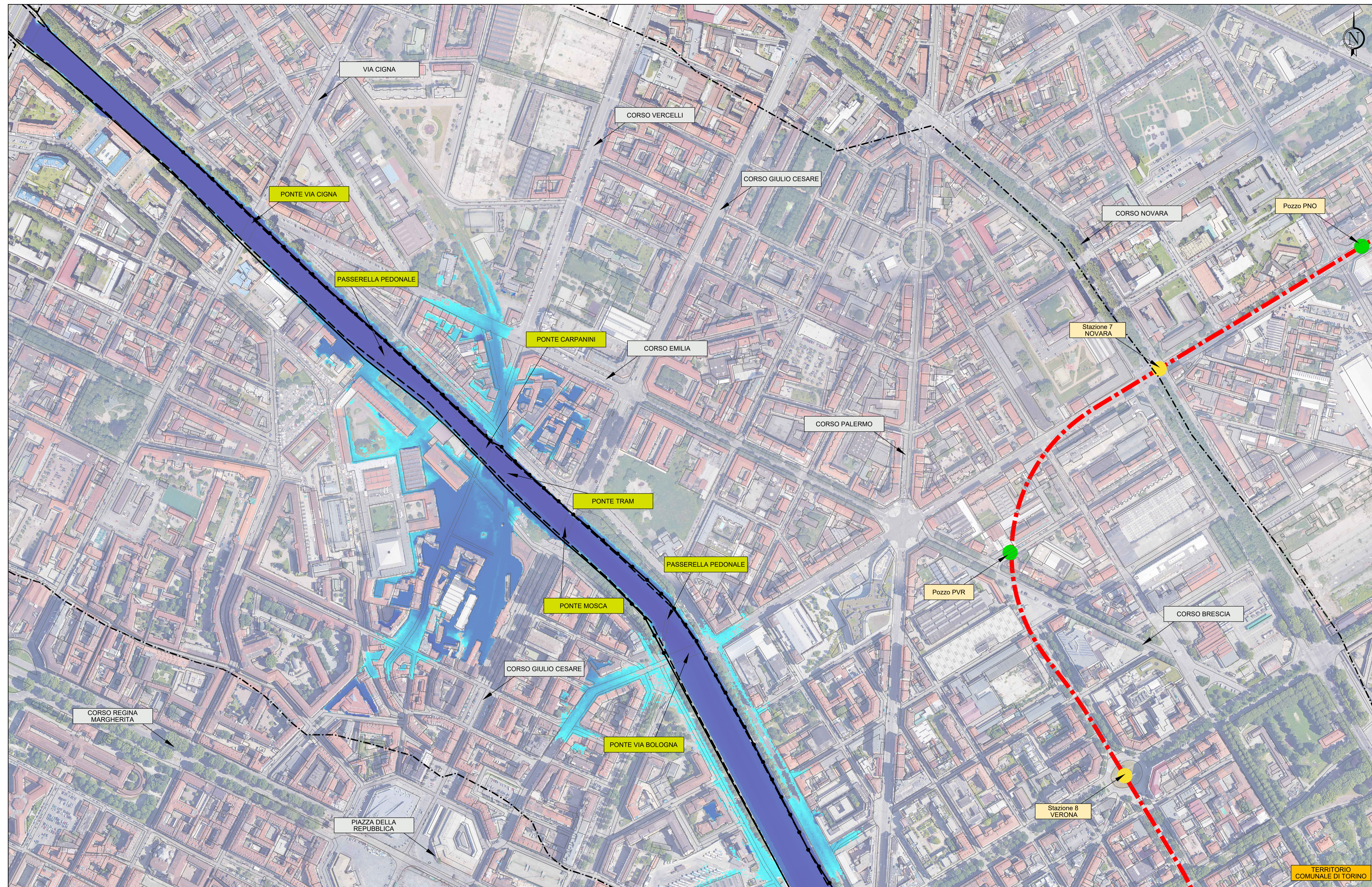
TIRANTI IDRAULICI MASSIMI PER UN EVENTO DI PIENA TR 200 ANNI, IN CONDIZIONI ATTUALI IN ASSENZA DI CASSA DI LAMINAZIONE A MONTE E PARZIALE OSTRUZIONE DEL PONTE DI VIA CIGNA Base carta: BDTRE Regione Piemonte, Ortofoto
