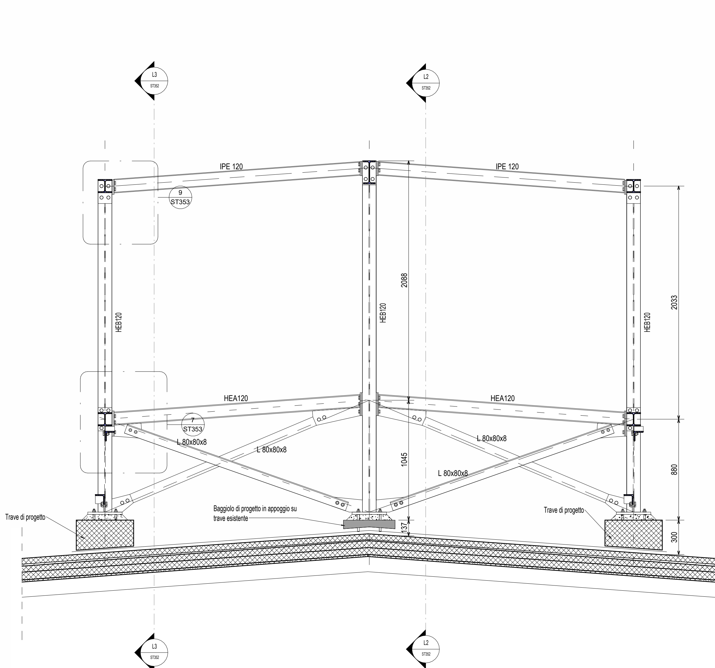
LUCERNAIO - Sezione 1 1 : 20
