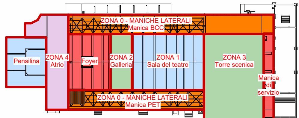
PIANTA CHIAVE 1 : 1000
