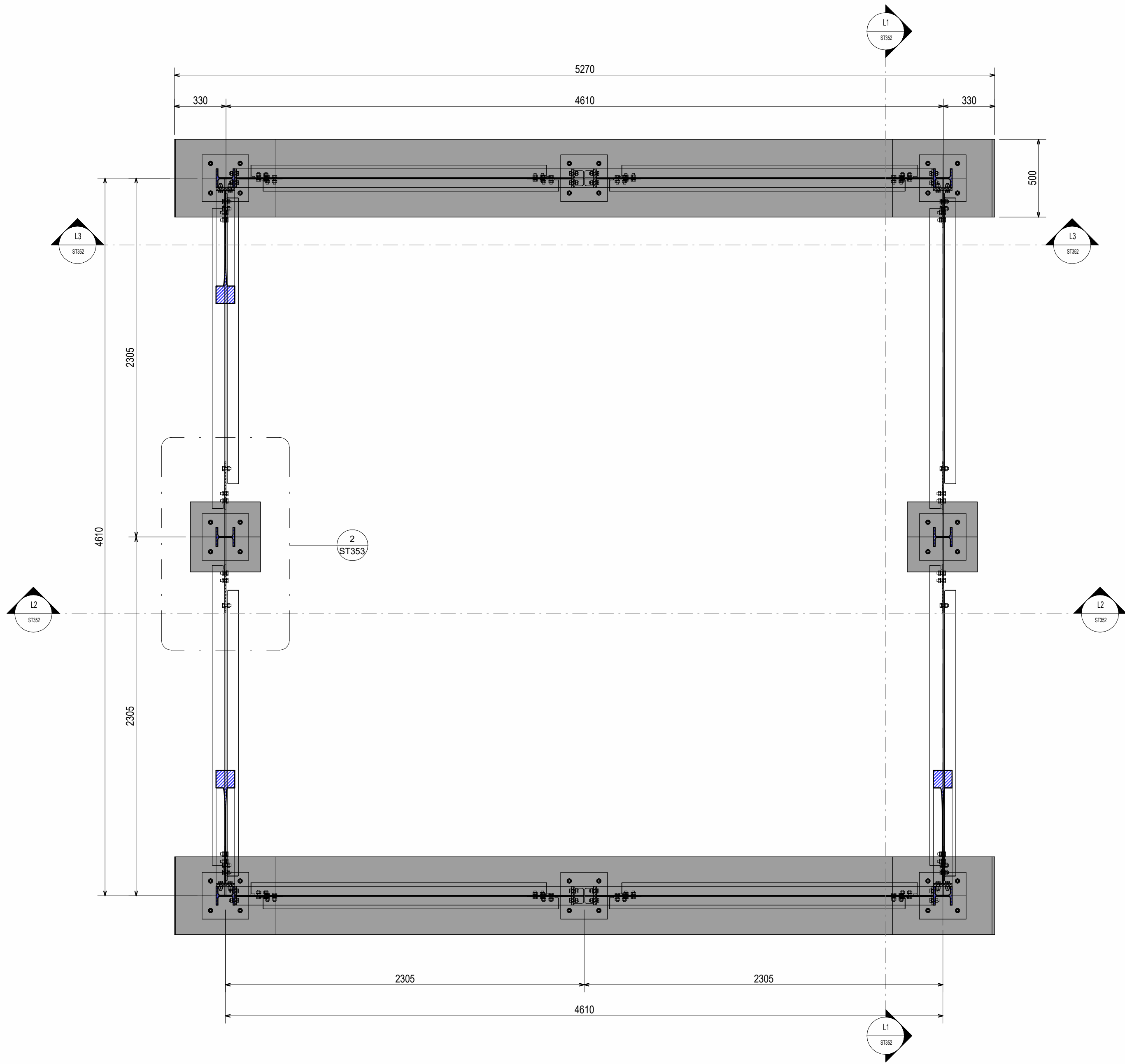
LUCERNAIO - Pianta struttura 1 : 20
