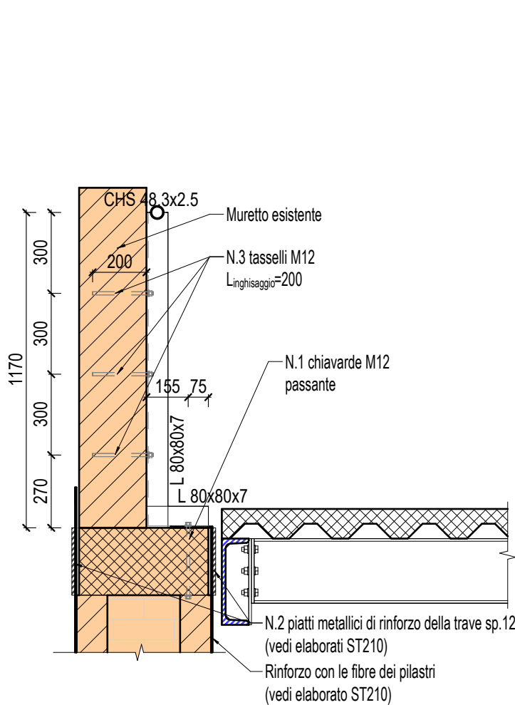
Sezione P1 Parapetti
