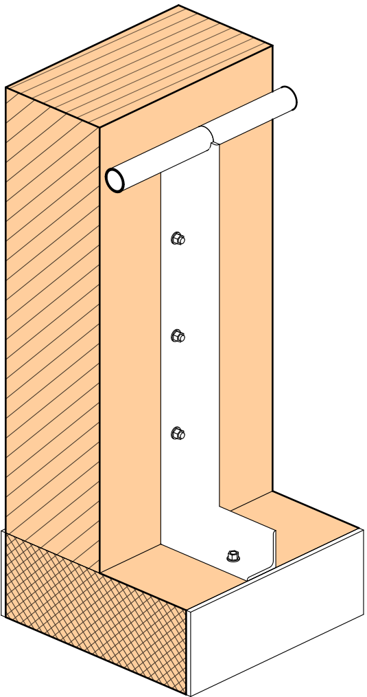
Parapetto Maniche - Vista 3D
