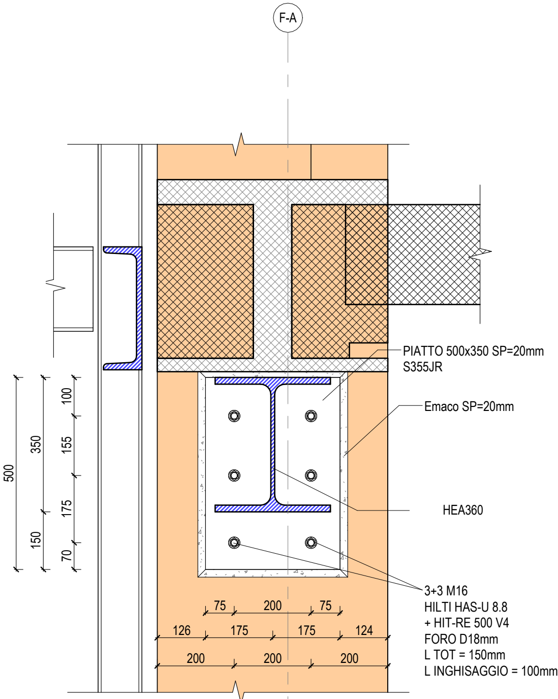
Dettaglio L - Sezione frontale 1: 10
