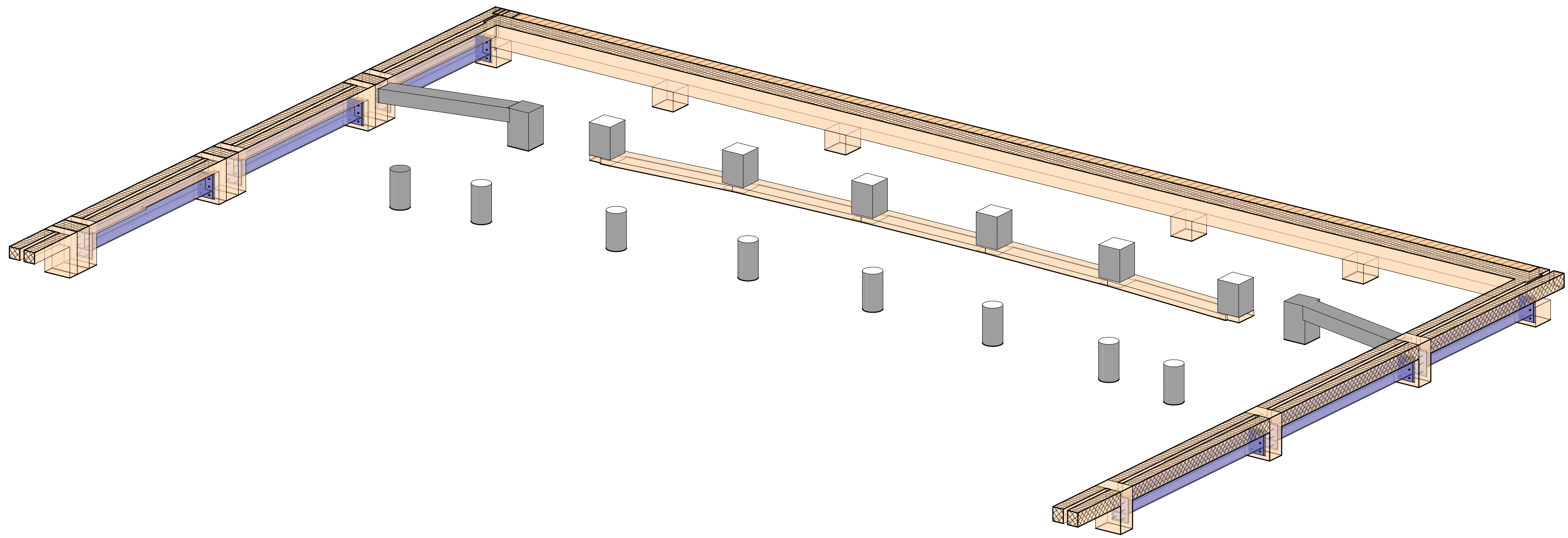
Rinforzo Trave Galleria - Vista 3D
