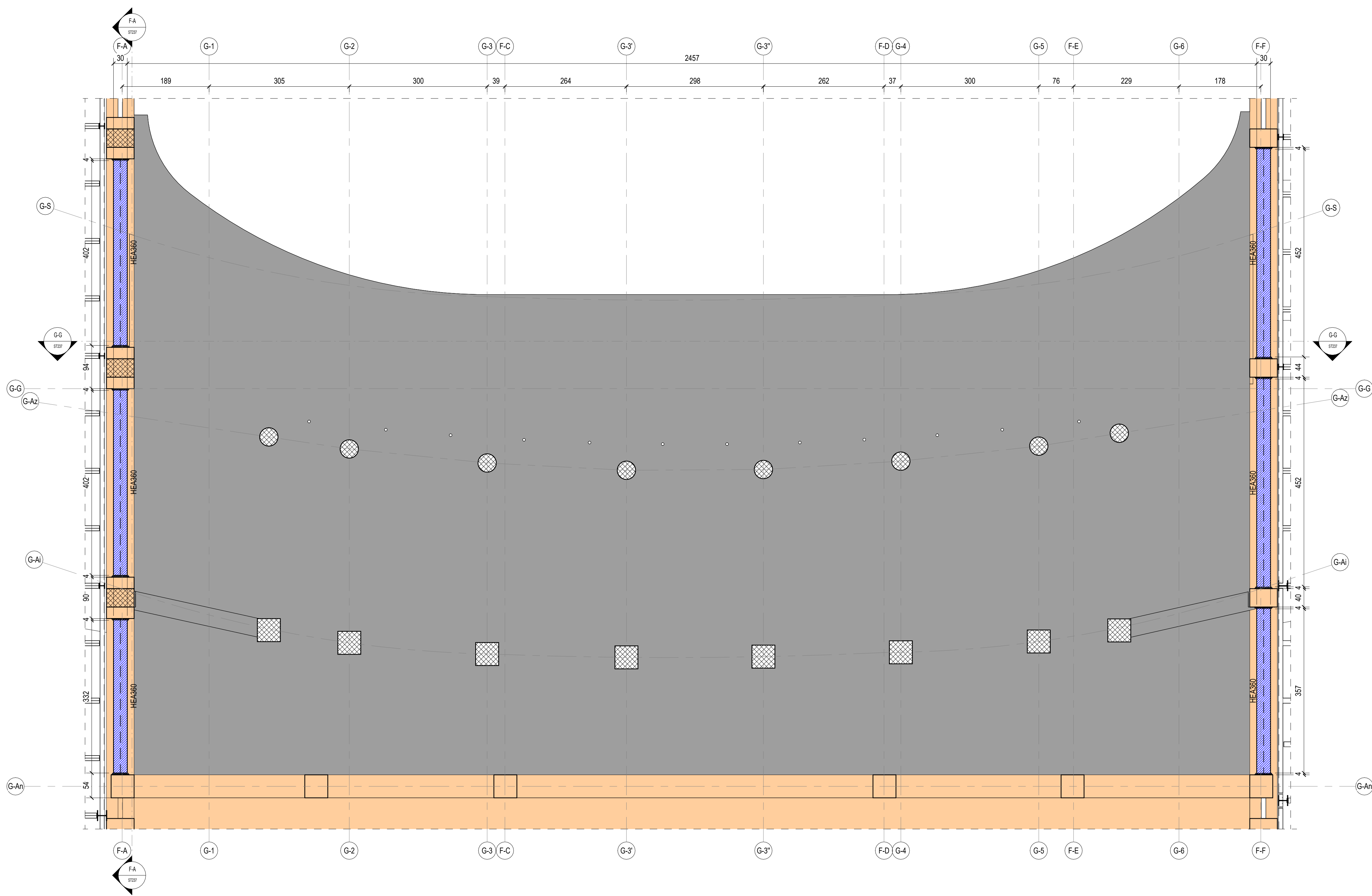
STRUTTURE - GALLERIA - RINFORZO TRAVI ESISTENTE - Pianta piano primo- vista dal basso verso l'alto 1: 50
