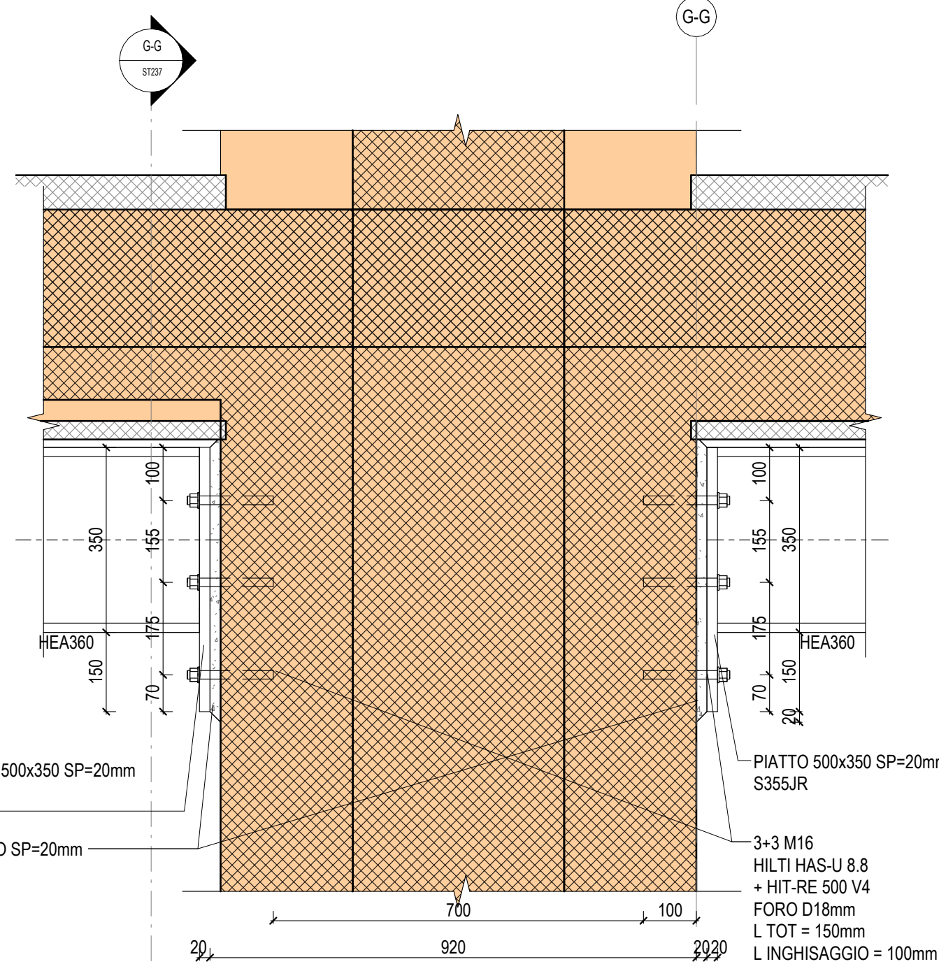
Dettaglio L - Sezione trasversale 1: 10
