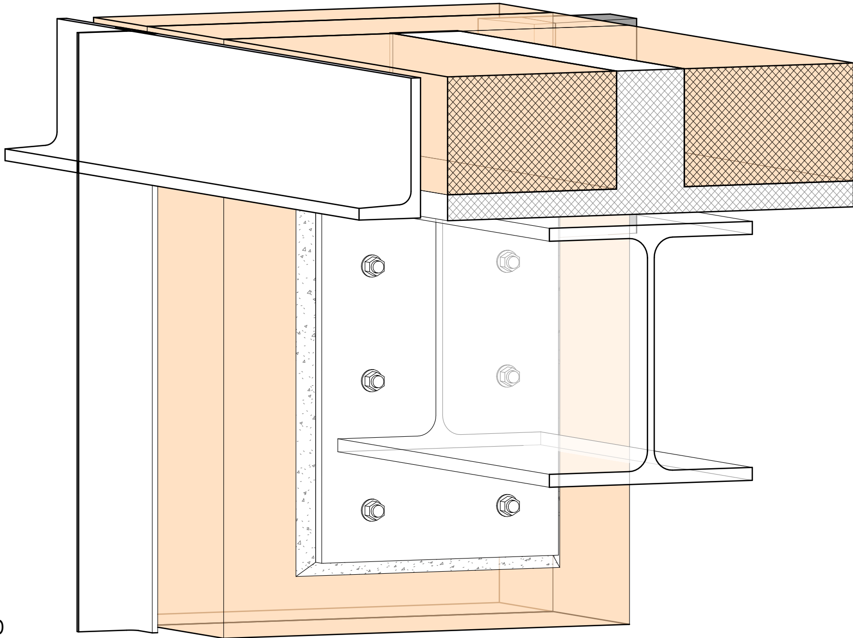
Dettaglio L - Vista 3D
