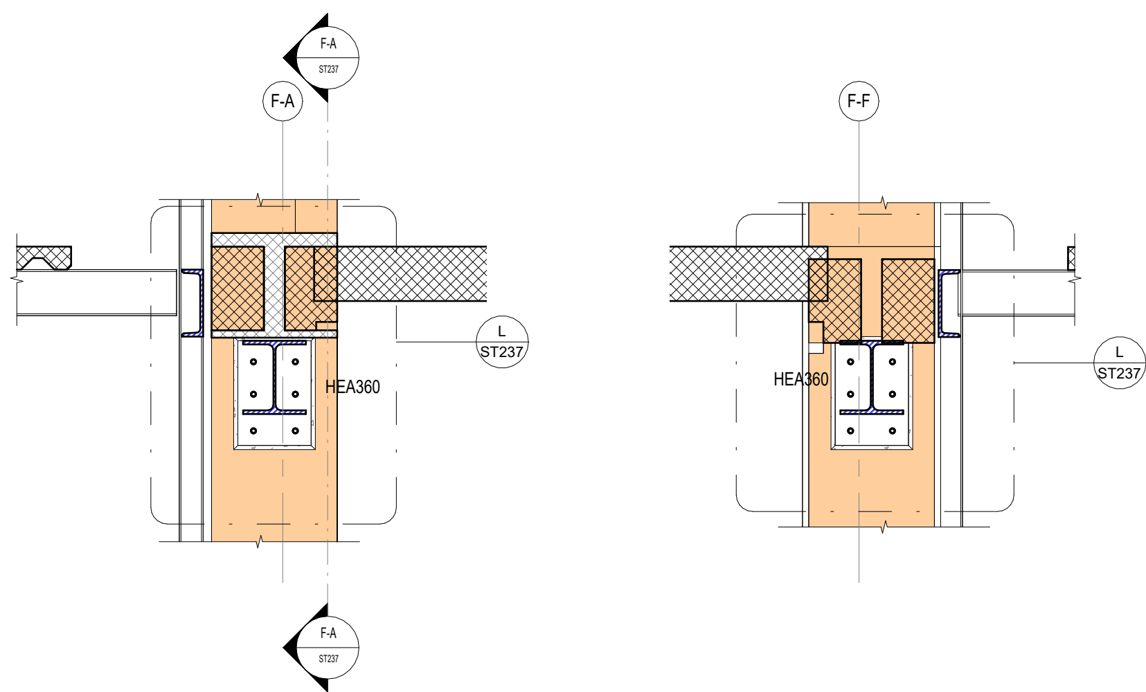
STRUTTURE - GALLERIA - RINFORZO TRAVI ESISTENTE - Sezione G-G 1: 25
