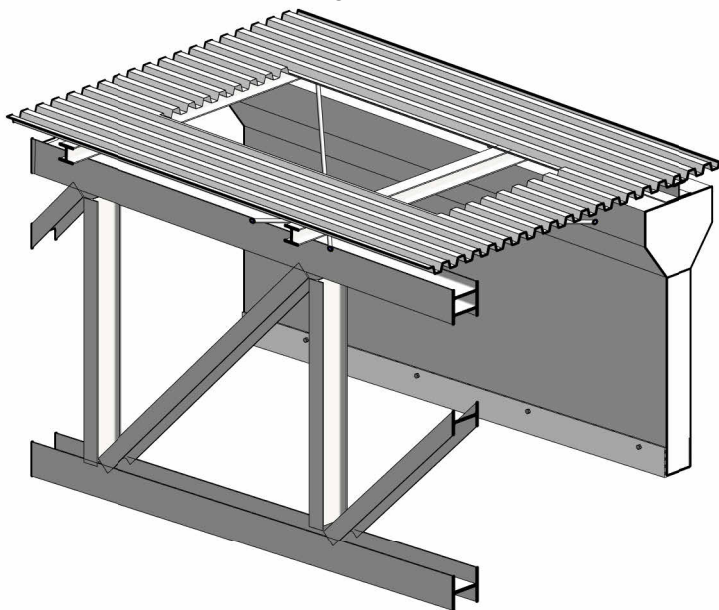
Vista 3D - Foro nella lamiera grecata
