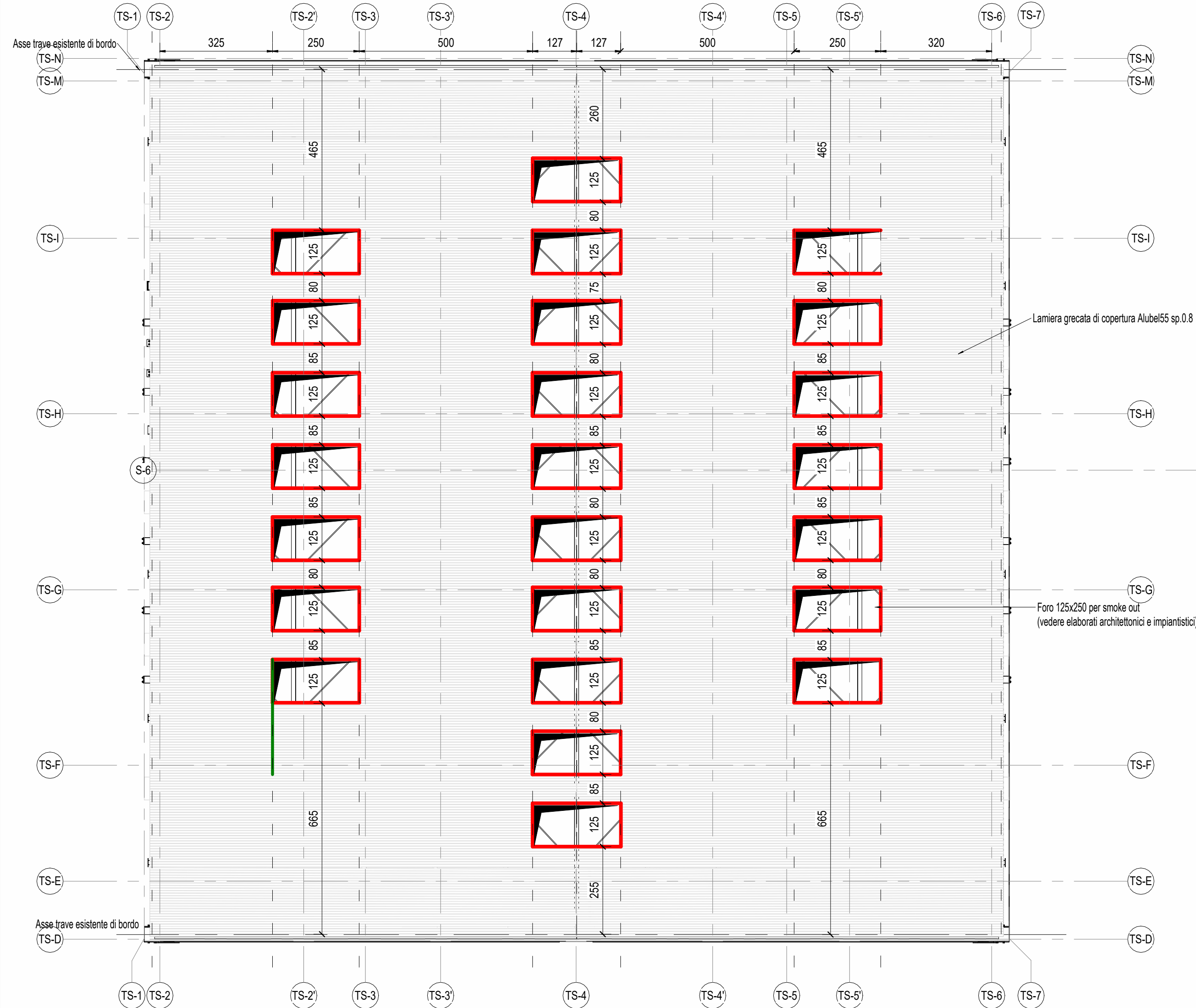
Torre Scenica - Pianta di copertura dall'alto verso il basso 1 : 100
