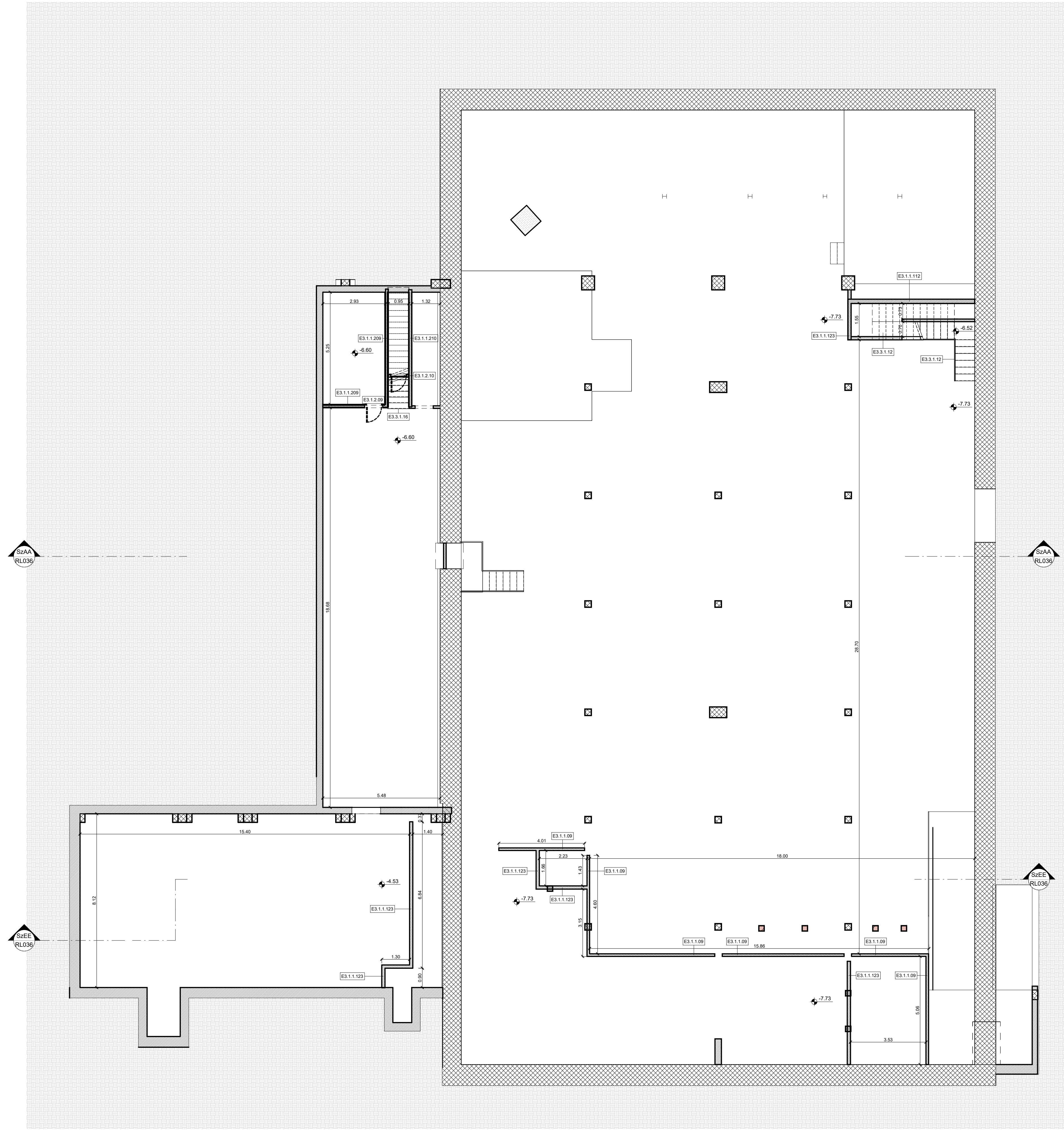
3 Pianta Secondo Interrato Scala 1 : 100
