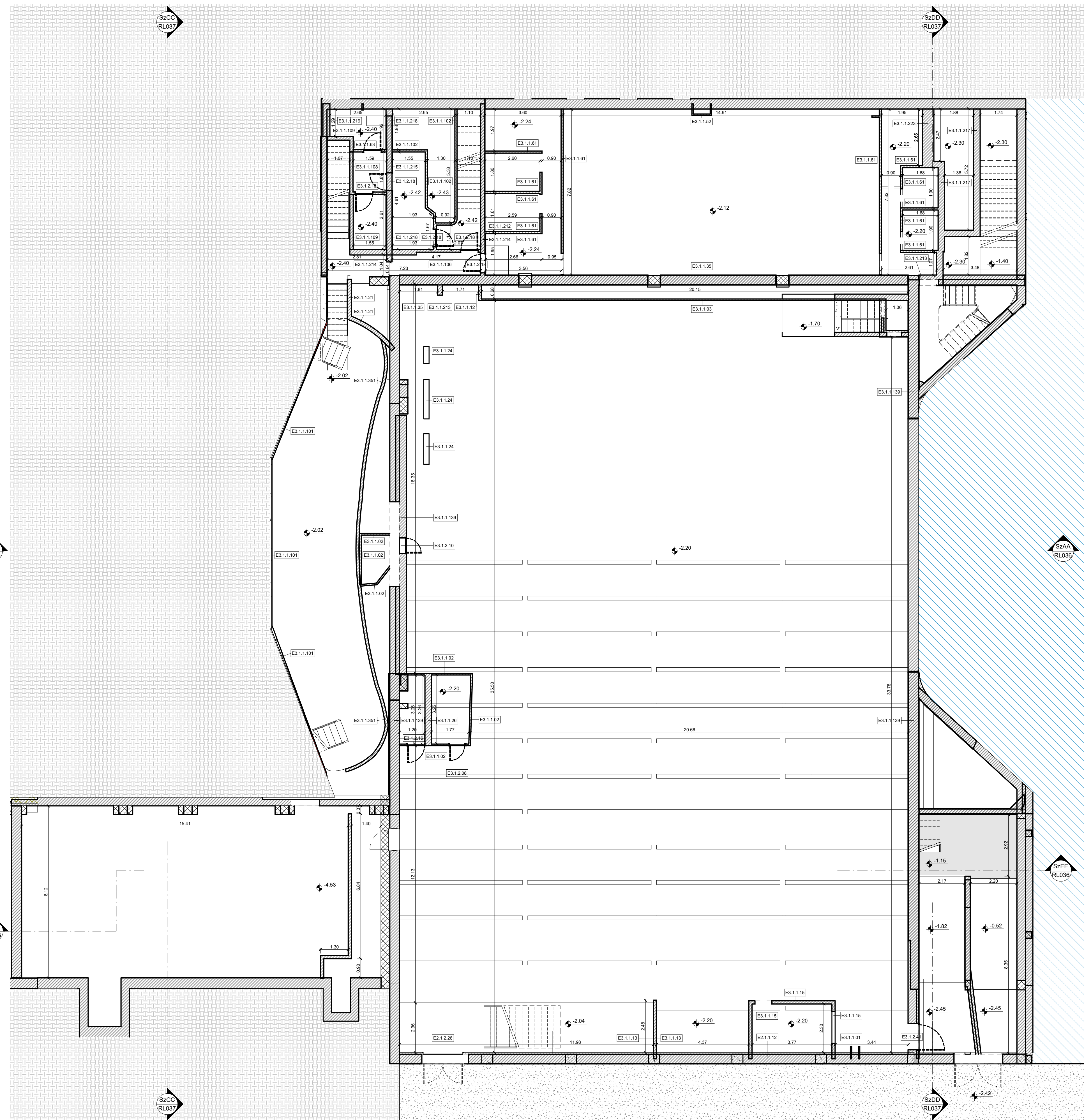
1 Pianta Primo Interrato Scala 1 : 100
