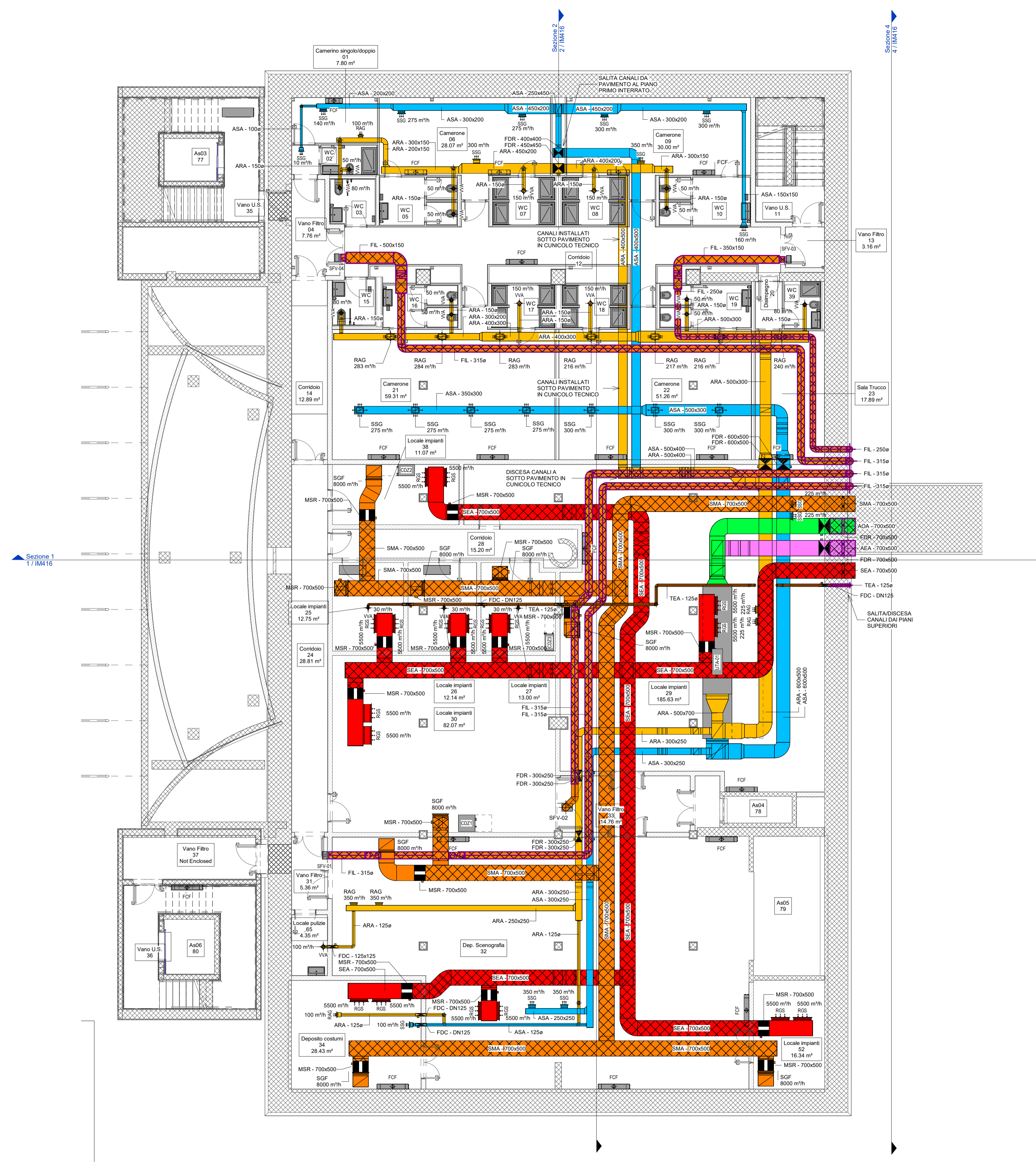
1 1:100 Pianta piano interrato -2
