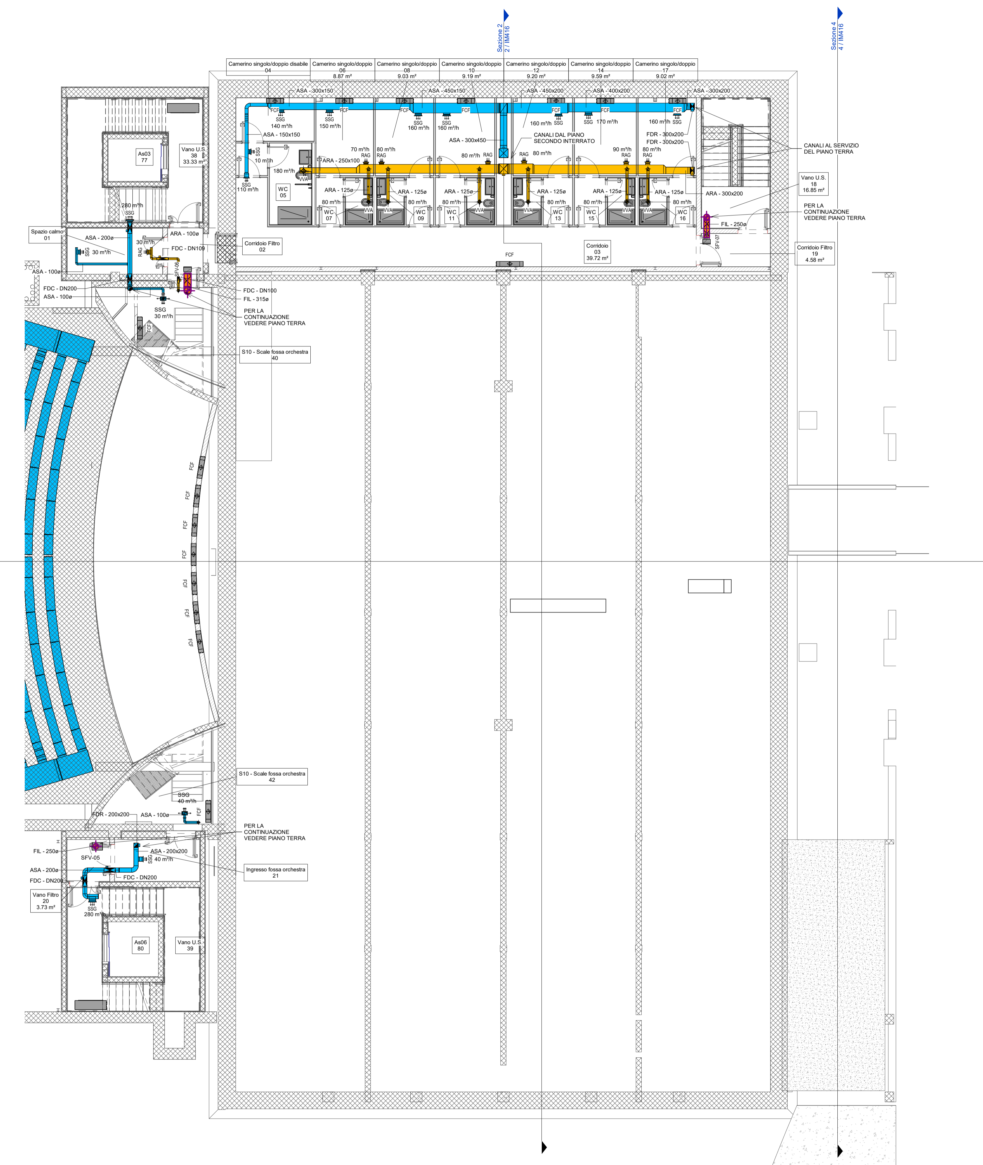
2 1:100 Pianta piano interrato -1
