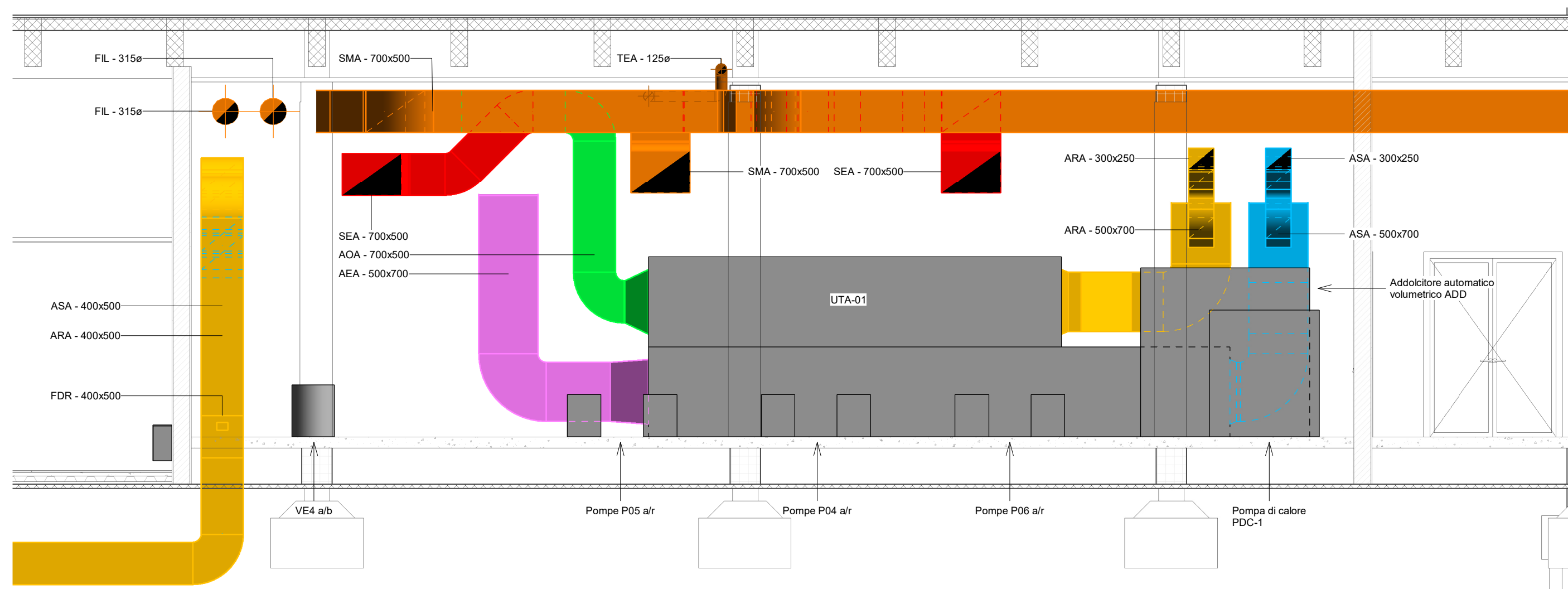
4 CLI Section_1 1:50
