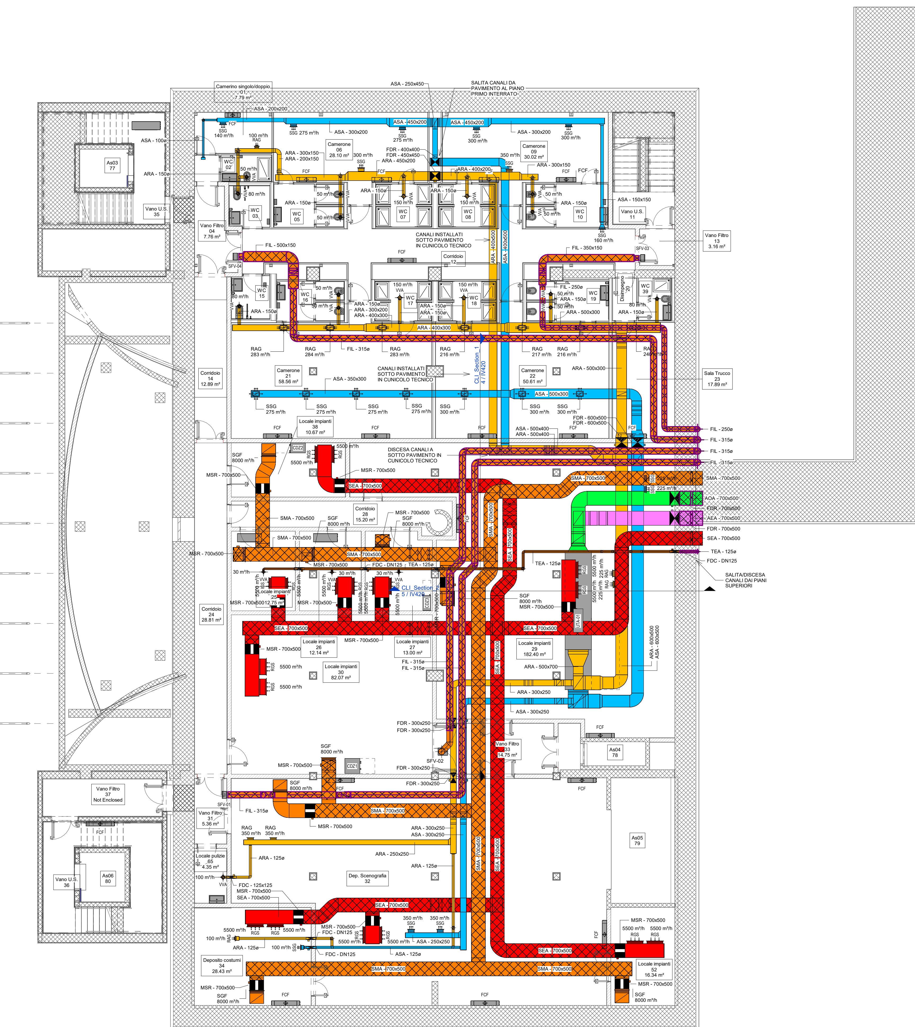
1 Pianta piano interrato -2 1:100
