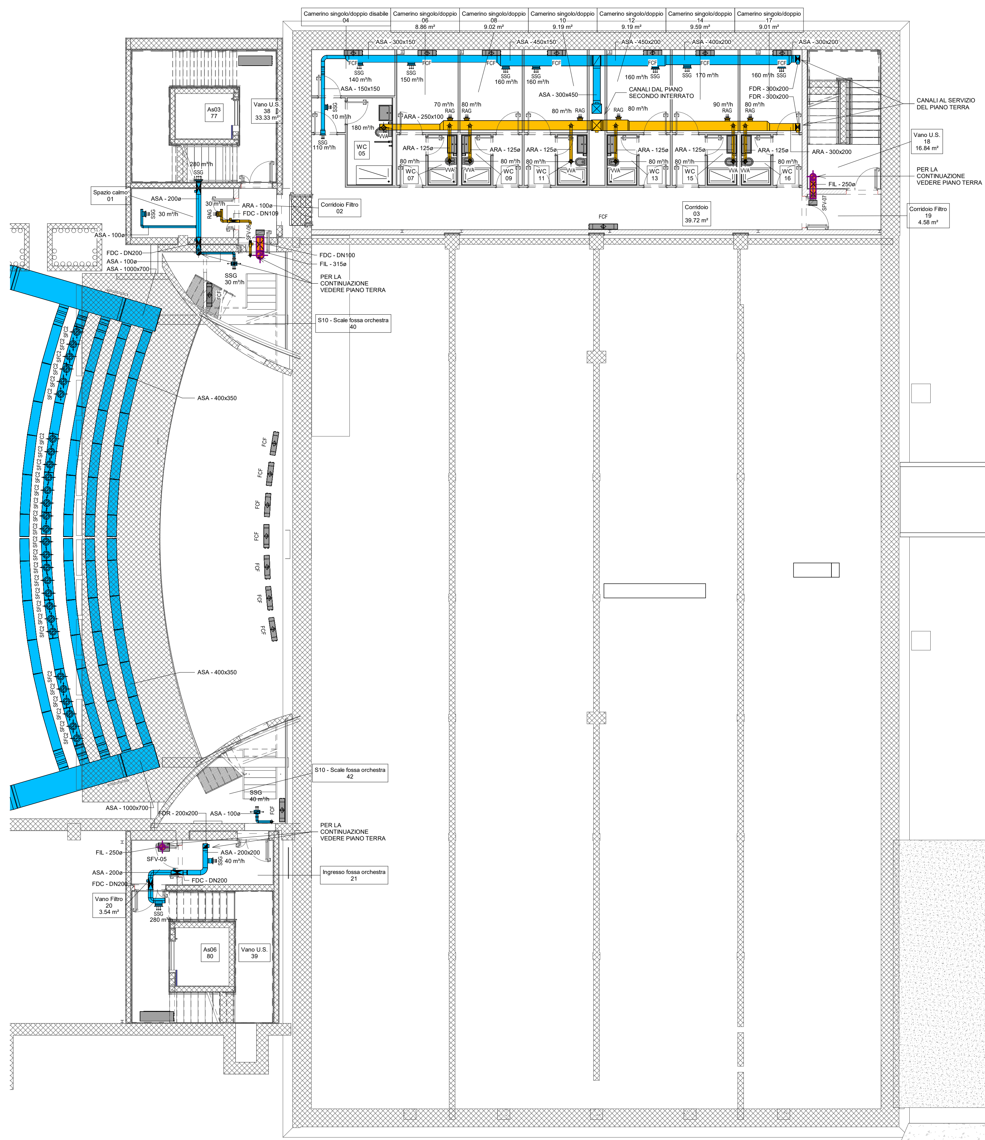
2 Pianta piano interrato -1 1:100
