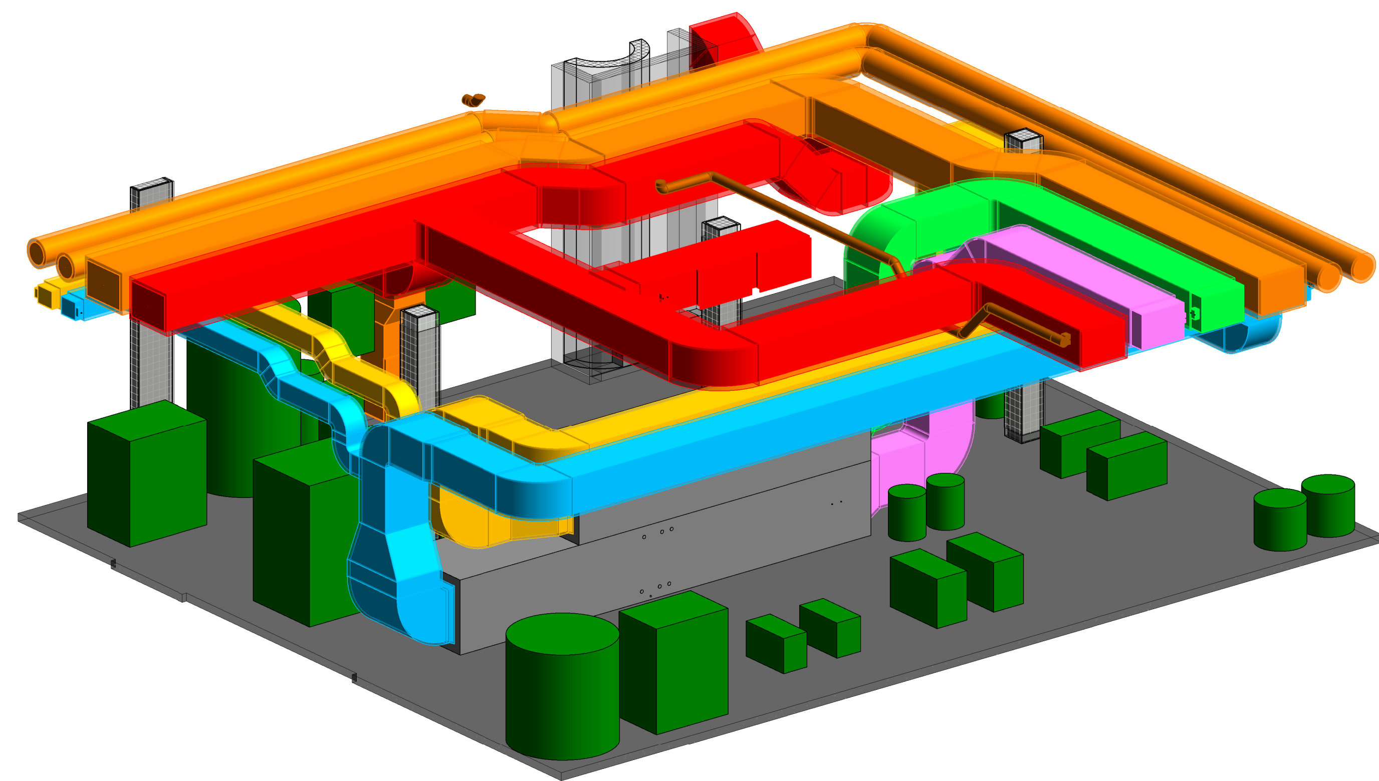
3 PARTICOLARE 3D - CENTRALE CANALI AERAILICI
