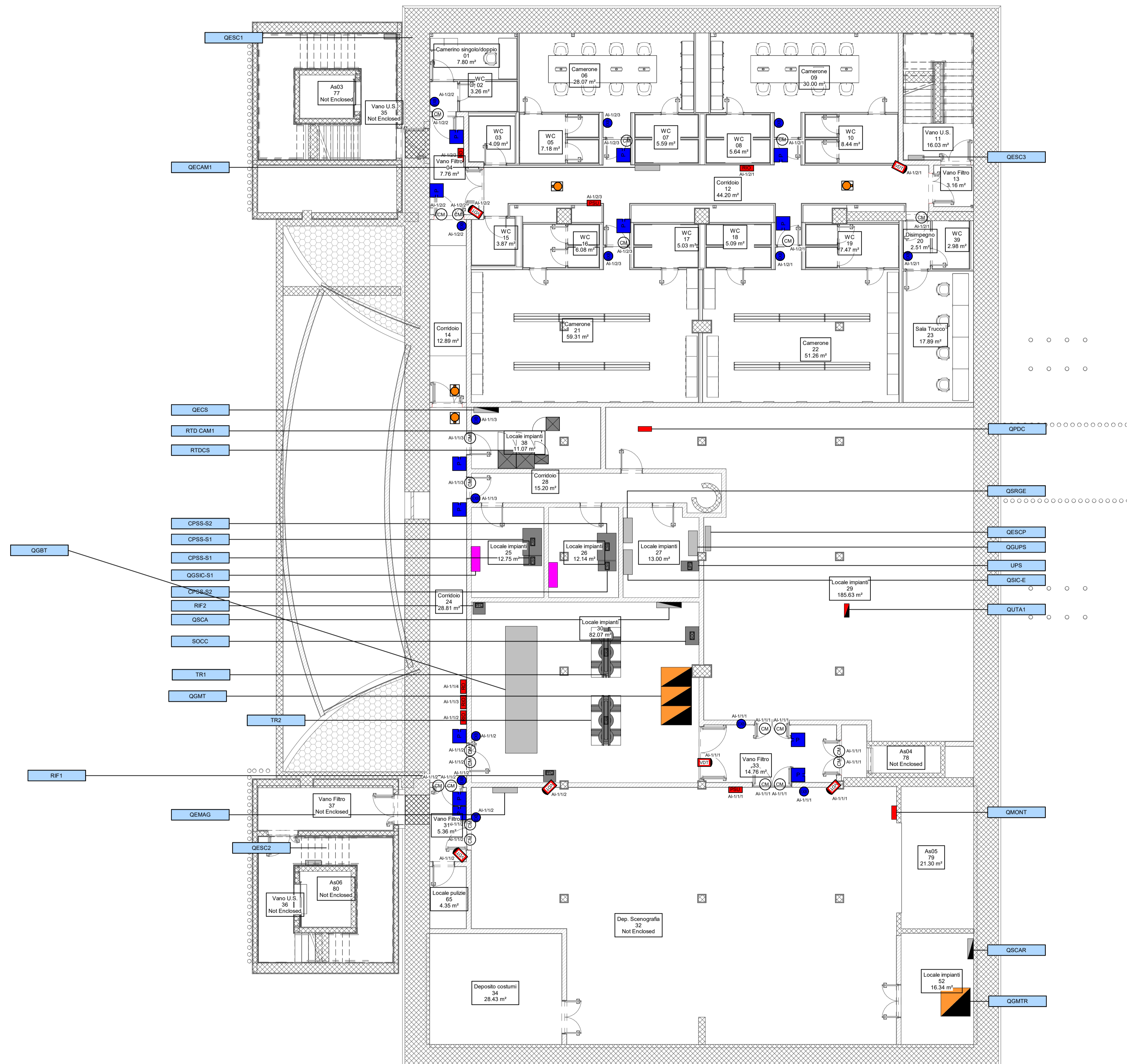
2 Pianta interrato -2 1:100
