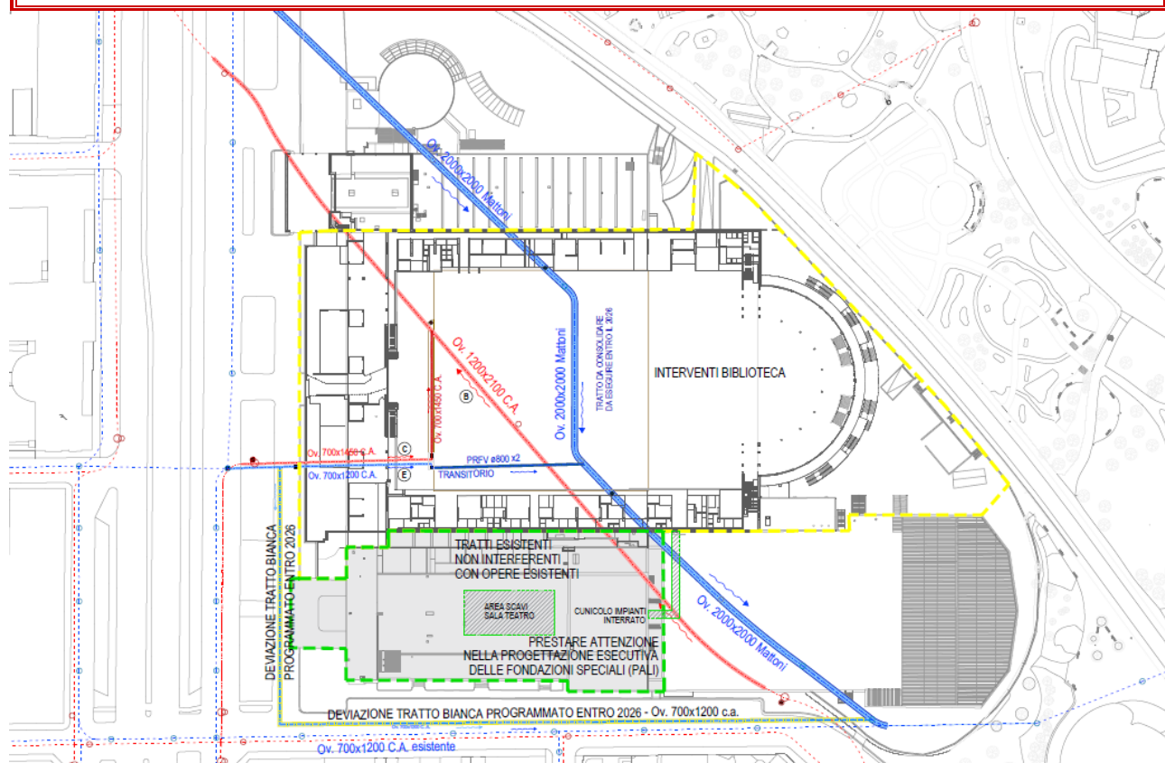
Figura 4 – Planimetria rete fognaria principale, modifiche Biblioteca e integrazione perimetro di intervento TNT Tracciato fognatura bianca = colore blu Tracciato fognatura nera = colore rosso
