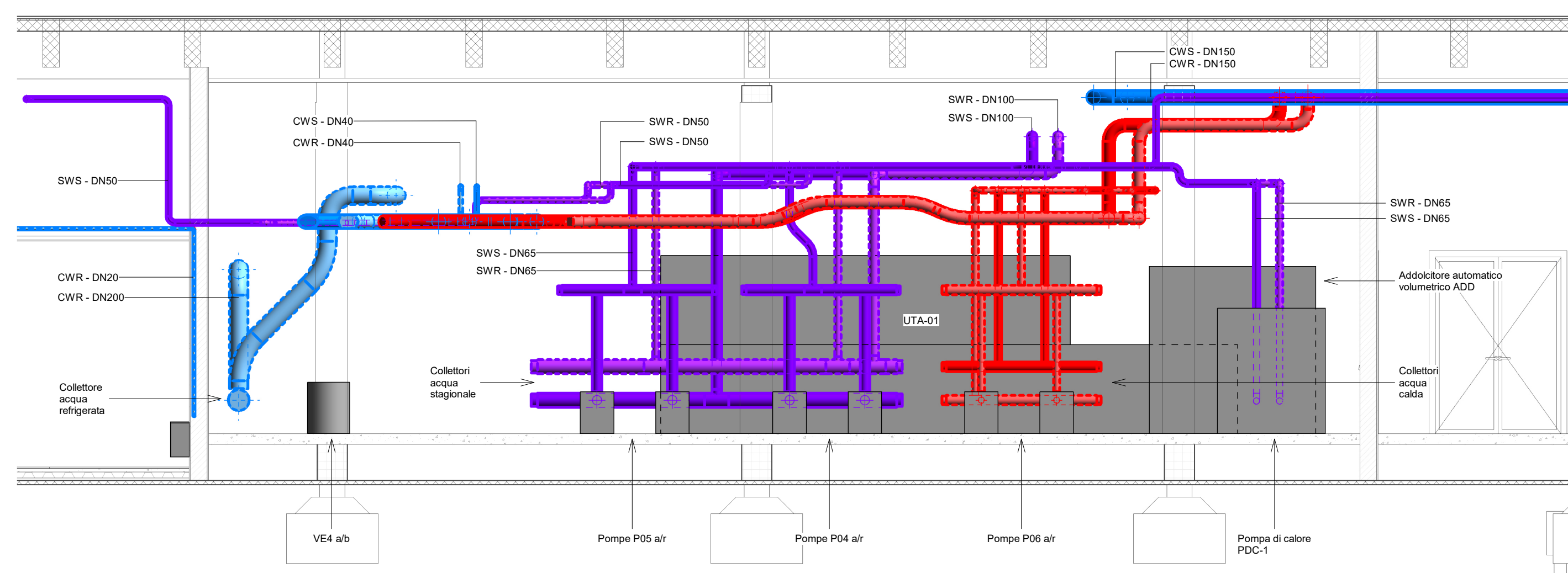
3 HYD_Section_1 1:50
