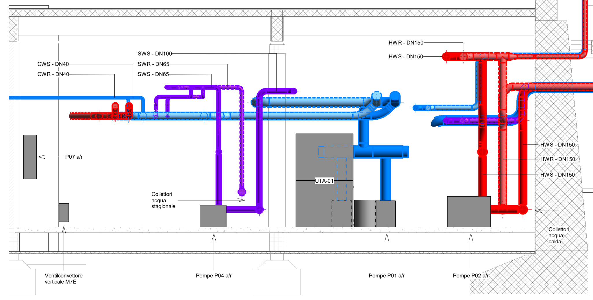
4 HYD_Section_2 1:50
