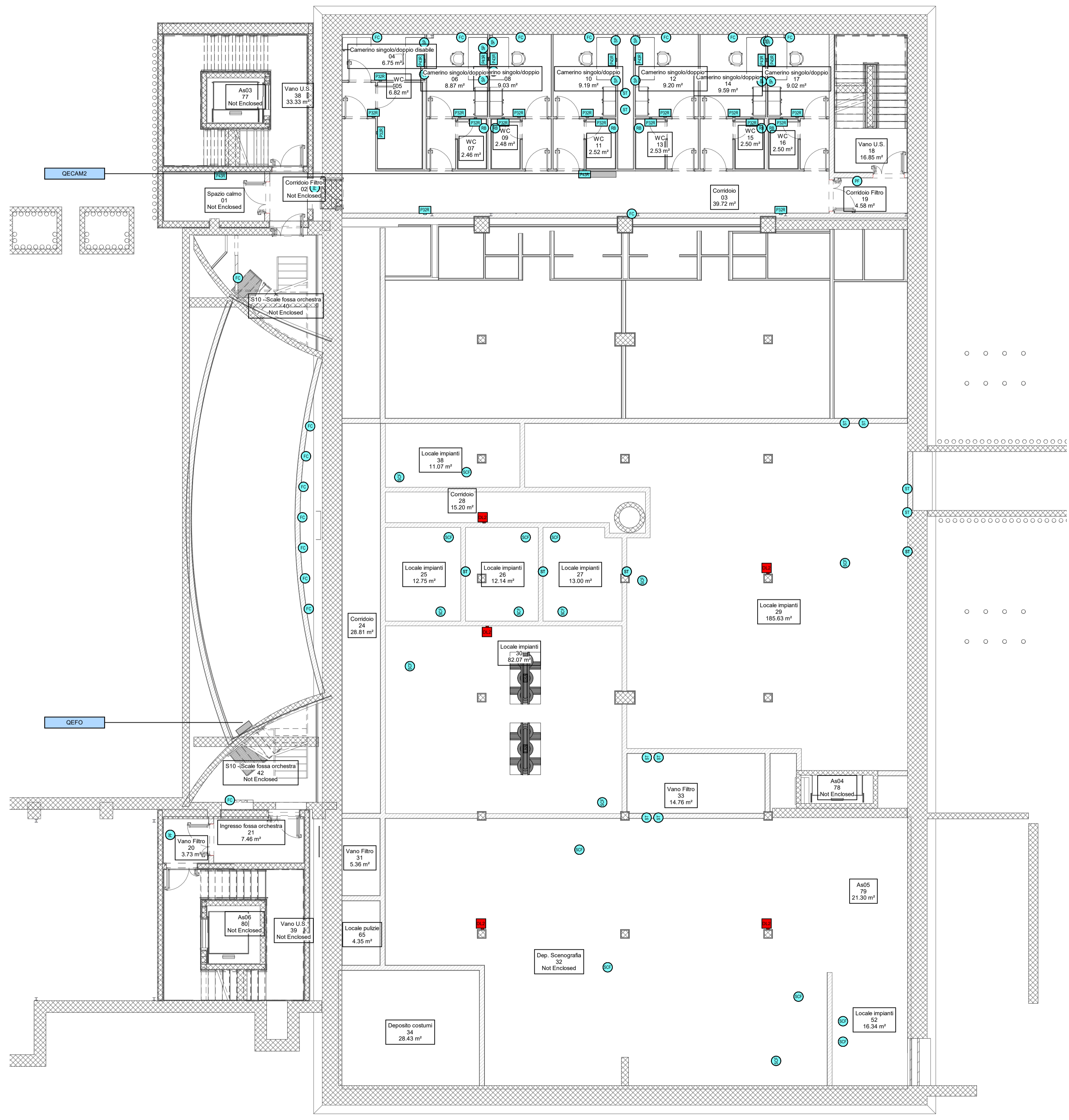
1 Pianta interrato -1 1 : 100
