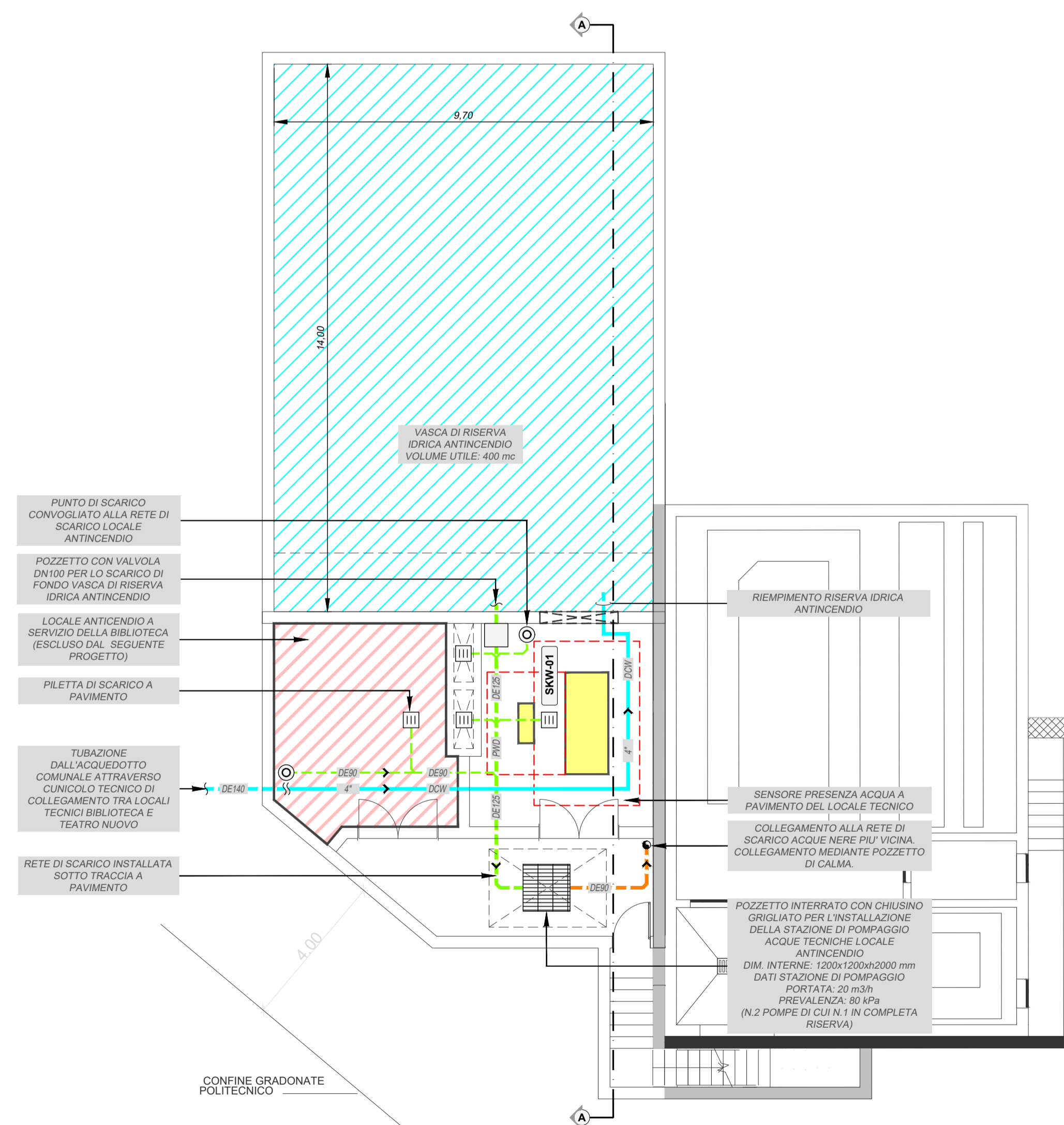
PARTICOLARE SISTEMA DI SCARICO E ADDUZIONE VASCA ANTINCENDIO
