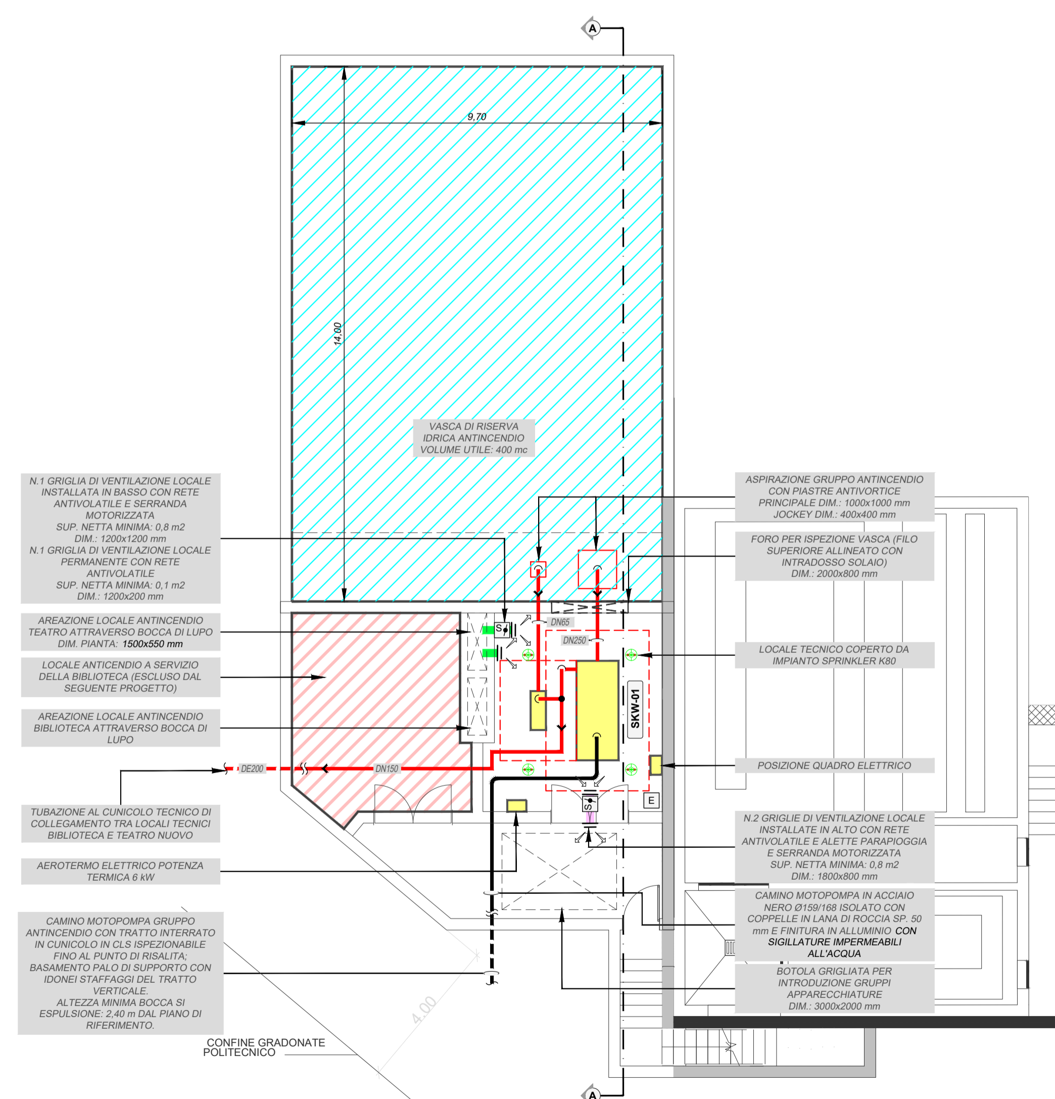
PIANTA LOCALE ANTINCENDIO
