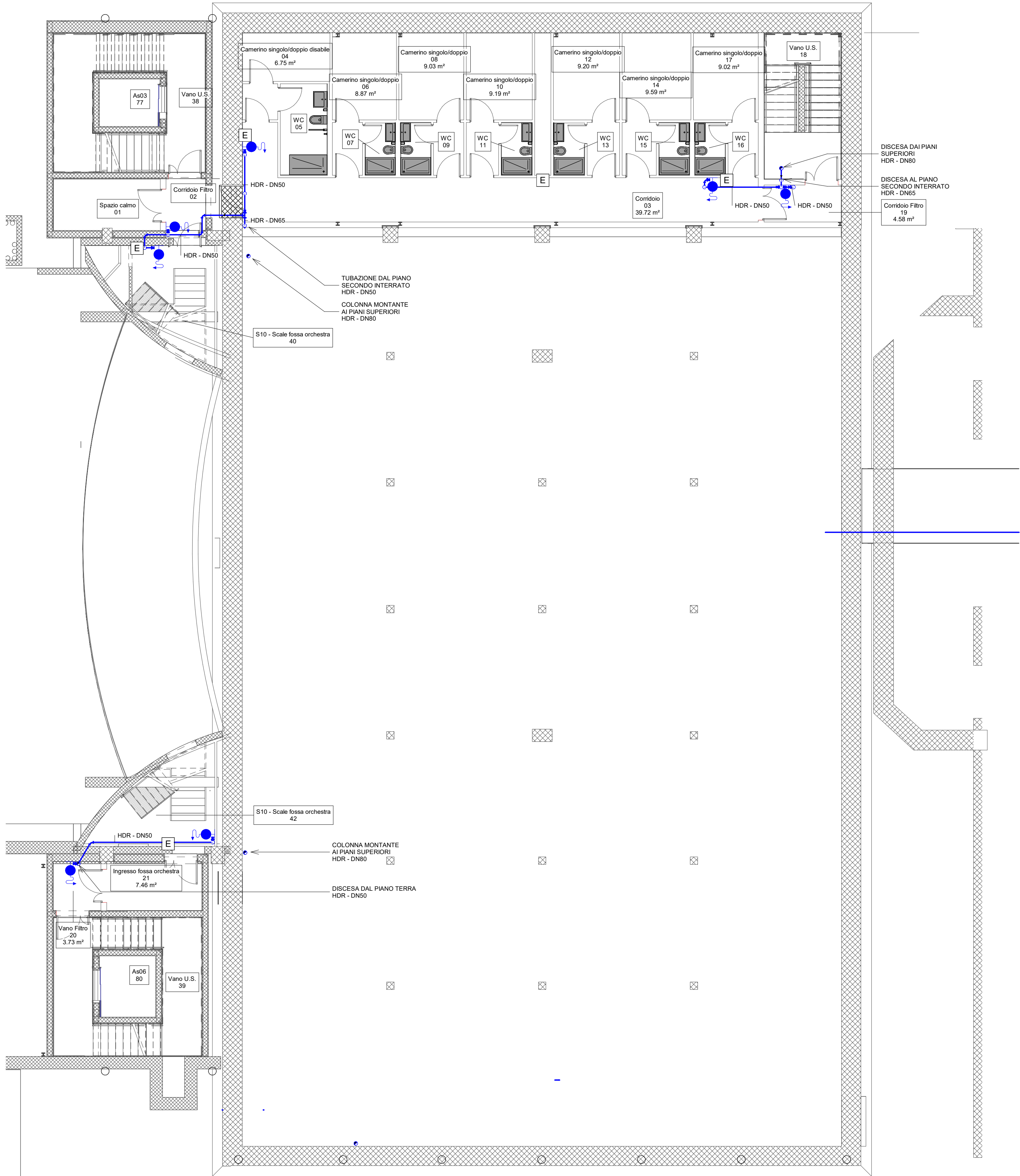
2 Pianta piano interrato -1 1 : 100
