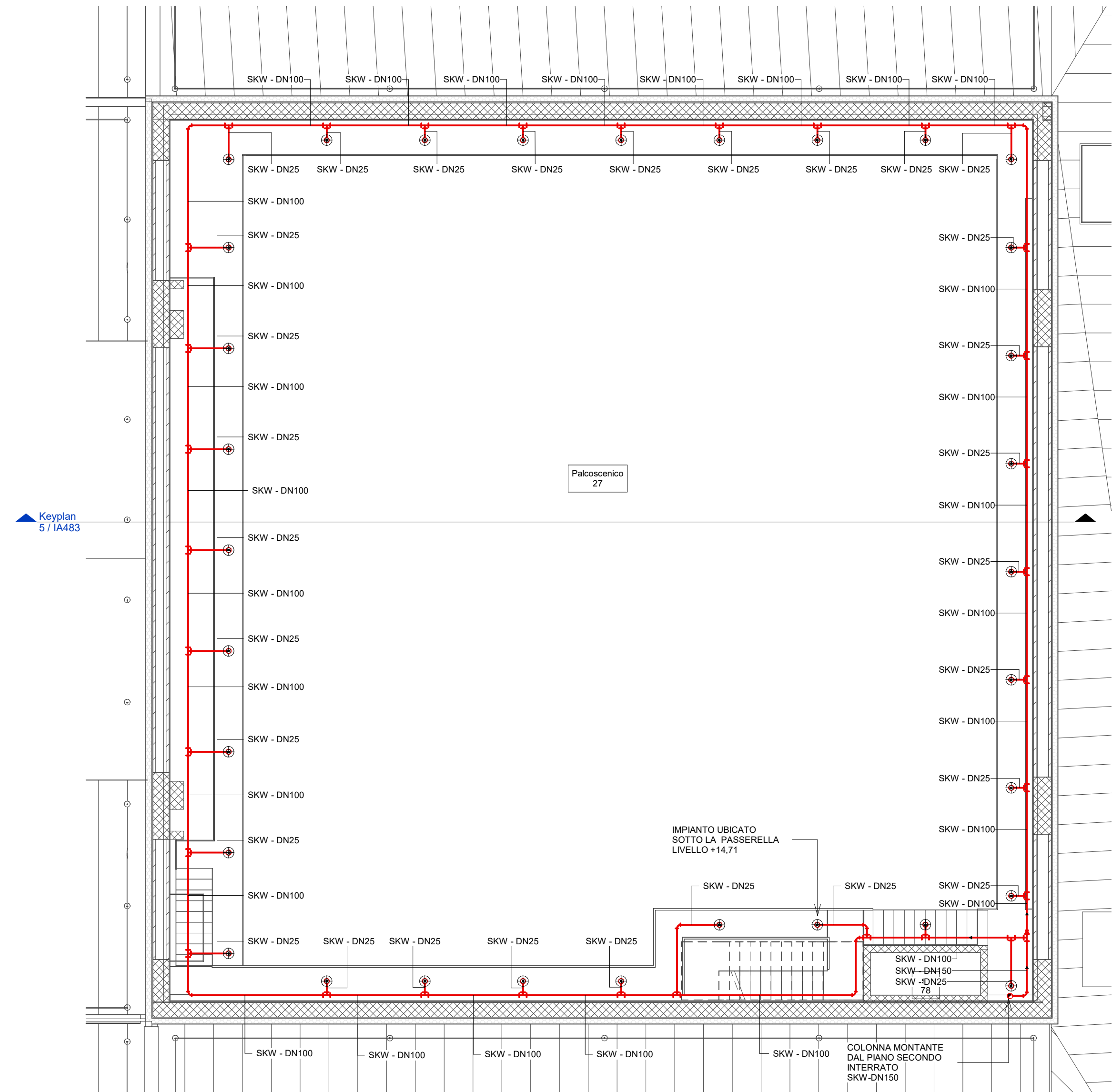
1 Livello Passerella +14.71 1 : 100
