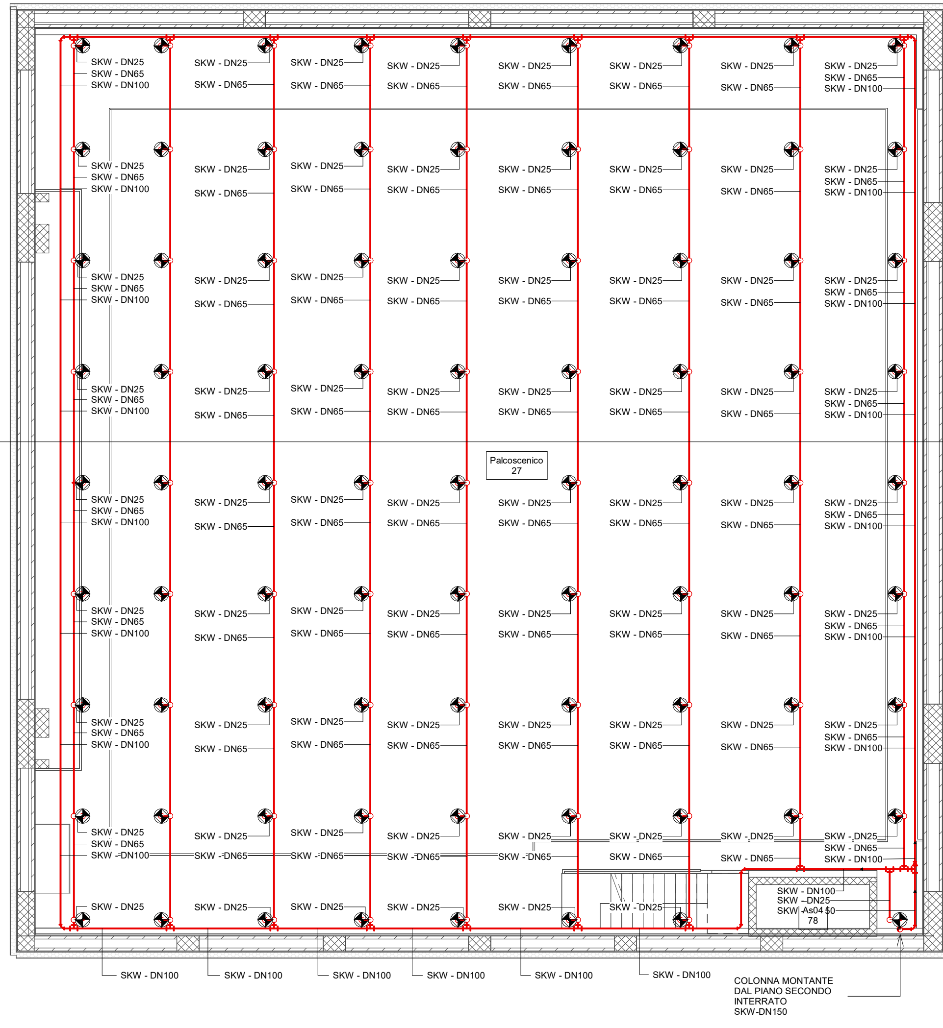
3 Piano Torre scenica sotto graticcio 1 : 100
