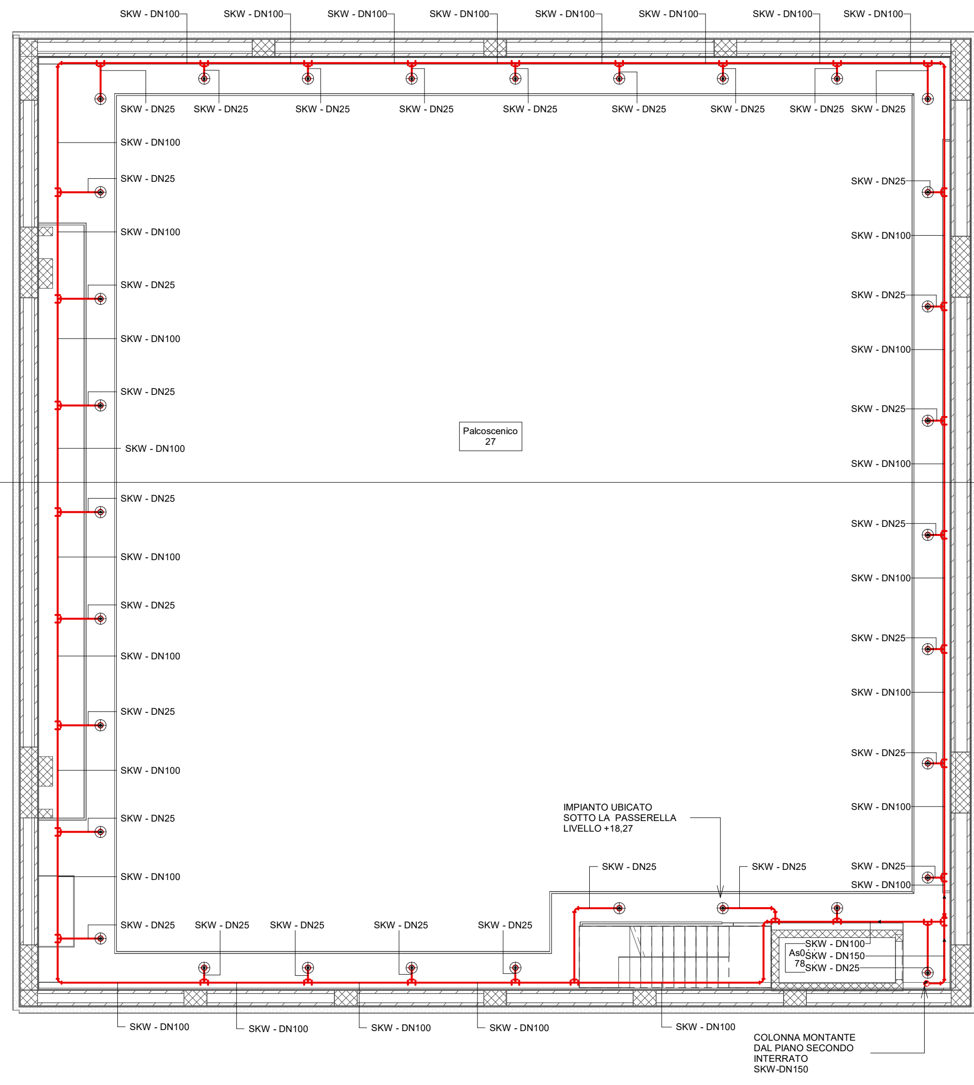
2 Livello Passerella +18.27 1 : 100
