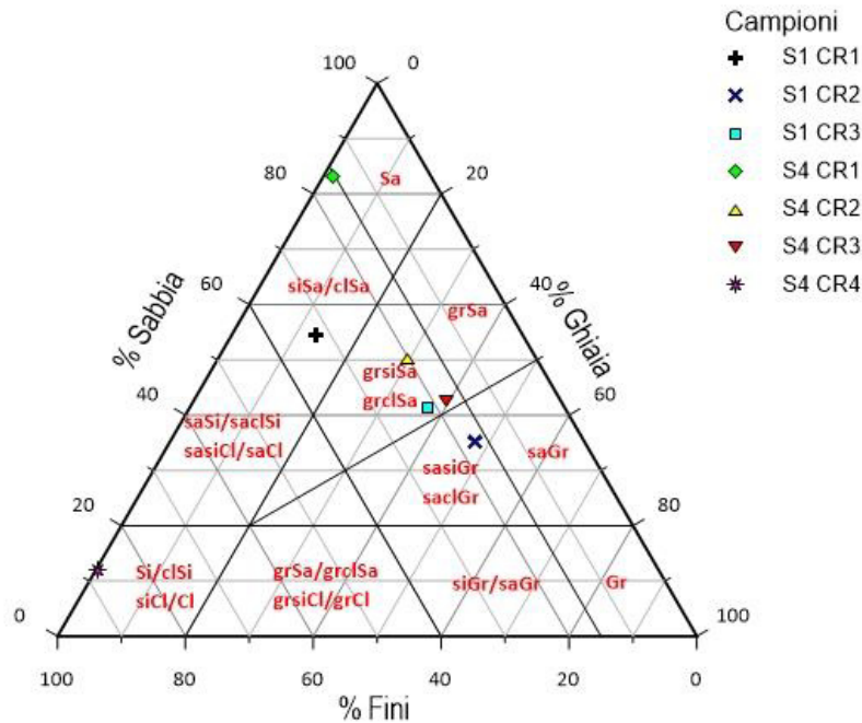
Figura 3-5 – Composizione granulometrica (UNI EN 14688-2)
