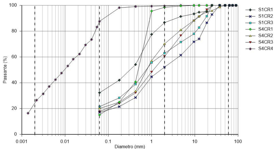
Figura 3-4 – Curva granulometrica
