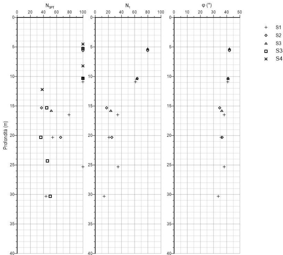
Figura 3-2 – Risultati ed elaborazione dati delle prove SPT
