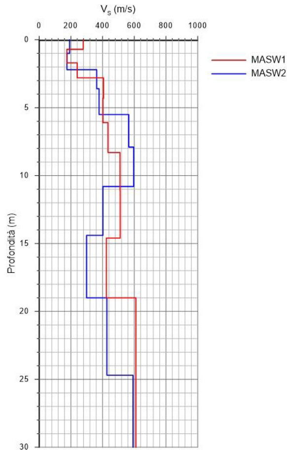
Figura 3-3 – Profilo delle velocità delle onde di taglio
