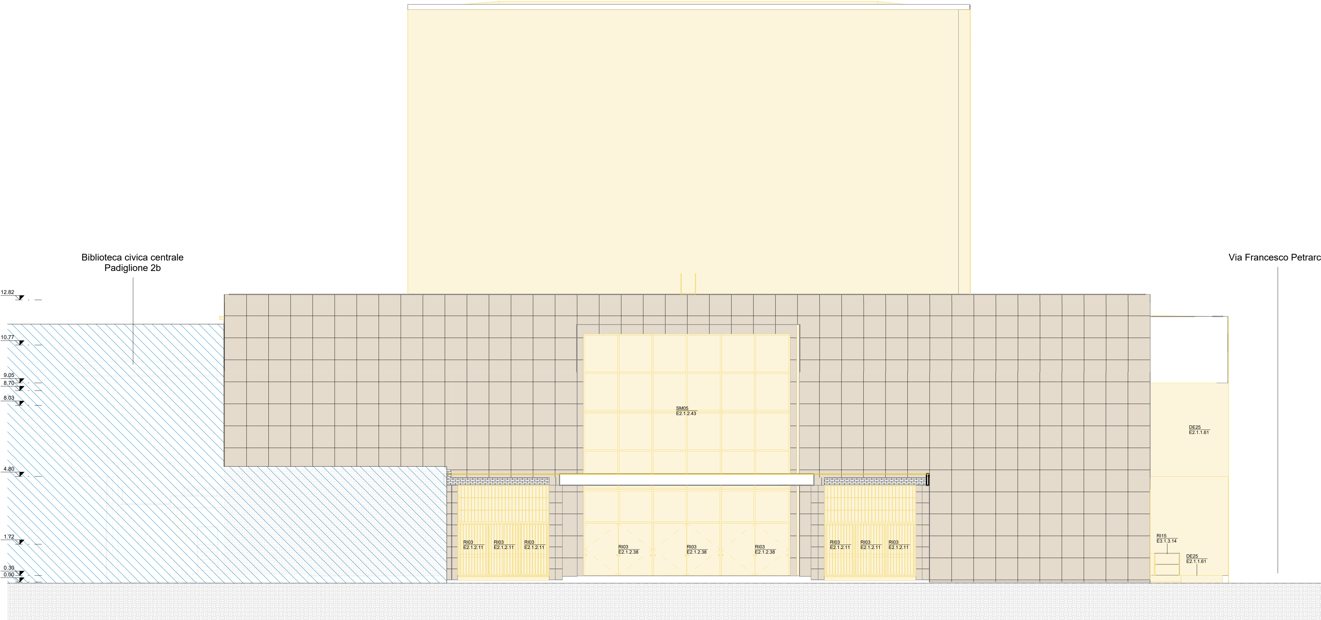
1 Prospetto N-O Scala 1:100
