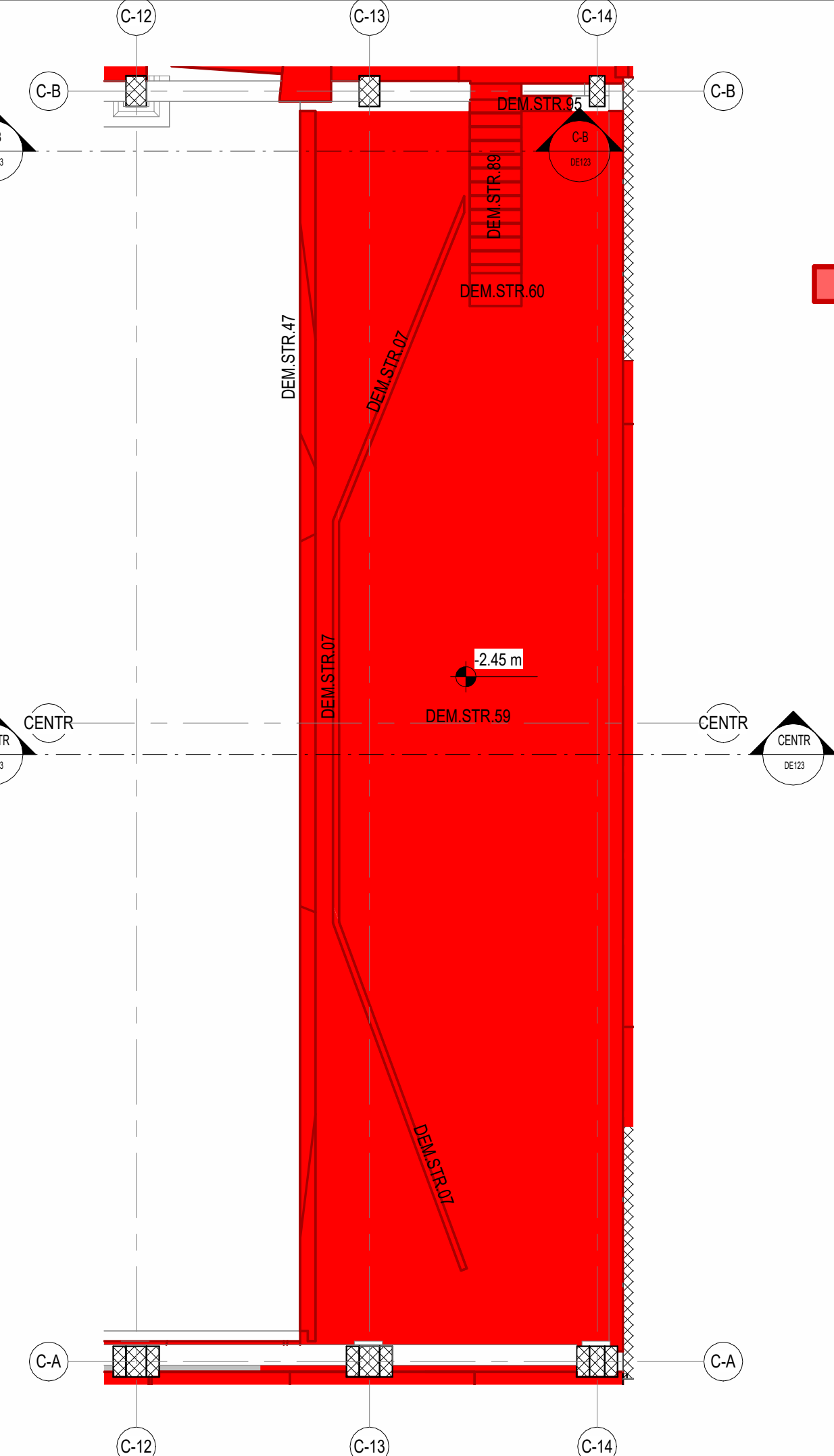
DEMOLIZIONI - FOYER GALLERIA E TEATRO - Pianta fossa orchestra - Vista dall'alto verso il basso
