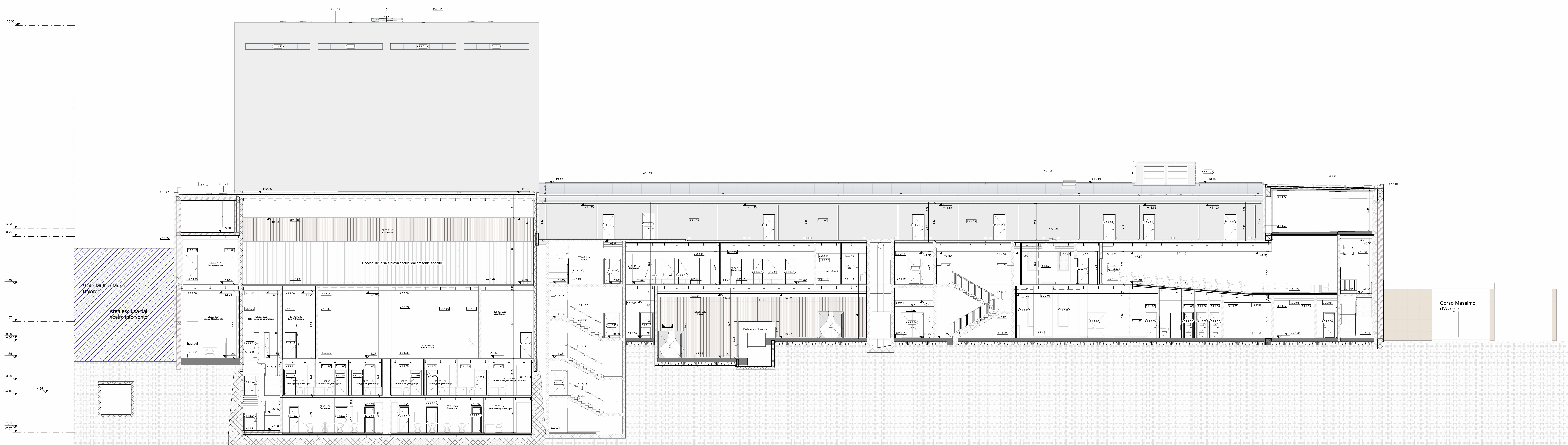
2 Sz B-B Scala 1:100
