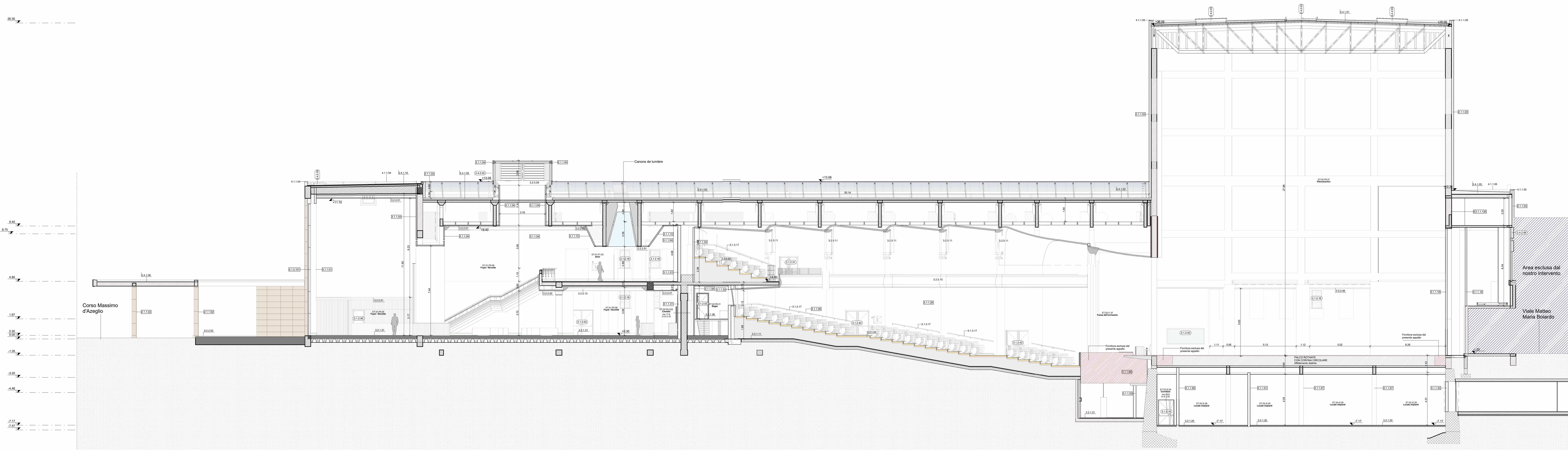
1 Sz A-A Scala 1:100
