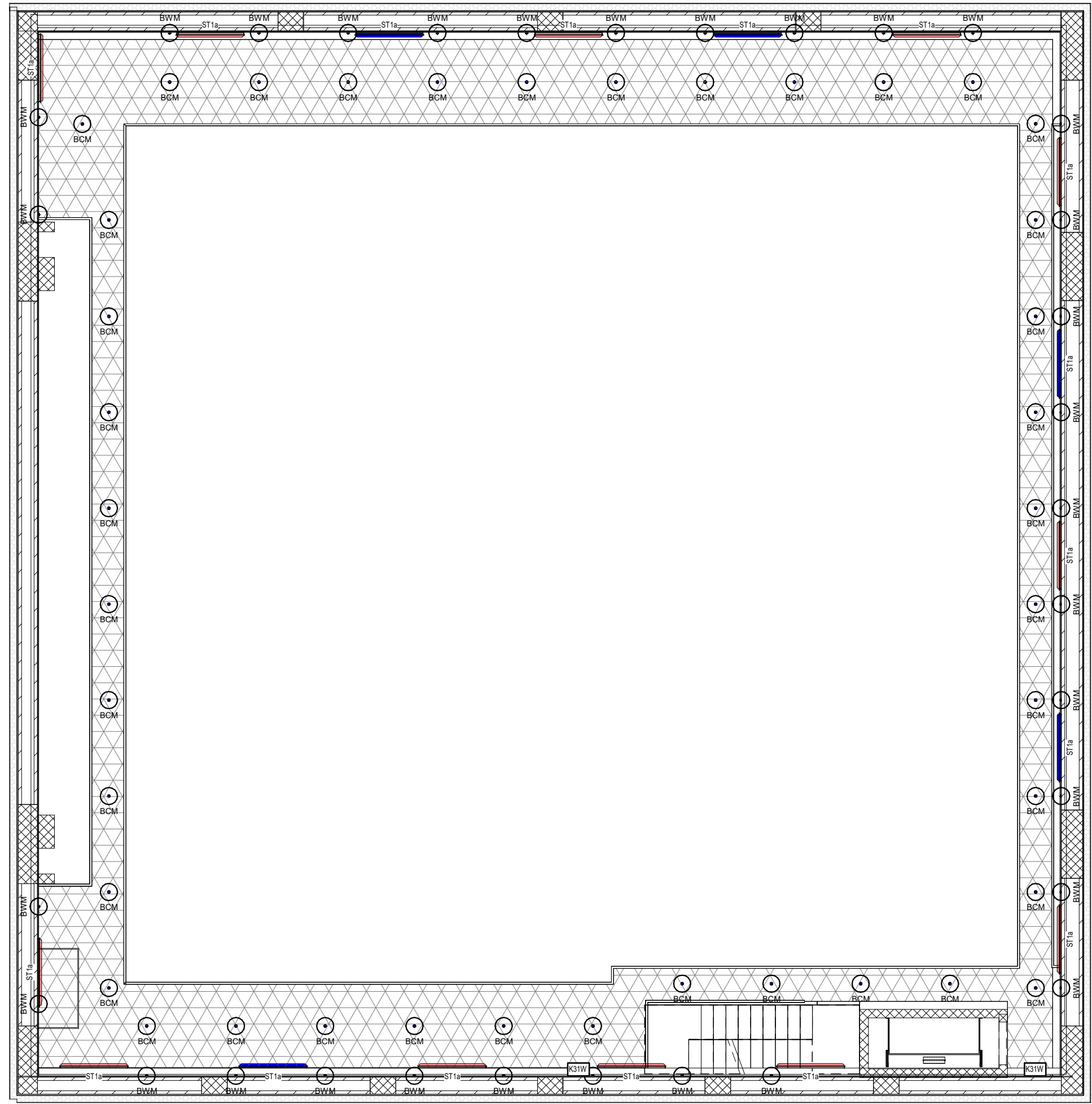
2 Livello Passerella + 18,27 1 : 100
