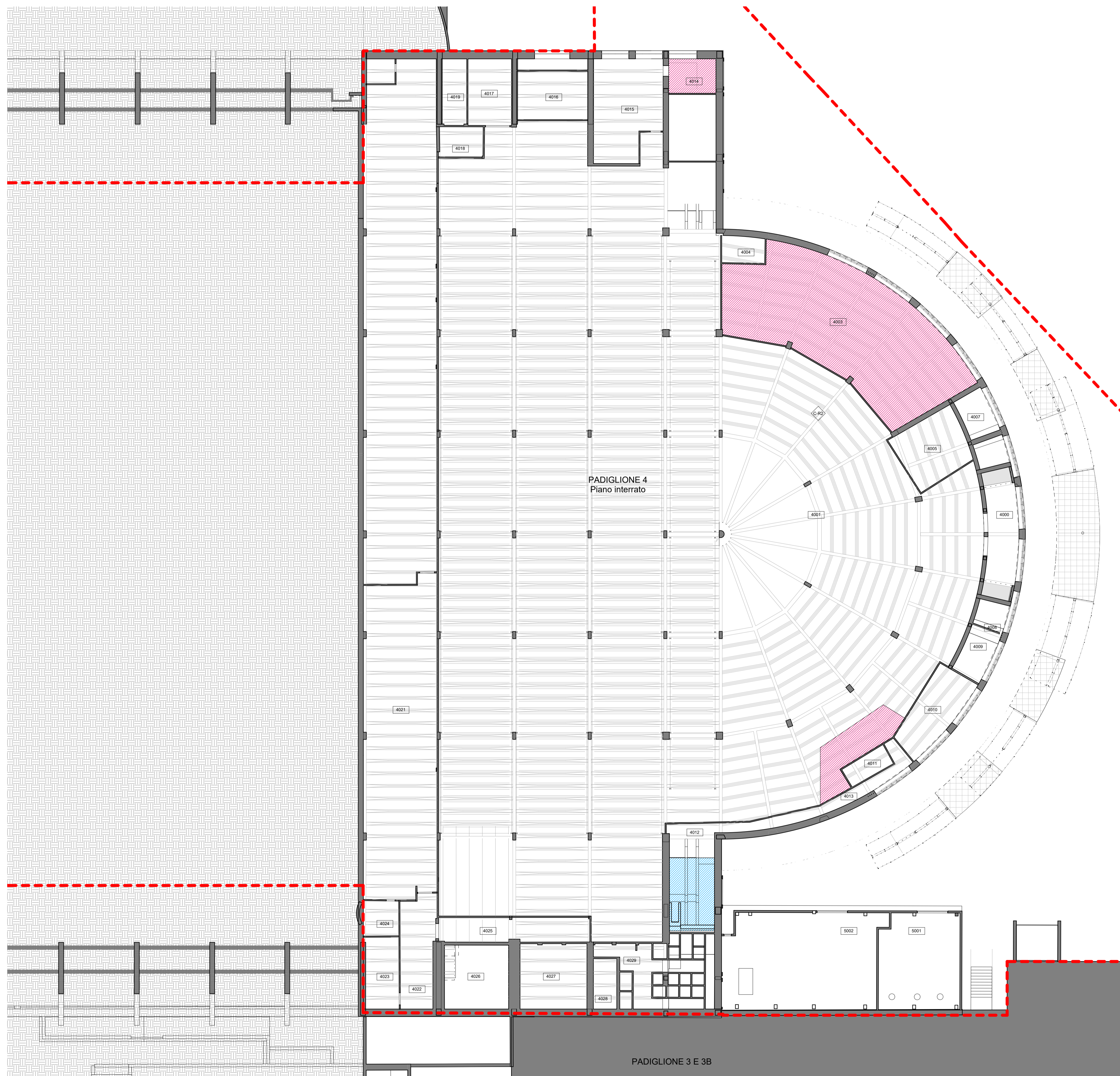
Pianta piano interrato
