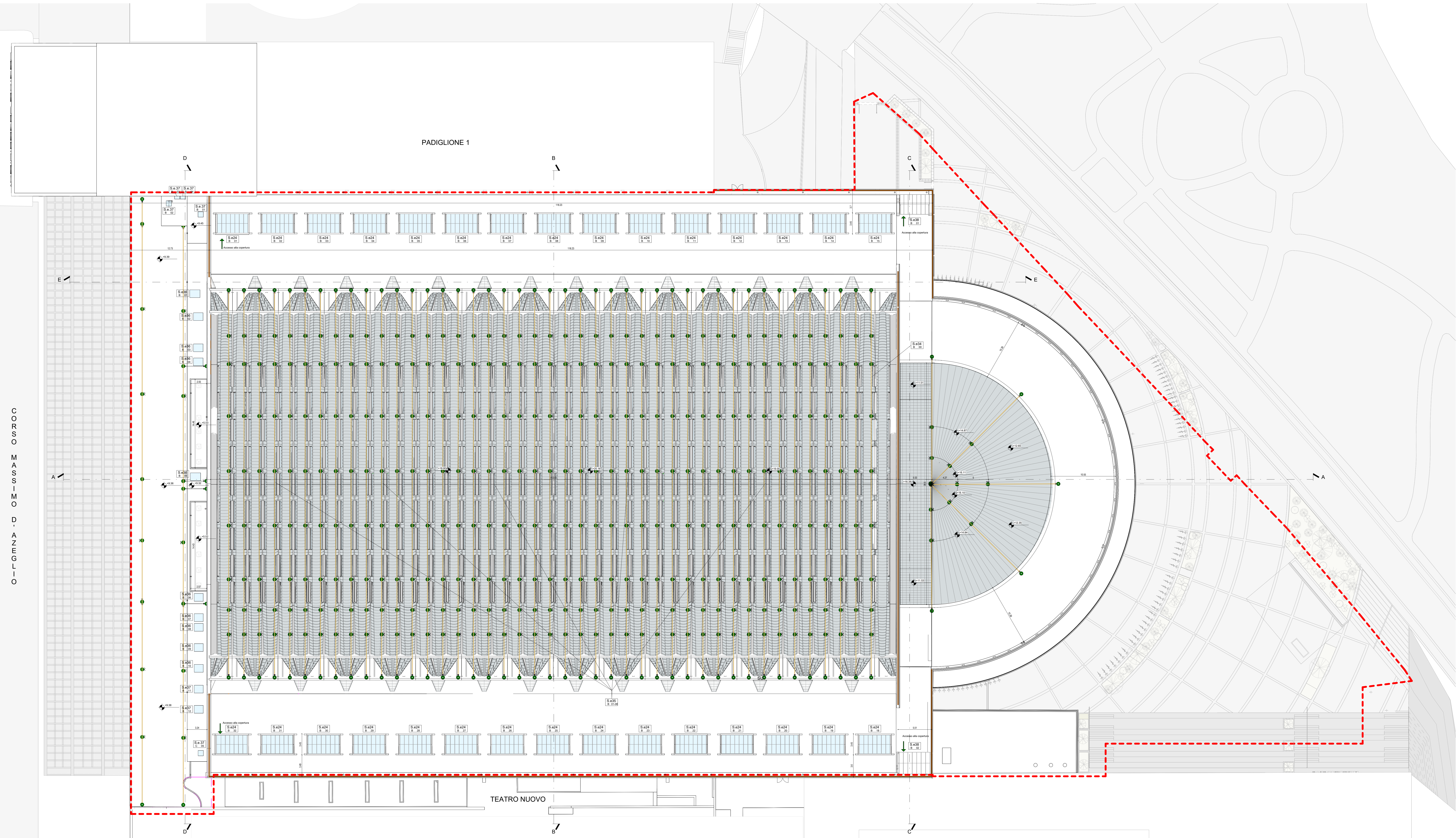
Pianta copertura
