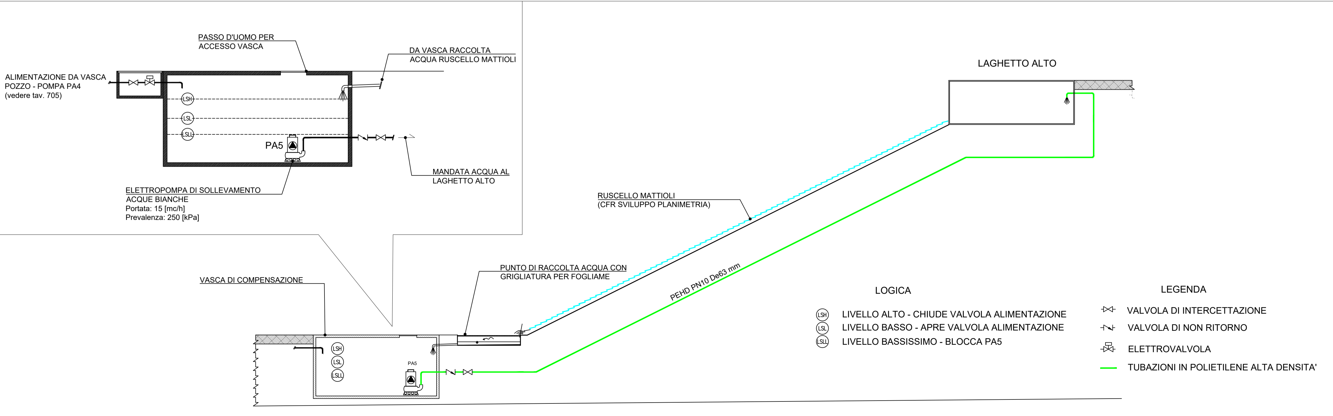
Schema impianto fontana Mattioli
