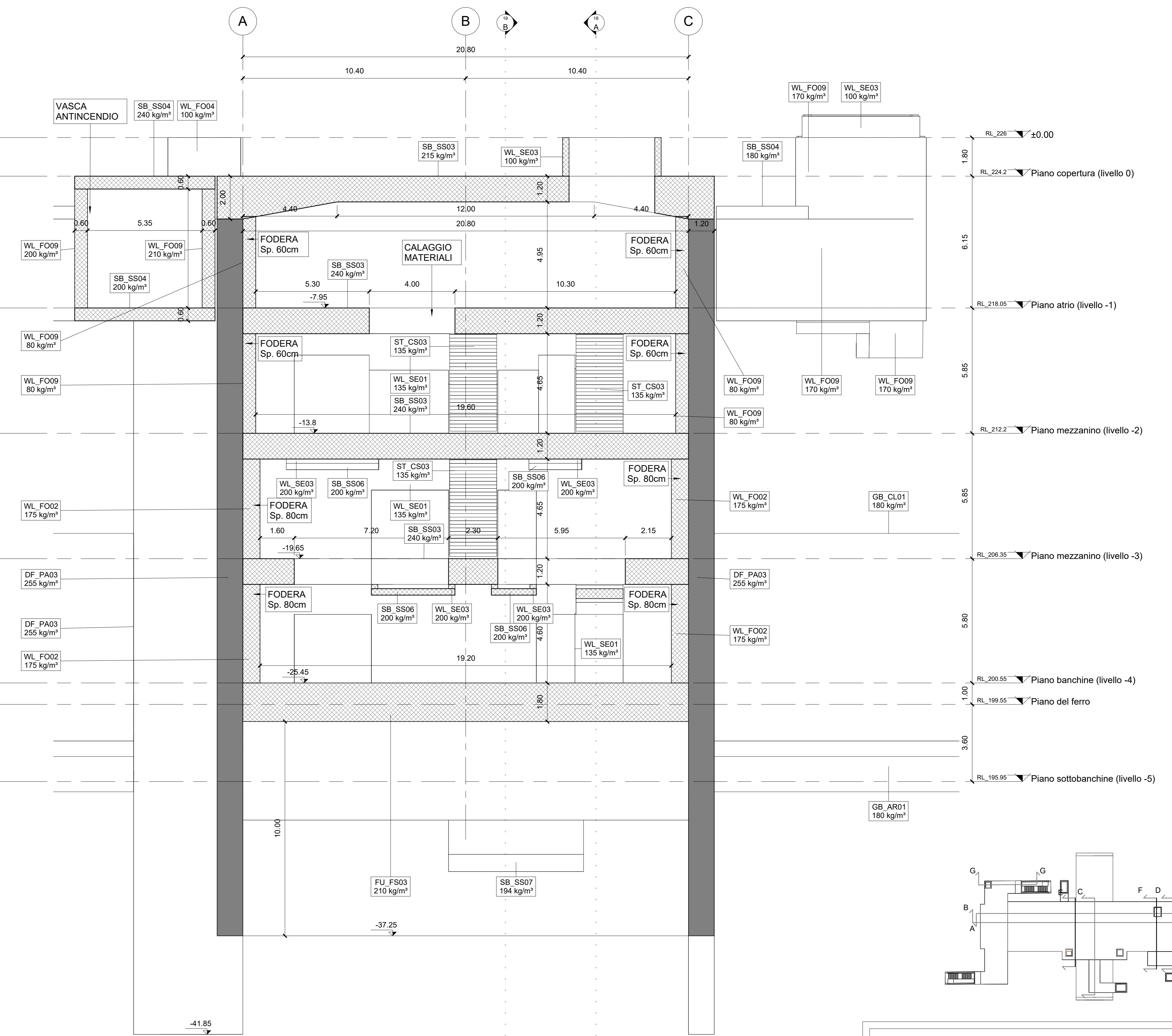
2 SEZIONE F 1:100
