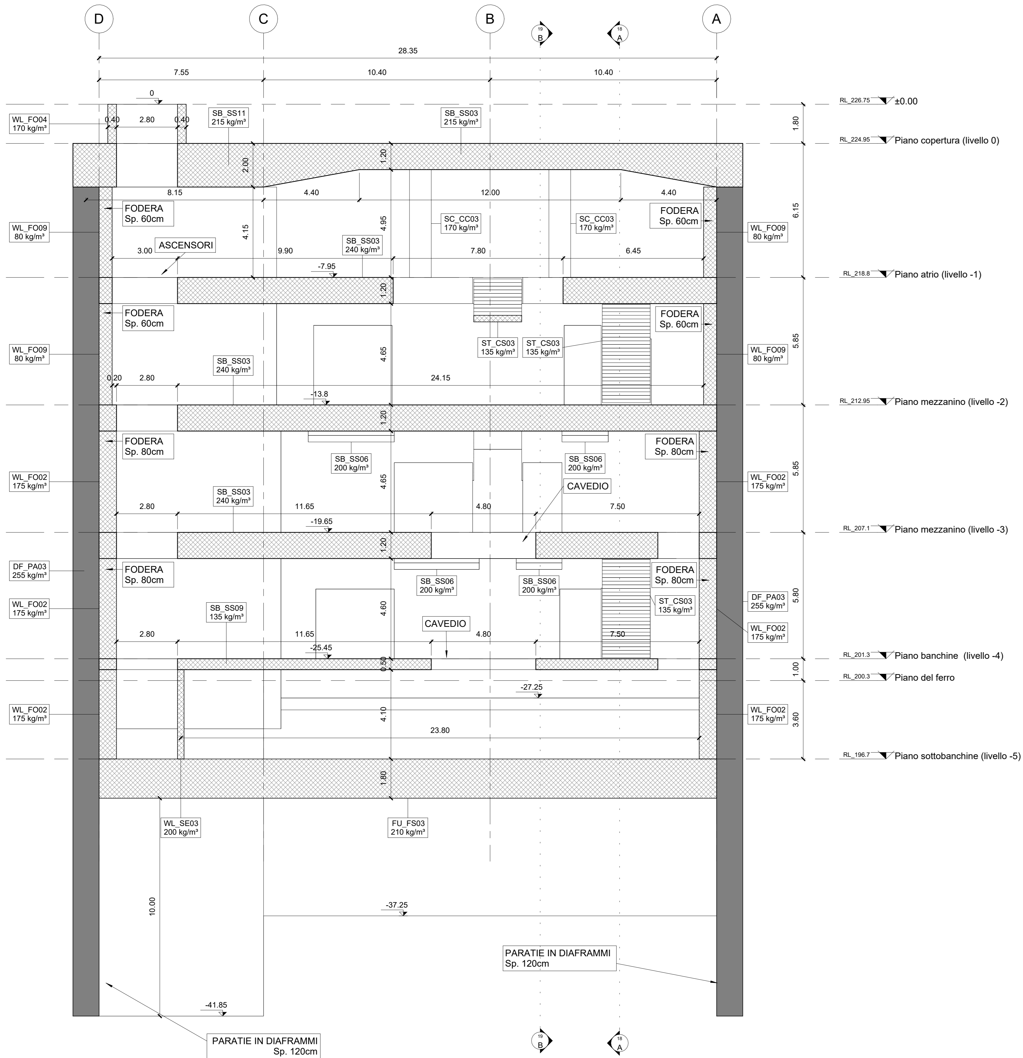
1 SEZIONE E 1:100
