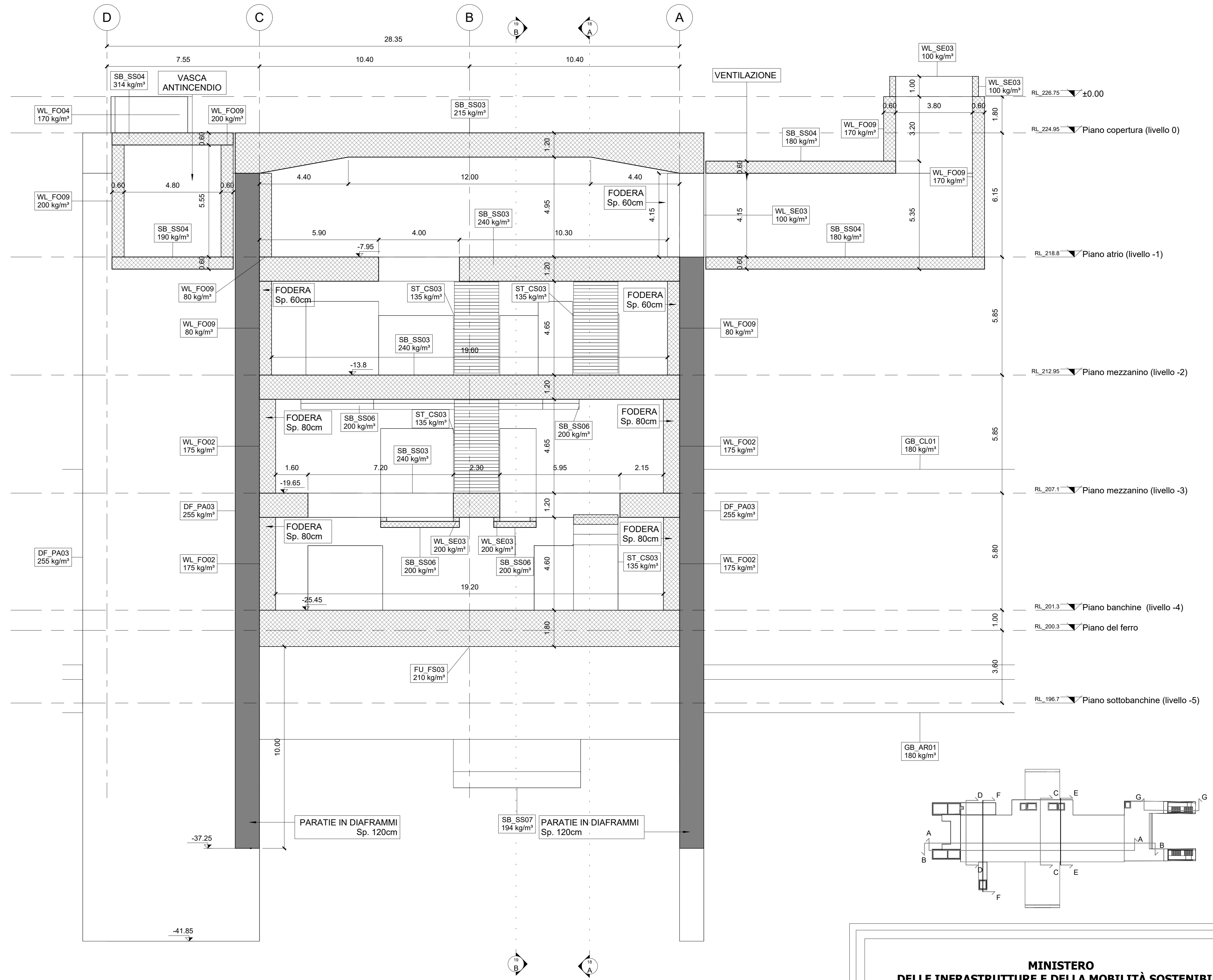
2 SEZIONE F 1:100
