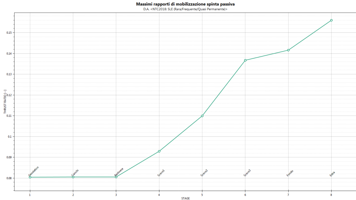
Figura 46. Resistenza passiva mobilitata in condizioni di esercizio (SLE)
