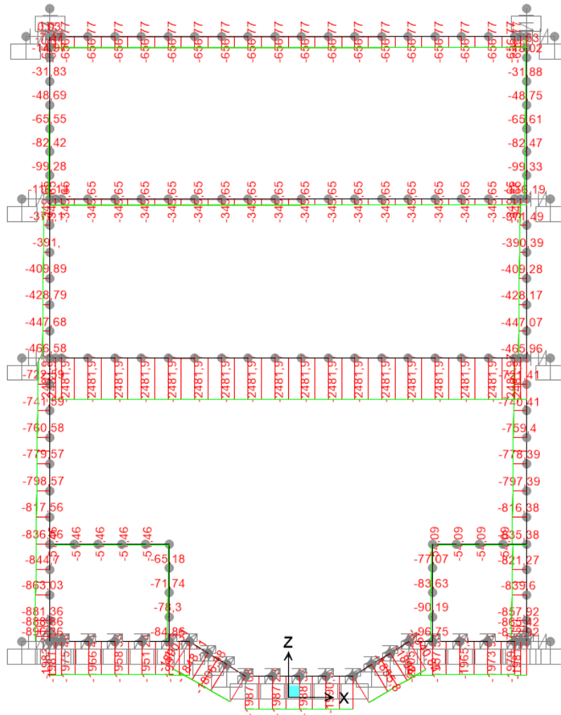
Figura 78.ENV N QUASI PERMANENTE
