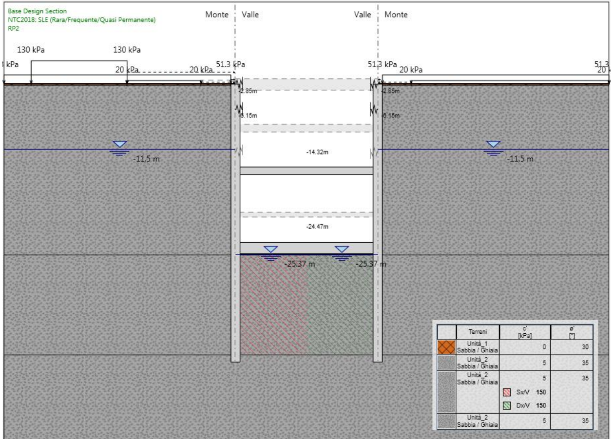
Figura 167.Fase 19: rimozione secondo ordine di puntelli metallici
