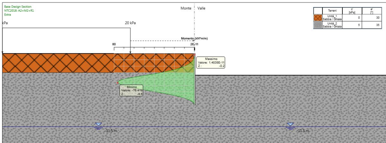
Figura 42. Involuppo dei momenti flettenti sulla berlinese provvisoriale (A2+M2+R1)
