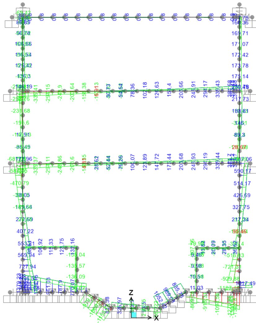
Figura 72.ENV V SLU/SLV
