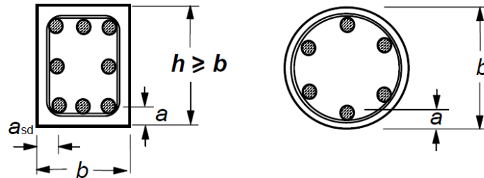
Figura 145. Sezioni degli elementi strutturali e distanza dall'asse a (UNI EN 1992-1-2:2005)
