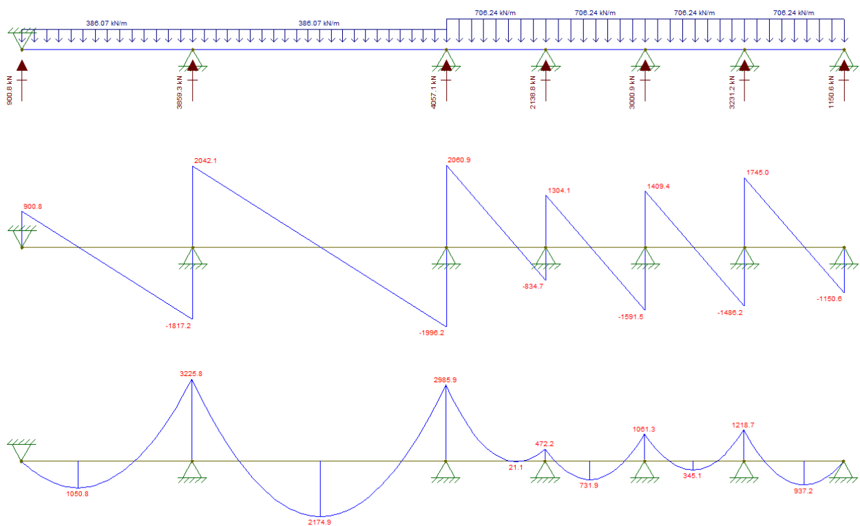
Figura 25. Sollecitazioni agenti nella trave di ripartizione del primo ordine (A1+M1+R1)
