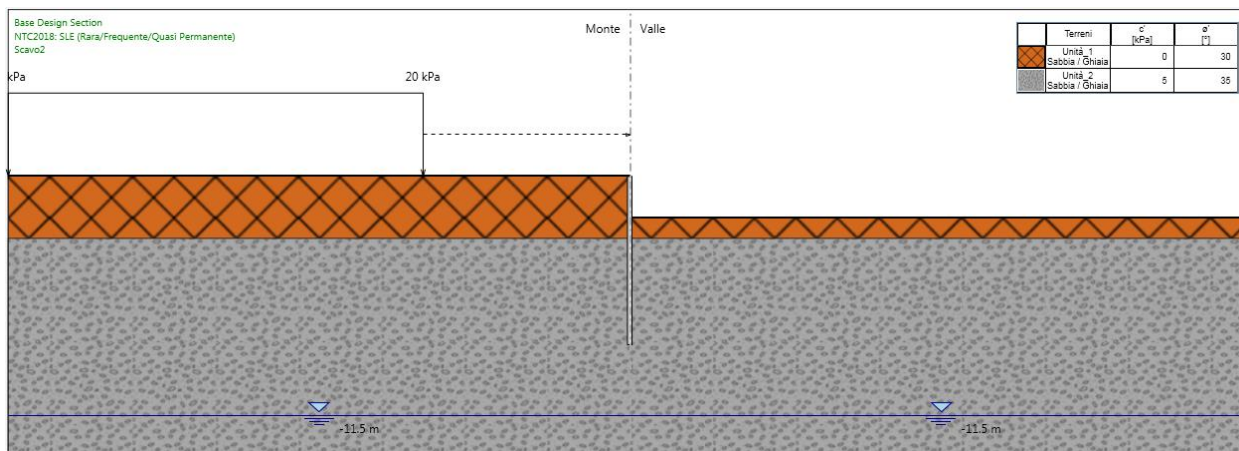
Figura 179.Fase 5: scavo a -2.0 m
