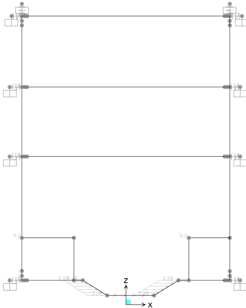
Figura 69.S2 inerzia sismica dei permanenti portati
