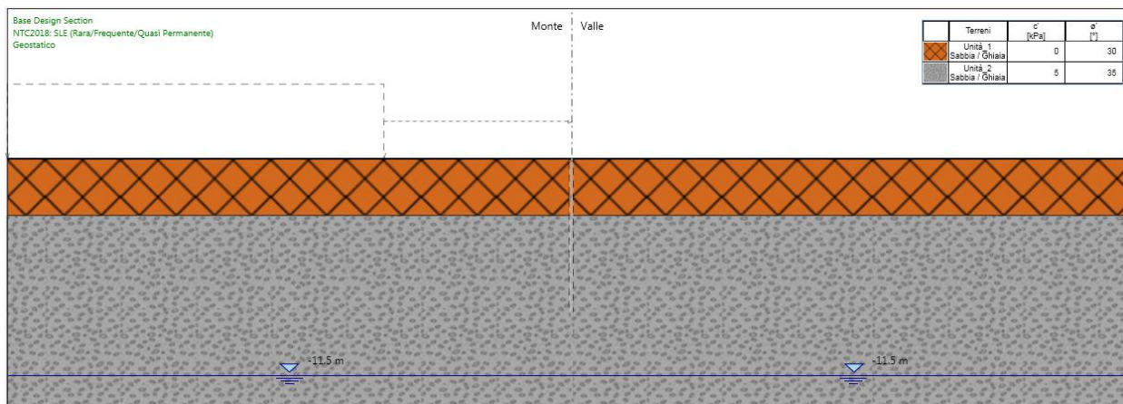
Figura 175.Fase 1: condizione geostatica
