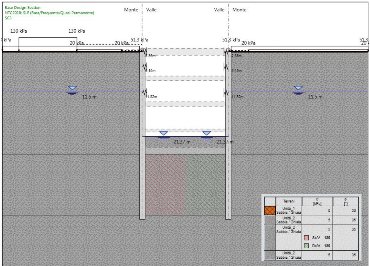
Figura 159.Fase 11: terzo scavo di ribasso
