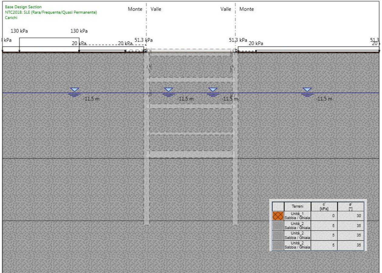
Figura 150.Fase 2: applicazione carichi preesistenze e scavo a quota realizzazione diaframmi
