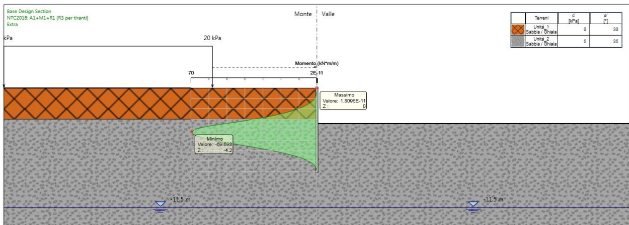
Figura 40. Involuppo dei momenti flettenti sulla berlinese provvisoriale (A1+M1+R1)
