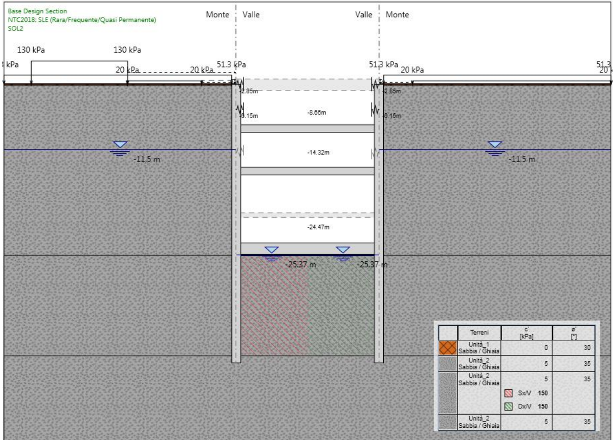
Figura 168.Fase 20: realizzazione secondo ordine di soletta in c.a.
