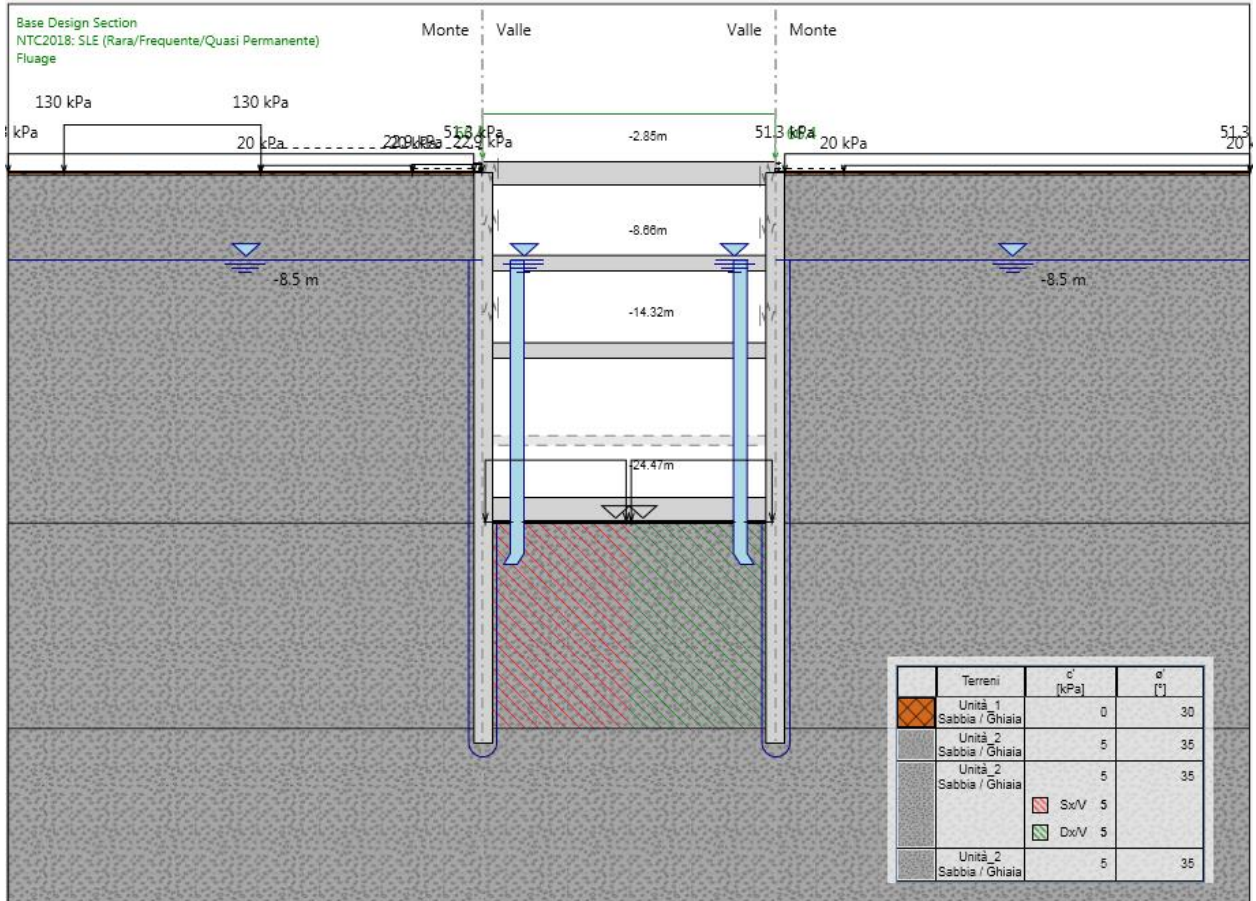
Figura 173.Fase 25 SLE: simulazione effetto fluage
