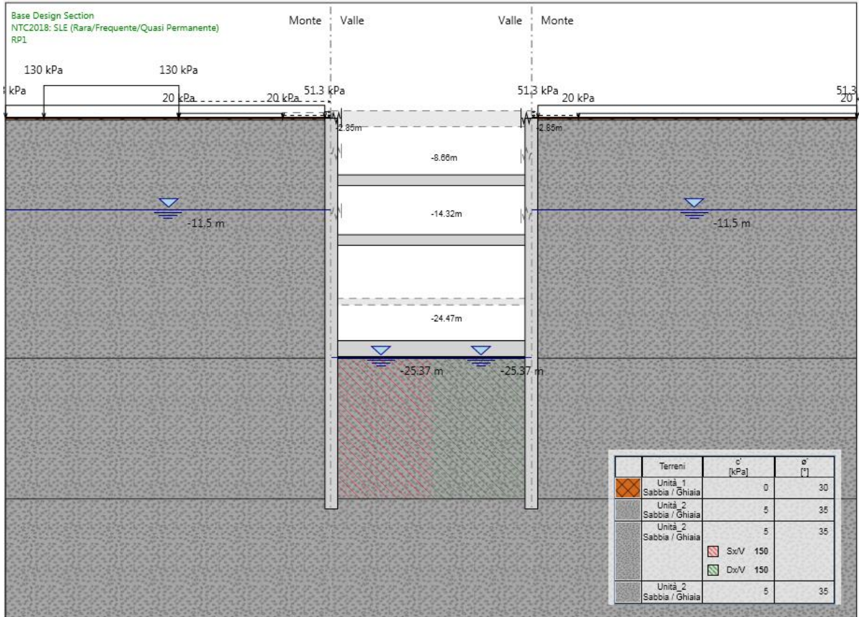
Figura 169.Fase 21: rimozione terzo ordine di puntelli metallici
