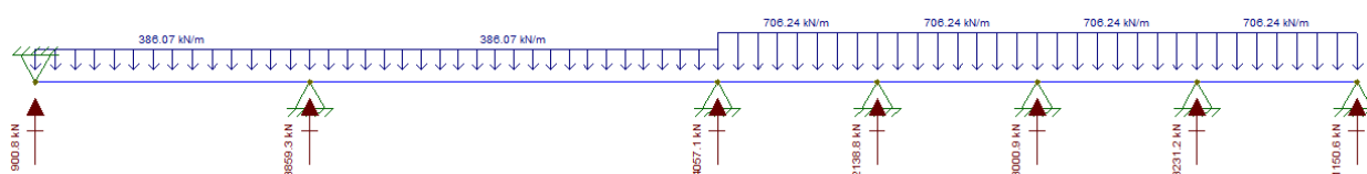
Figura 22. Azione agente sui puntelli metallici del primo ordine (A1+M1+R1)
