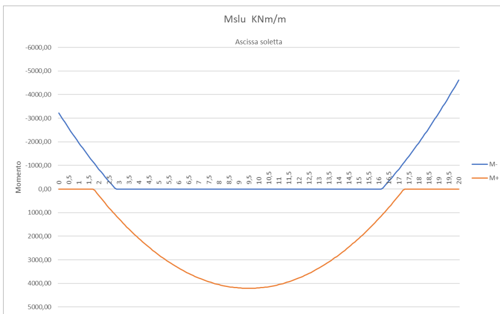
Figura 132.Momento flettente (SLU)
