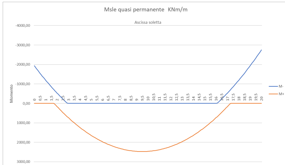
Figura 136.Momento flettente (SLE Quasi Permanente)
