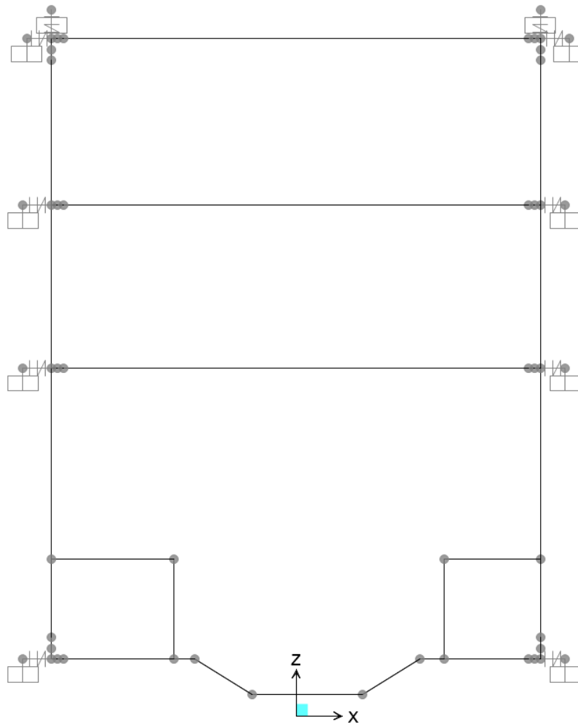
Figura 59. Vincoli del modello
