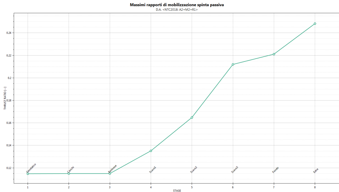
Figura 47. Resistenza passiva mobilitata in condizioni di stato limite ultimo (A2+M2+R1)
