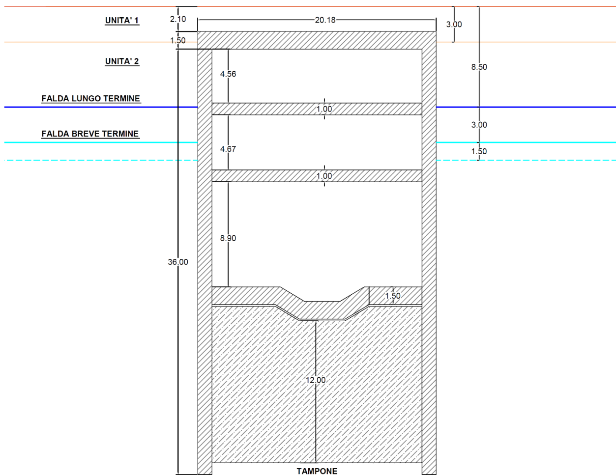
Figura 11. Dimensioni del modello di calcolo realizzato mediante Paratie Plus
