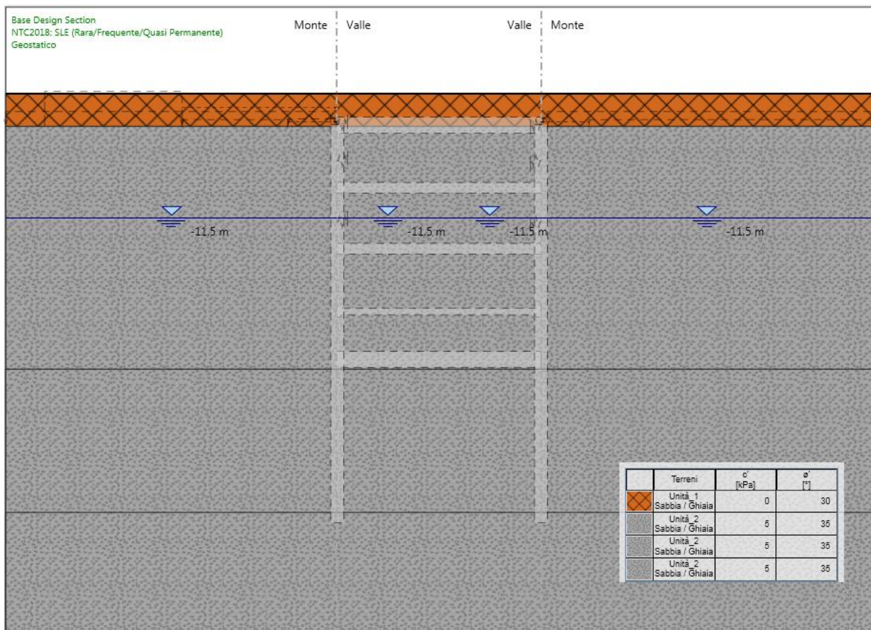
Figura 149.Fase 1: condizione geostatica
