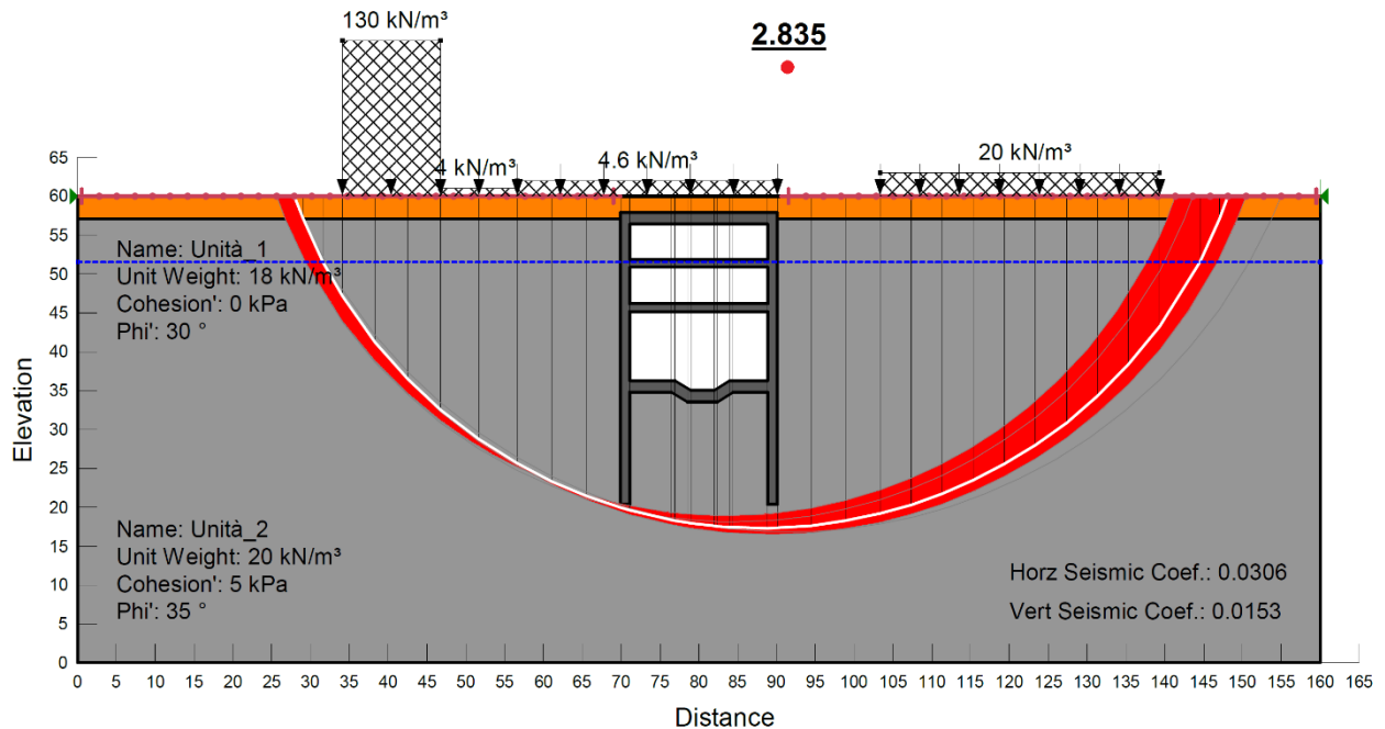
Figura 33.Verifica di stabilità globale in condizioni sismiche (kv positiva)
