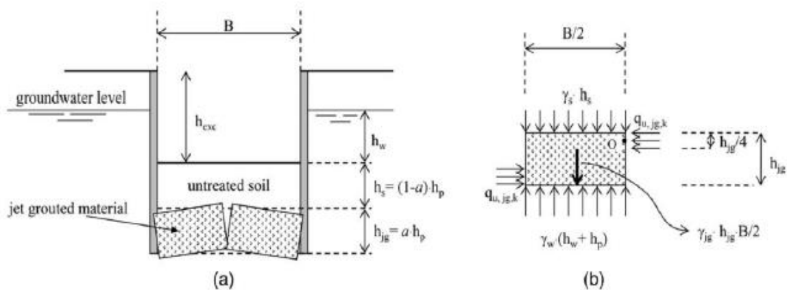
Figura 35. Meccanismo di rottura del tappo di fondo
