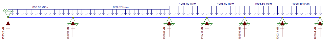
Figura 23. Azione agente sui puntelli metallici del secondo ordine (A1+M1+R1)
