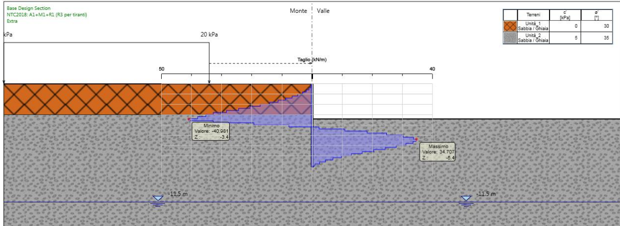
Figura 41. Involuppo del taglio sulla berlinese provvisoriale (A1+M1+R1)
