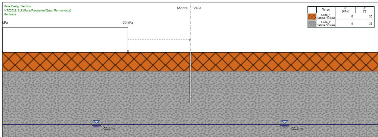
Figura 177.Fase 3: realizzazione berlinese di micropali
