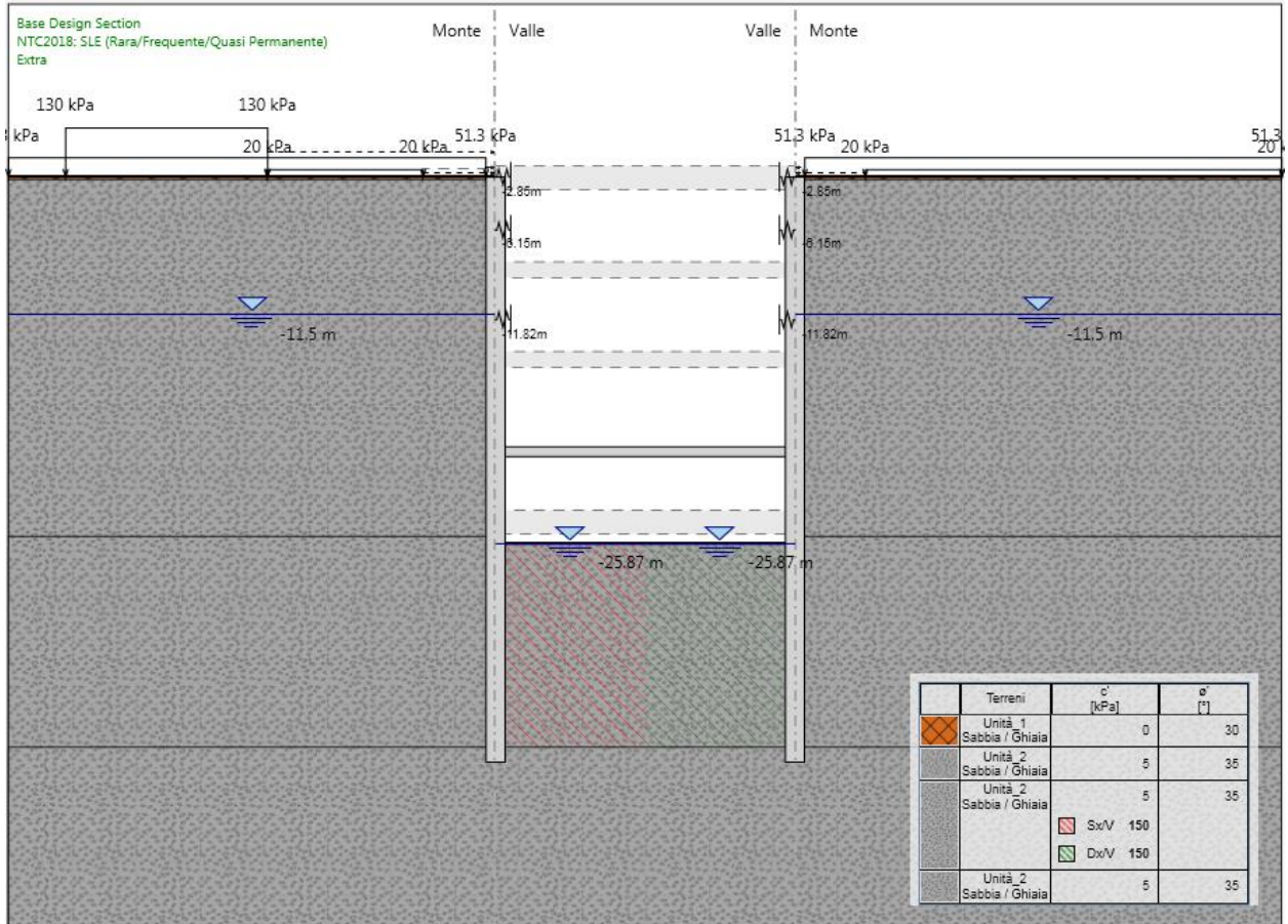
Figura 162.Fase 14: extra-scavo secondo NTC2018
