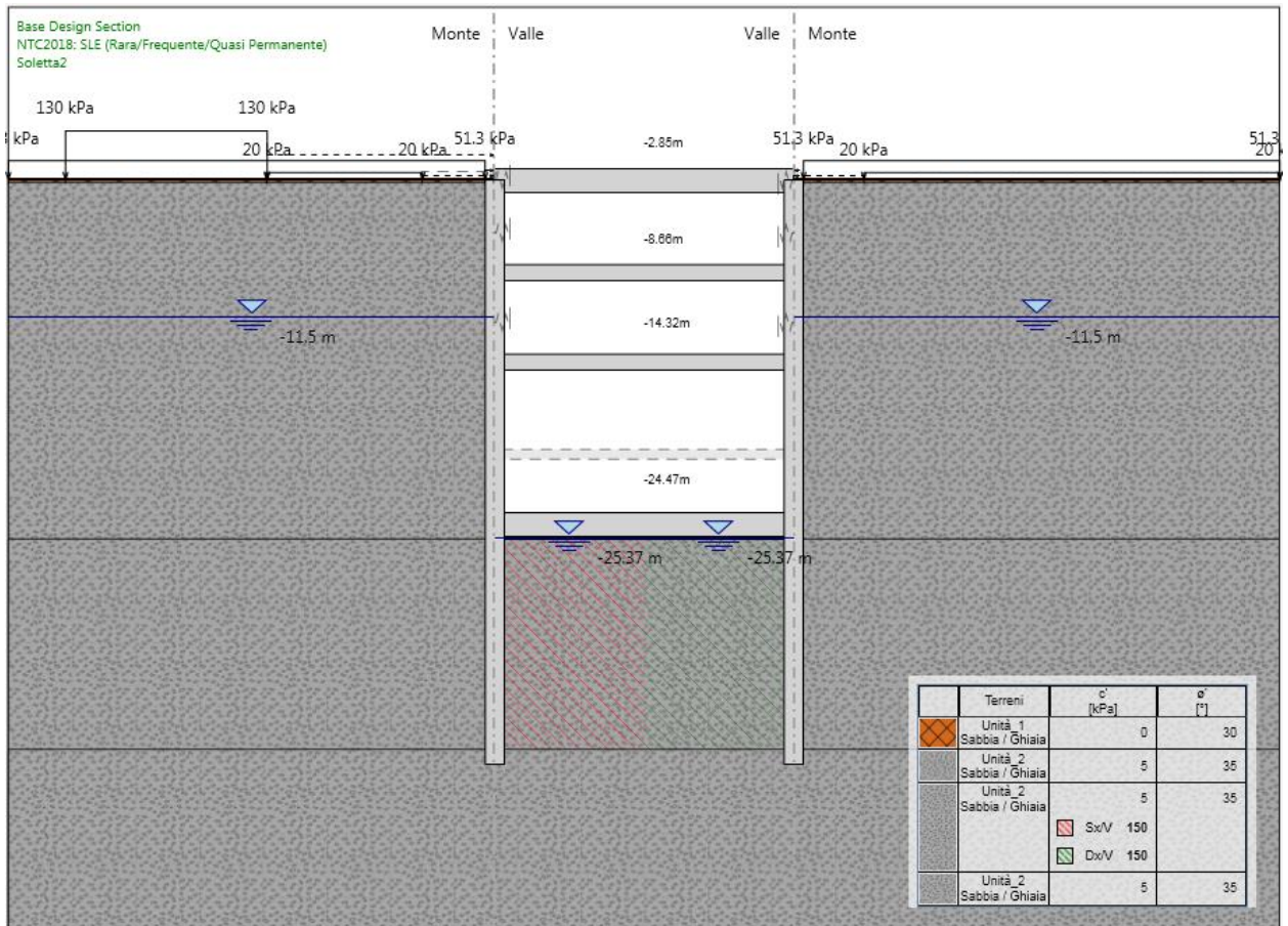
Figura 170.Fase 22: realizzazione soletta di copertura
