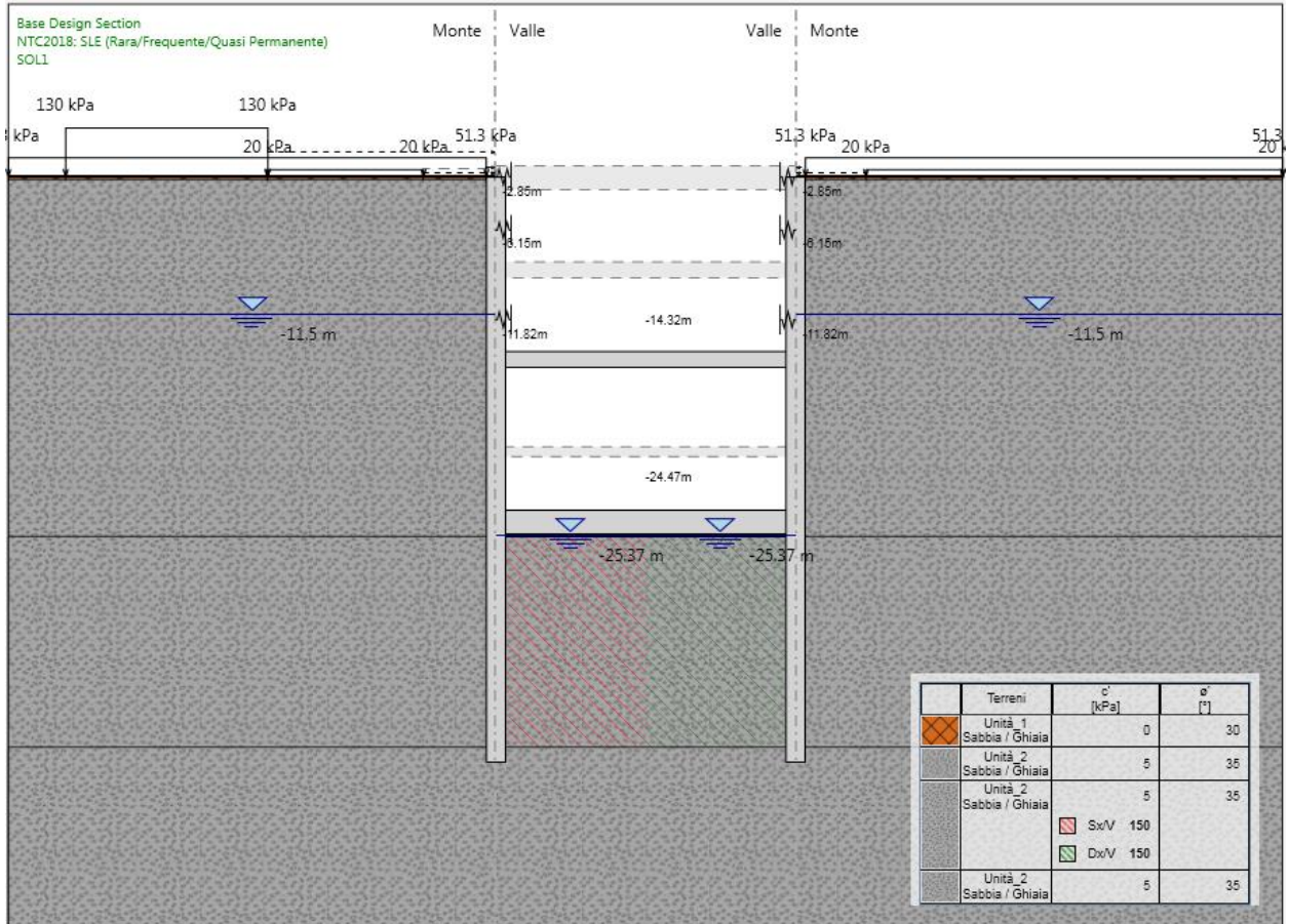
Figura 166.Fase 18: realizzazione primo ordine di soletta in c.a.
