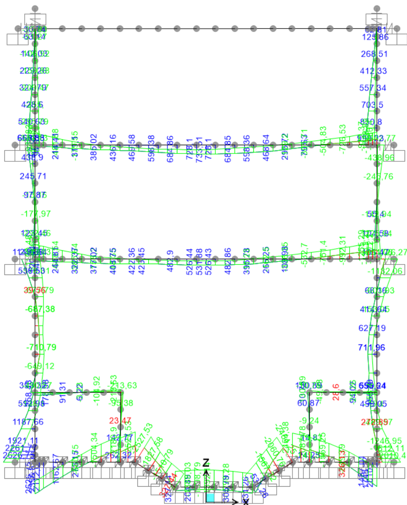
Figura 70.ENV M SLU/SLV
