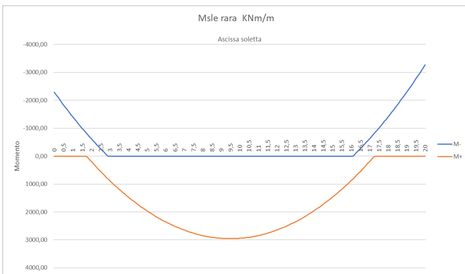
Figura 134.Momento flettente (SLE Rara)
