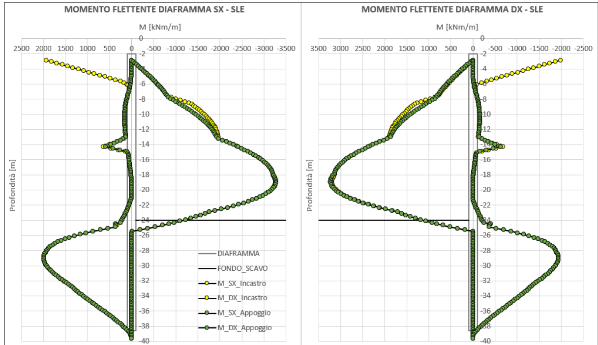
Figura 17. Inviluppo di momento flettente – SLE
