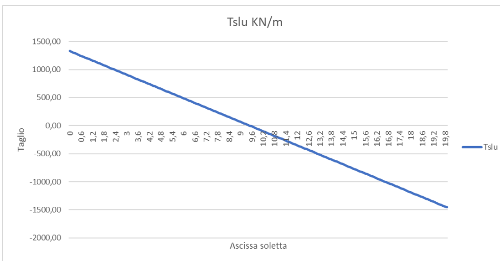
Figura 133.Taglio schema (SLU)
