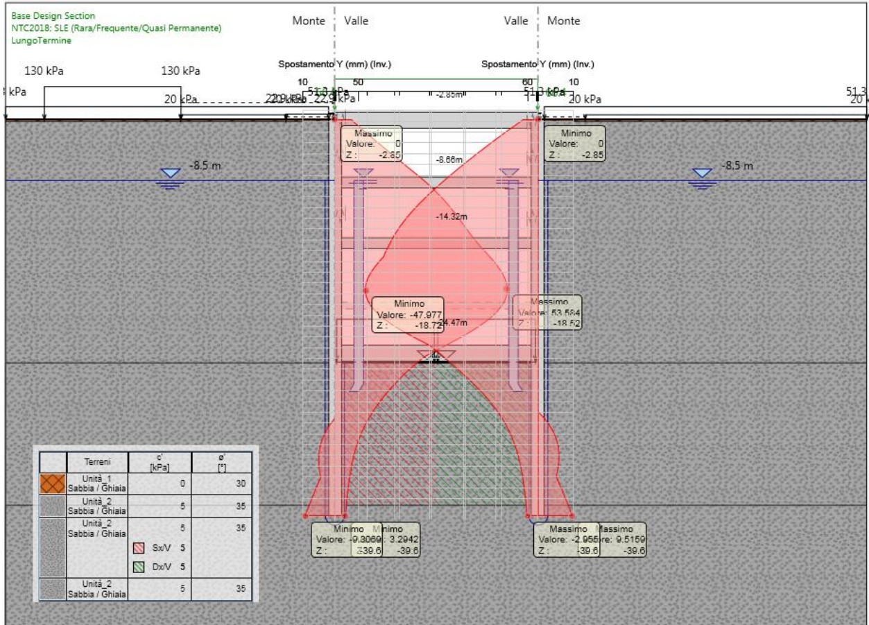
Figura 16.Spostamento massimo nella condizione di lungo termine - SLE
