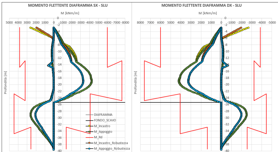
Figura 20. Diagramma di momento flettente agente e momento flettente resistente (SLU/SLV)
