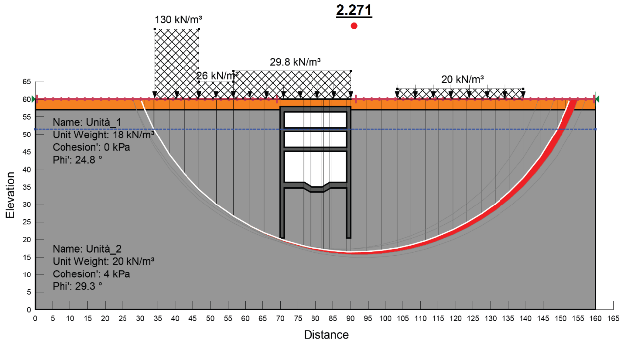
Figura 32.Verifica di stabilità globale in condizioni statiche
