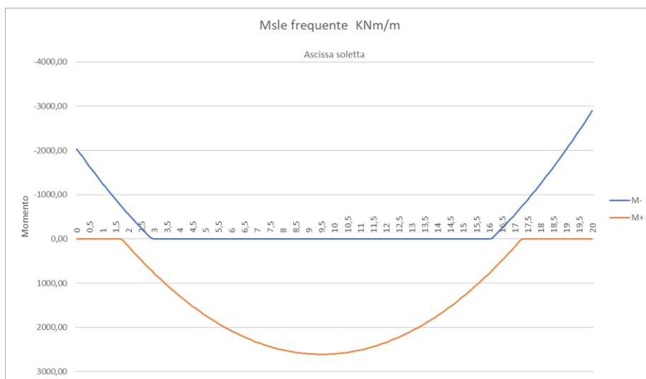
Figura 135.Momento flettente (SLE Frequente)
