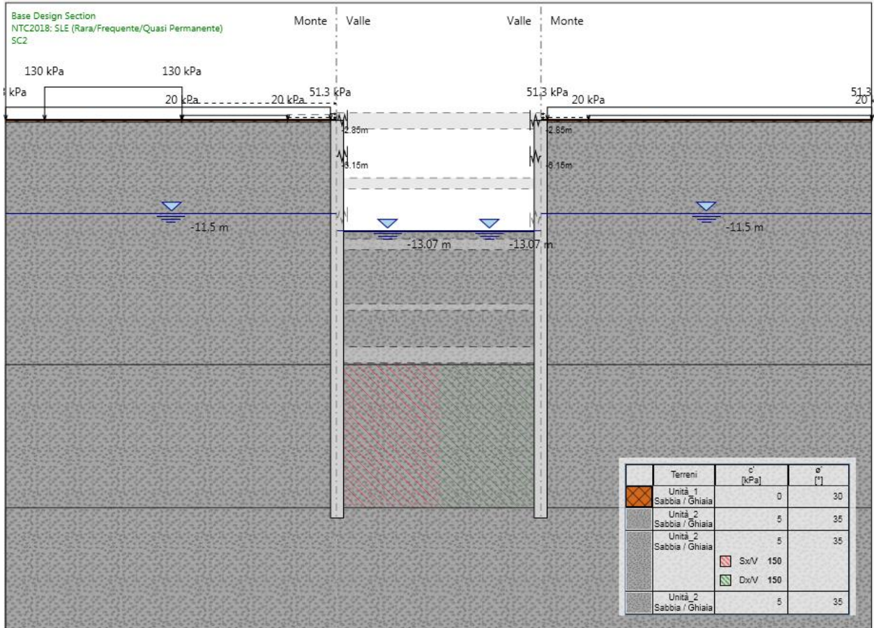
Figura 157.Fase 9: secondo scavo di ribasso
