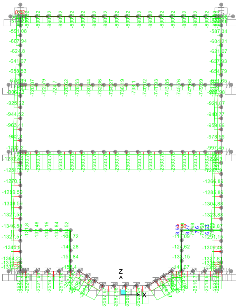
Figura 71.ENV N SLU/SLV
