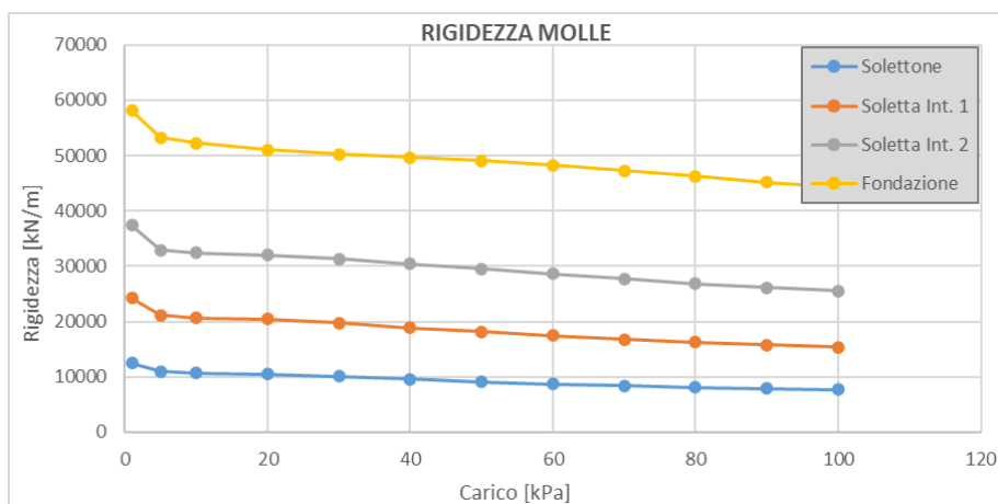
Figura 58.Andamento delle rigidezze
