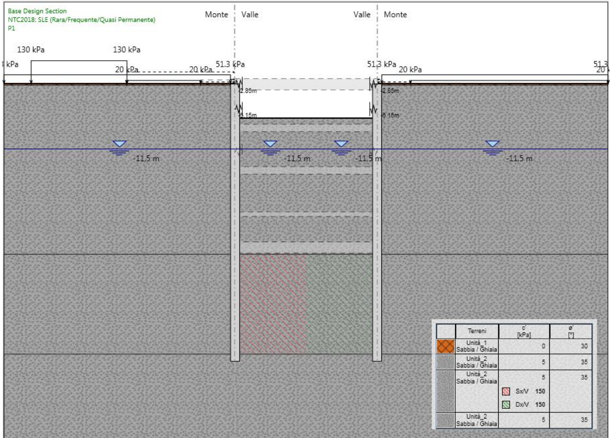
Figura 156.Fase 8: installazione primo ordine di travi di ripartizione (simulate mediante molle elastiche di rigidità equivalente)
