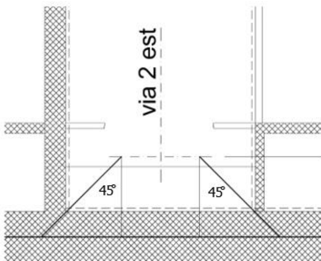
Figura 50. Distribuzione del carico sulla soletta
