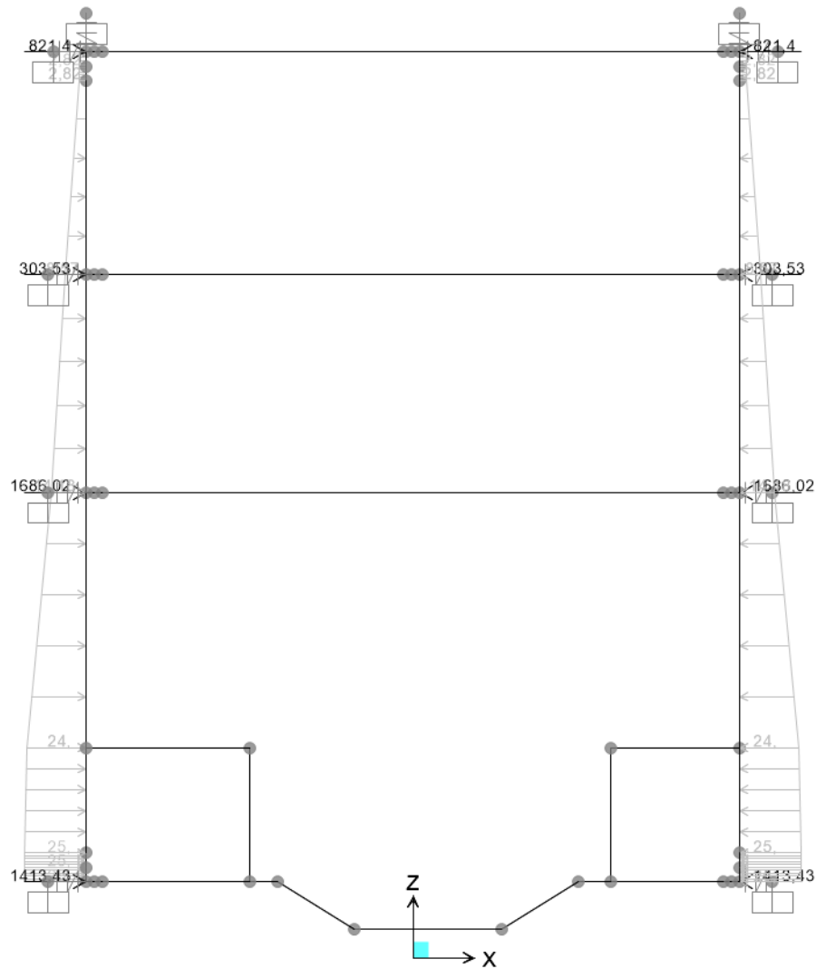
Figura 62.N SLU (terre)
