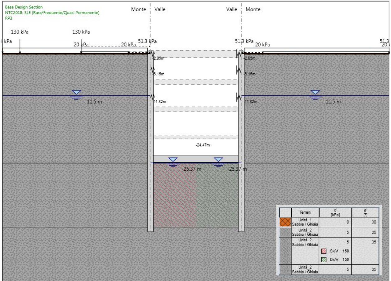
Figura 165.Fase 17: rimozione terzo ordine di puntelli metallici
