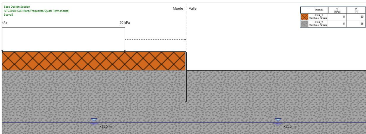
Figura 180.Fase 6: scavo a -3.0 m
