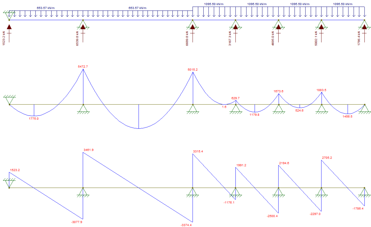
Figura 26.Sollecitazioni agenti nella trave di ripartizione del secondo ordine (A1+M1+R1)
