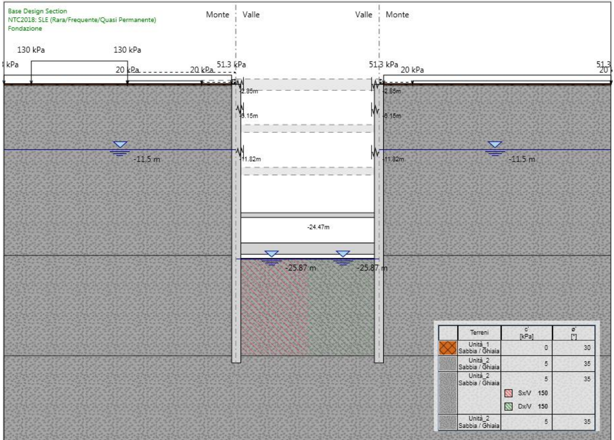
Figura 163.Fase 15: realizzazione soletta di fondazione
