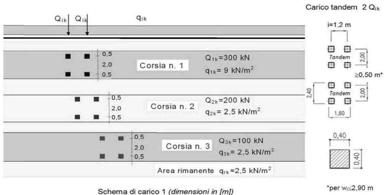
Figura 15. Schema di carico 1 previsto per la soletta di copertura
