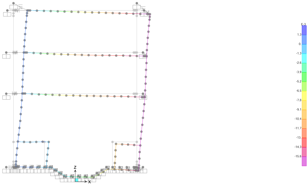
Figura 80.DEFORMATA SLV
