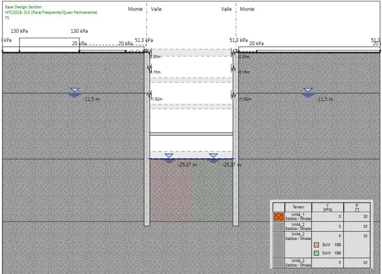
Figura 161.Fase 13: fondo scavo
