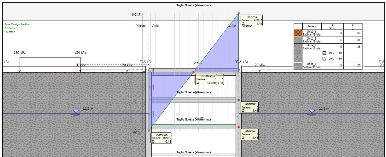
Figura 37. Taglio massimo agente sulla soletta di copertura (A1+M1+R3)
