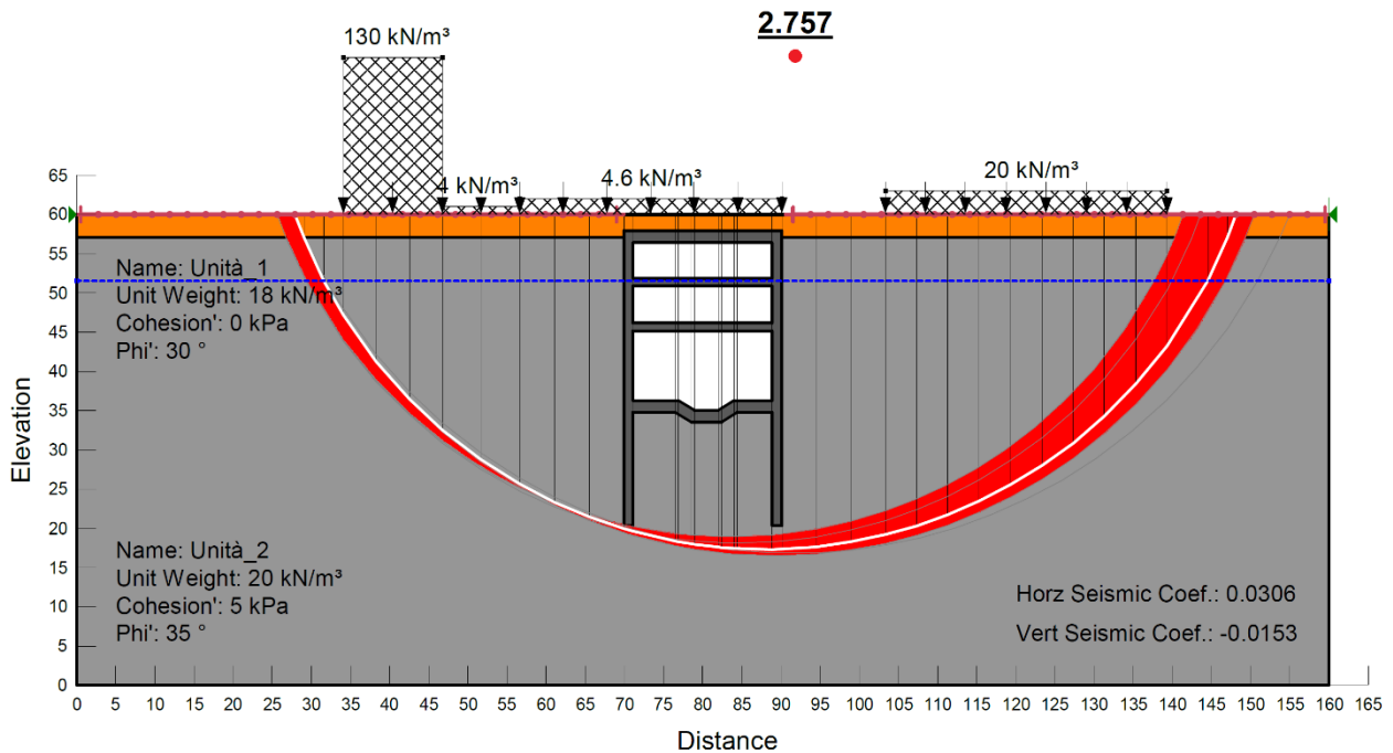
Figura 34. Verifica di stabilità globale in condizioni sismiche (kv negativa)
