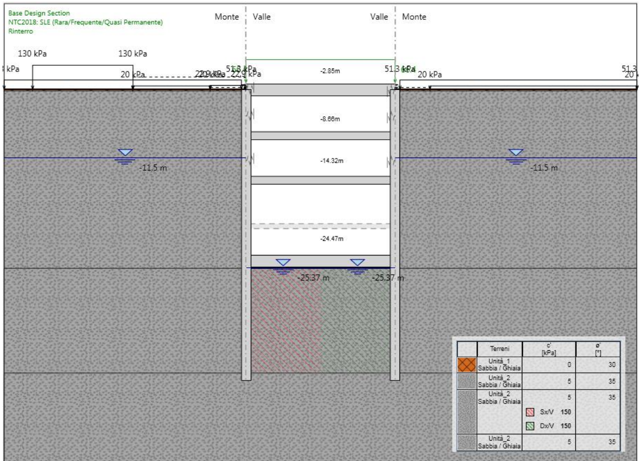
Figura 171.Fase 23: rinterro e applicazione carico accidentale
