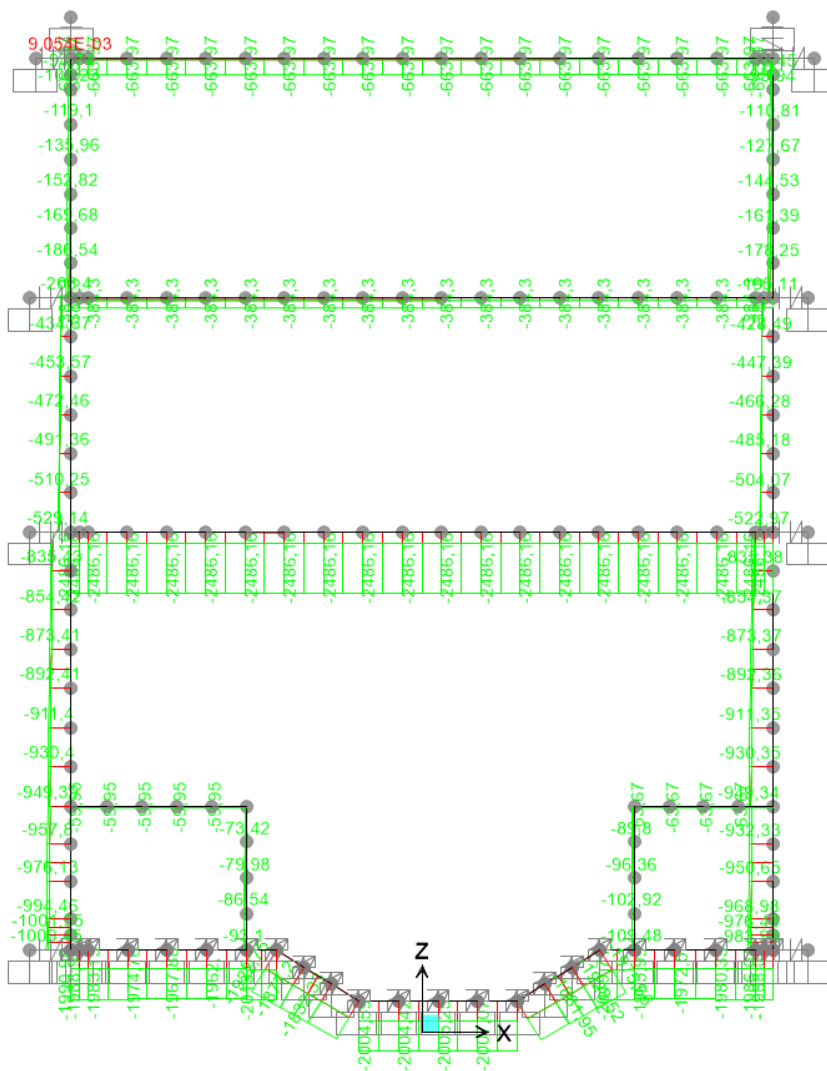
Figura 74.ENV N RARA
