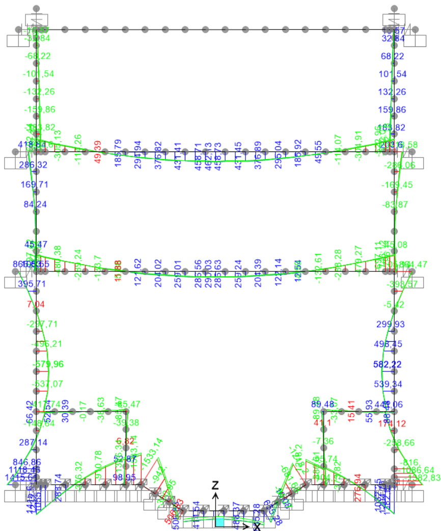
Figura 75.ENV M FREQUENTE
