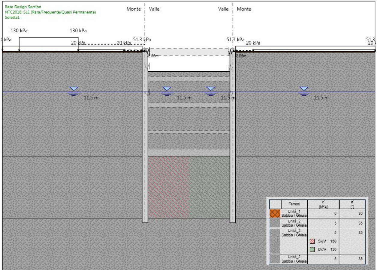
Figura 154.Fase 6: realizzazione cordoli di copertura (simulati mediante molle elastiche equivalenti)
