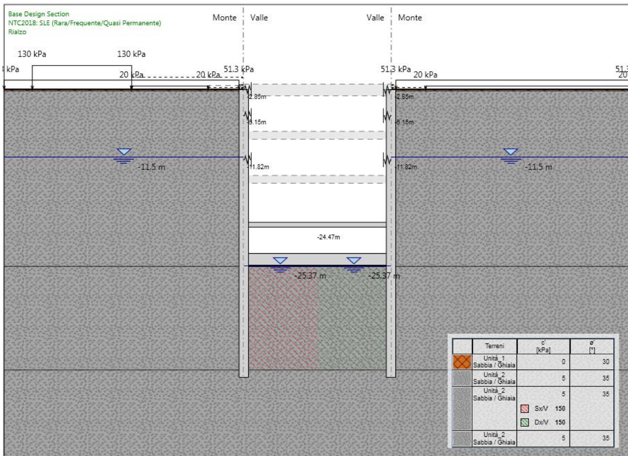
Figura 164.Fase 16: rialzo a quota di fondo scavo
