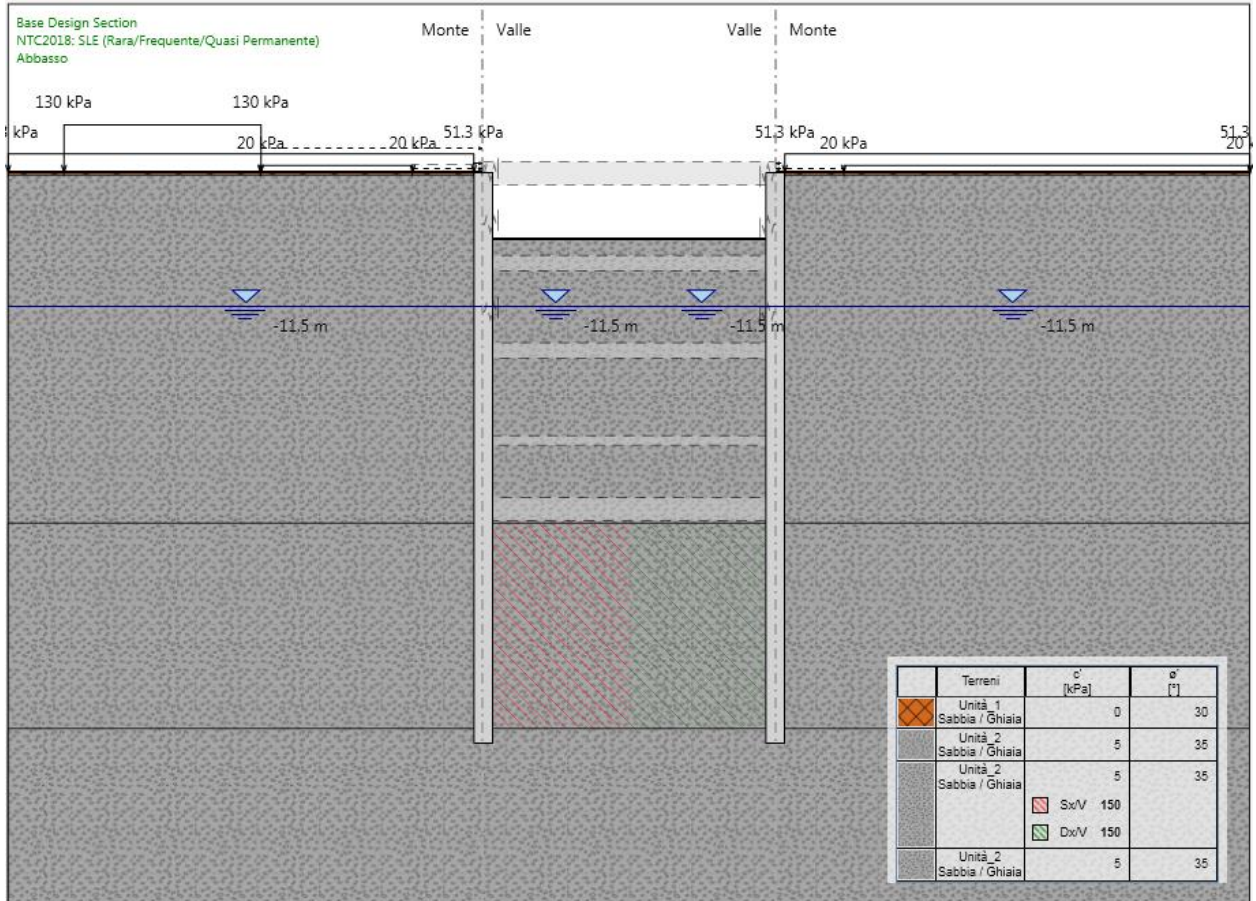
Figura 153.Fase 5: ribasso fino a quota realizzazione soletta di copertura
