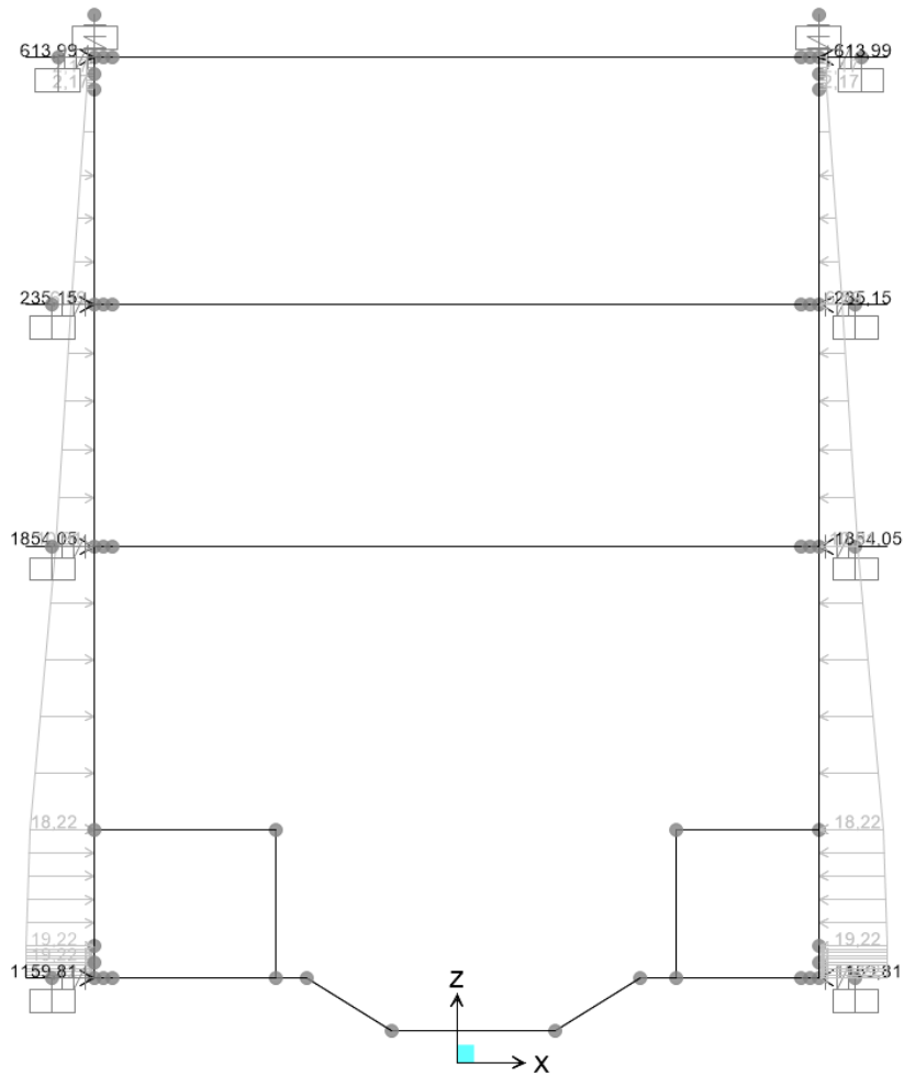
Figura 61.N sle (terre)
