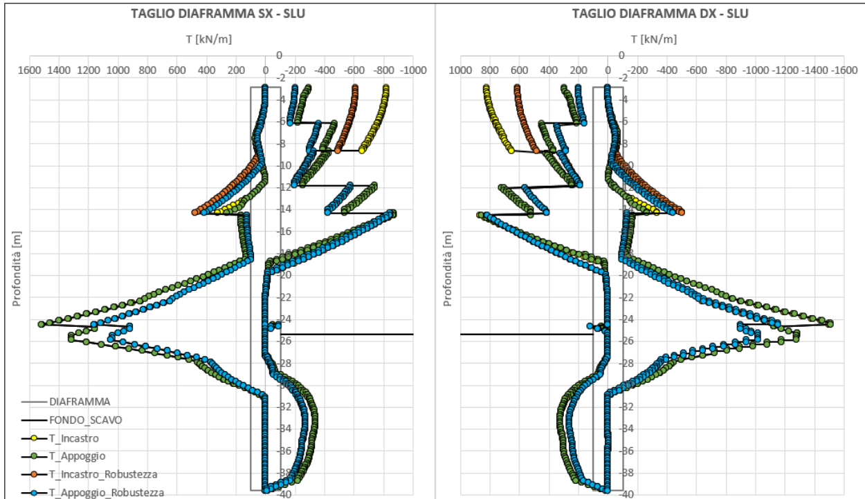
Figura 19. Involuppo di taglio – SLU / SLV
