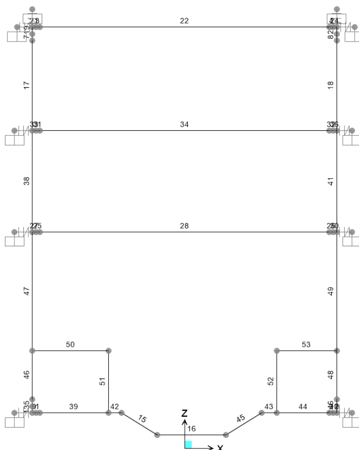
Figura 56. Numerazione delle aste
