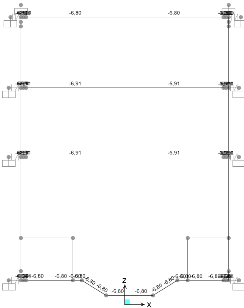
Figura 64.Ritiro
