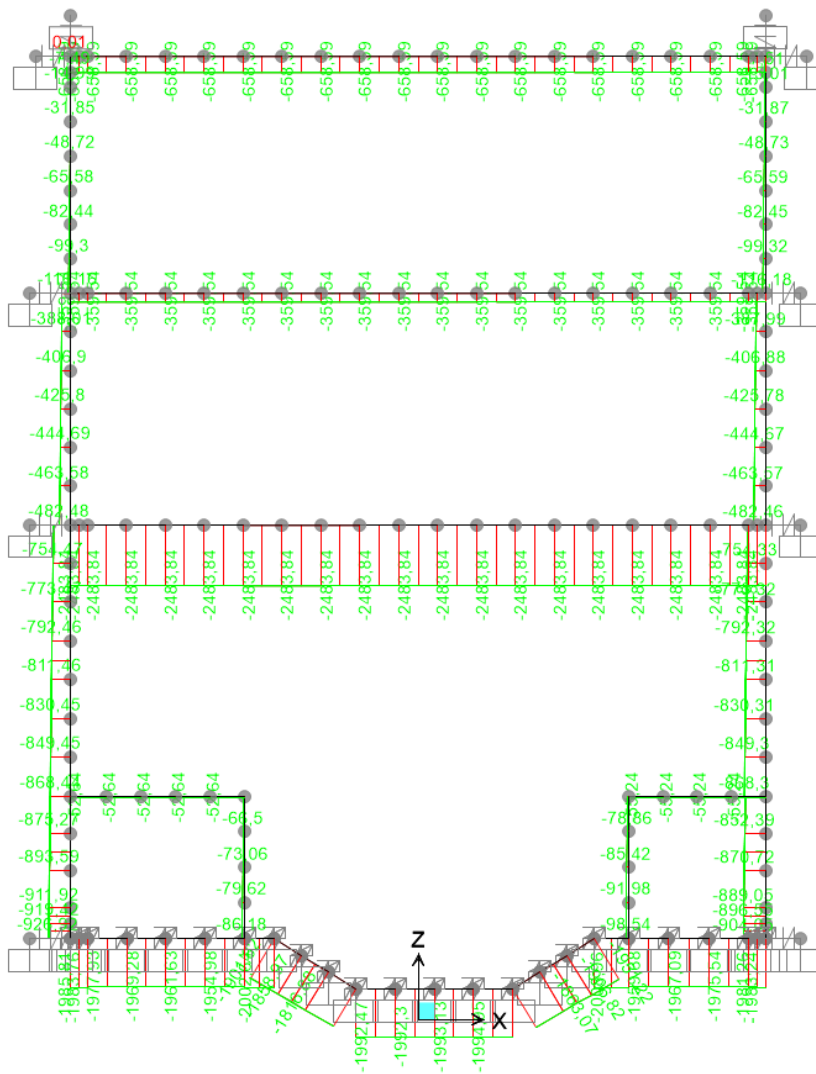
Figura 76.ENV N FREQUENTE
