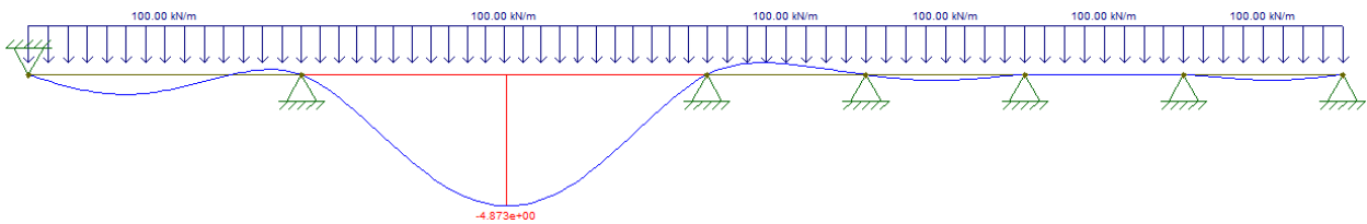
Figura 13.Schema trave su "n" appoggi (gli appoggi simulano la presenza dei puntelli metallici)
