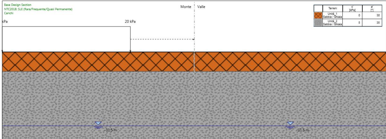
Figura 176.Fase 2: applicazione carico preesistenze
