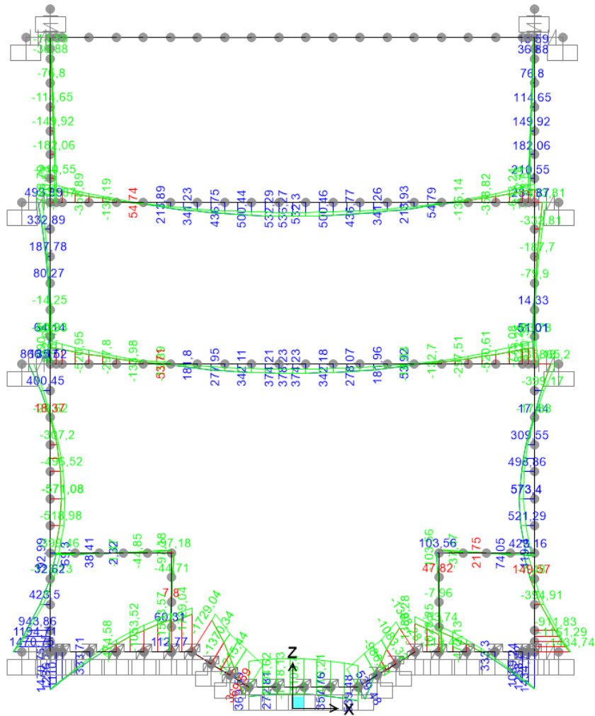
Figura 73.ENV M RARA
