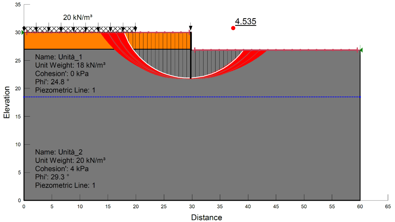
Figura 48.Verifica di stabilità globale della berlinese provvisoria in condizioni statiche
