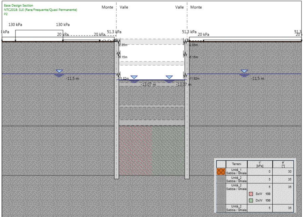
Figura 158.Fase 10: installazione secondo ordine di travi di ripartizione (simulate mediante molle elastiche di rigidità equivalente)
