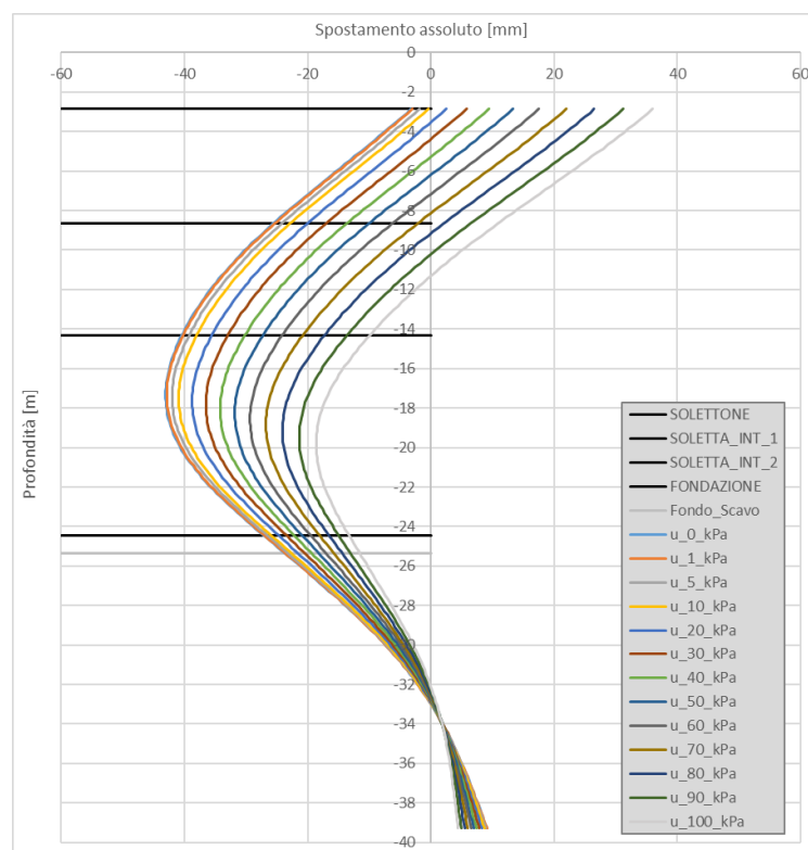
Figura 57. Grafico spostamento assoluto-profondità paratie
