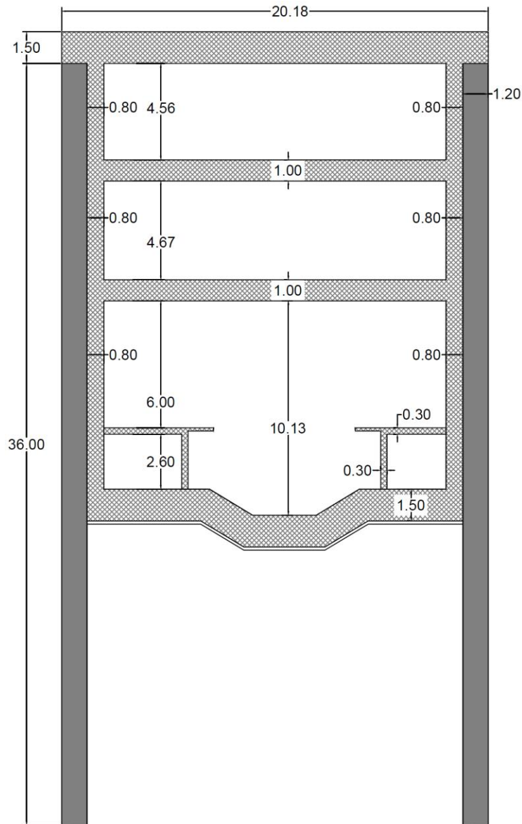
Figura 3. Esempio di sezione trasversale del pozzo Novara
