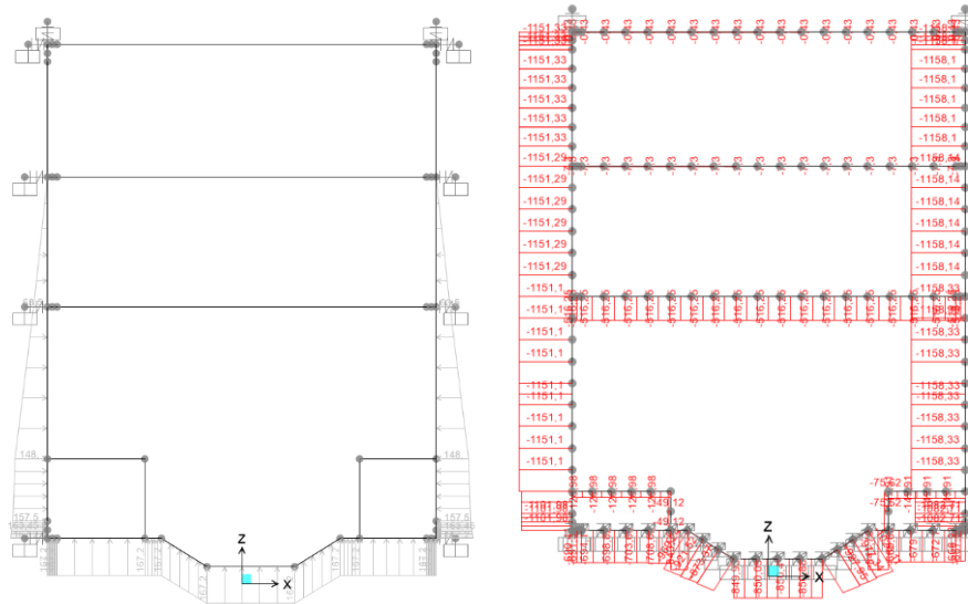
Figura 51. Modello delle strutture interne soggette a spinta idrostatica della falda e conseguenti sollecitazioni assiali
