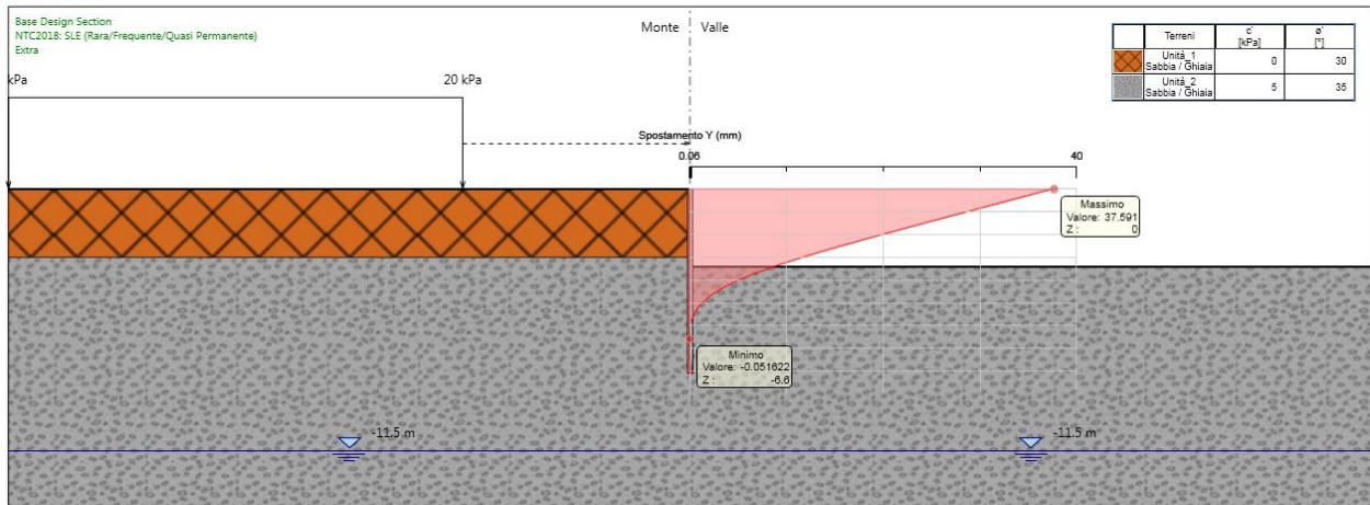
Figura 39. Involuppo degli spostamenti sulla berlinese provvisoriale (SLE)
