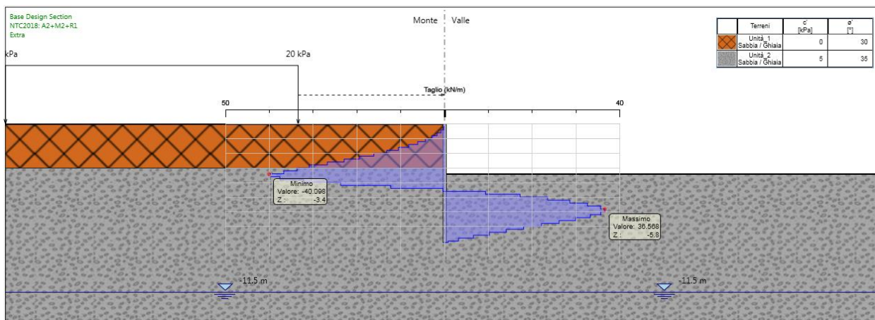
Figura 43. Involuppo del taglio sulla berlinese provvisoriale (A2+M2+R1)
