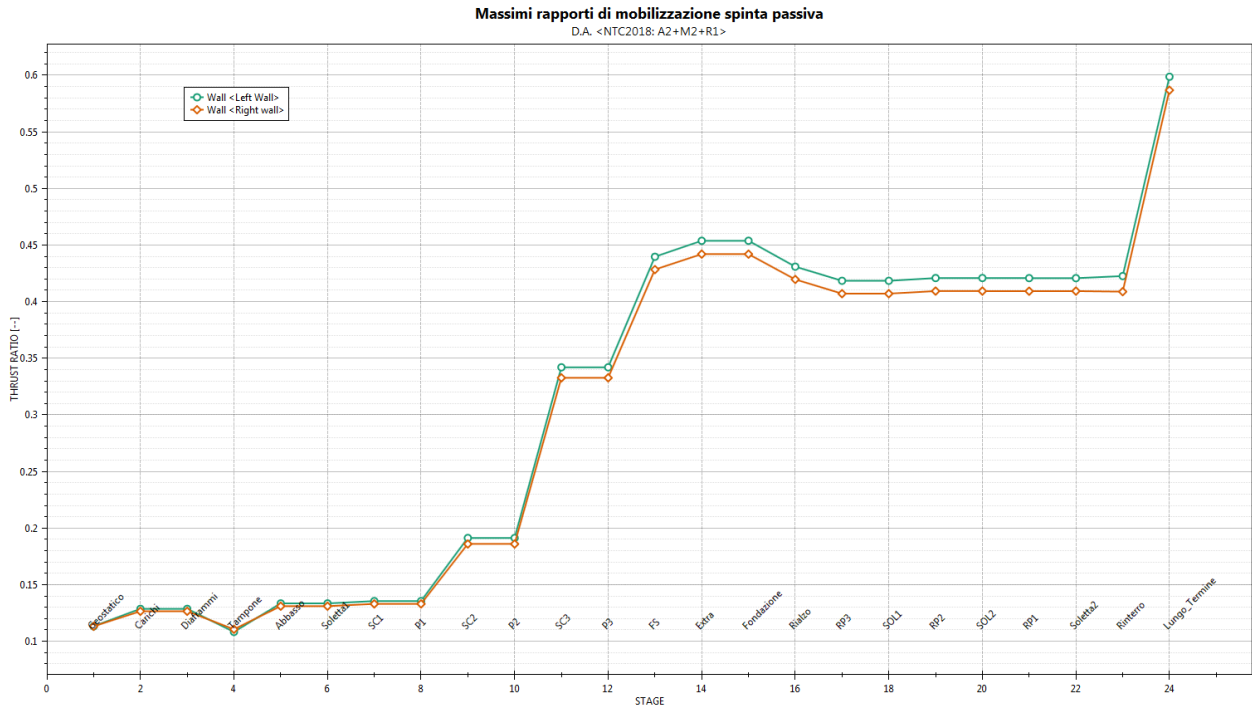
Figura 30. Resistenza passiva mobilitata in condizioni di stato limite ultimo (A2+M2)
