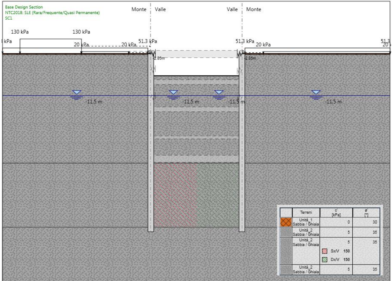
Figura 155.Fase 7: primo scavo di ribasso
