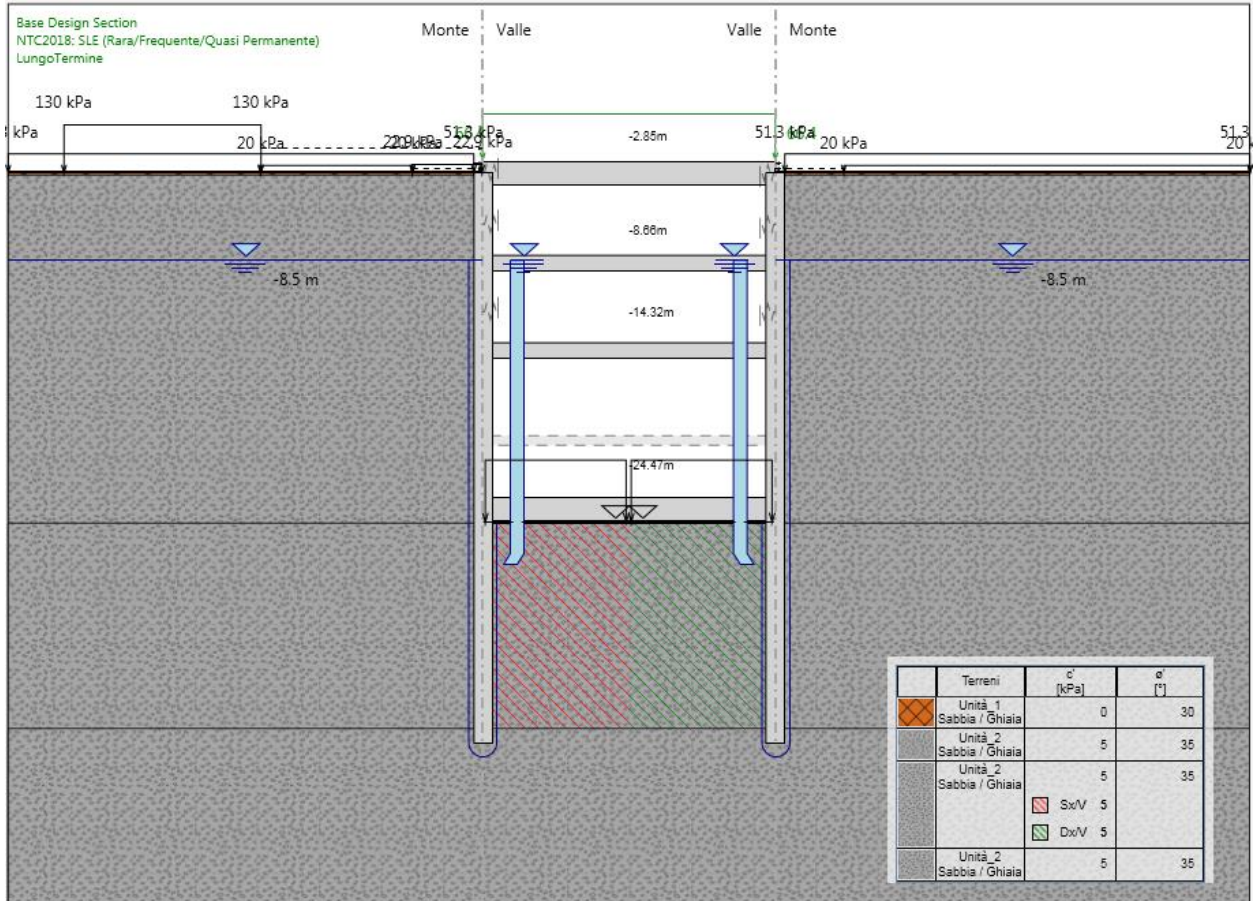
Figura 172.Fase 24: condizione di lungo termine
