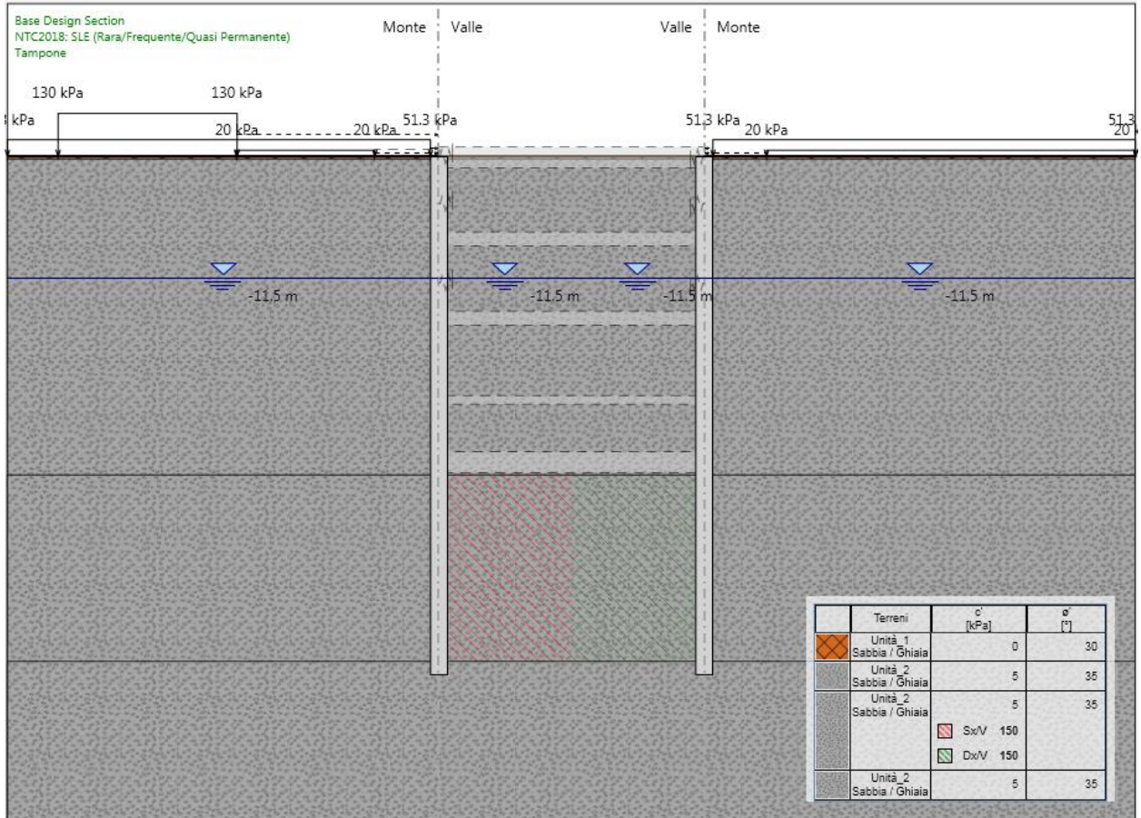
Figura 152.Fase 4: realizzazione tampone di fondo
