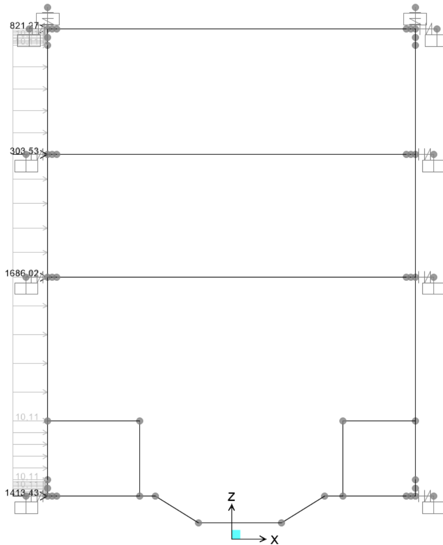
Figura 67.S1 azione sismica
