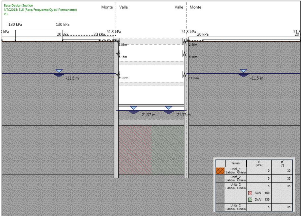
Figura 160.Fase 12: installazione terzo ordine di puntelli metallici
