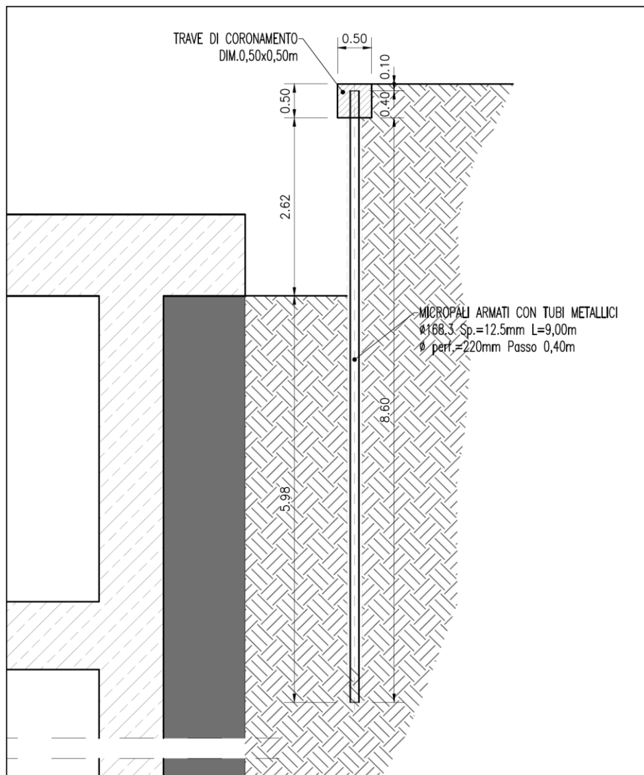
Figura 38.Rappresentazione grafica della berlinese oggetto di studio
