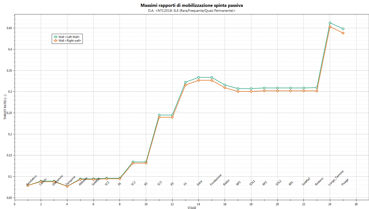
Figura 29. Resistenza passiva mobilitata in condizioni di stato limite di esercizio (SLE)
