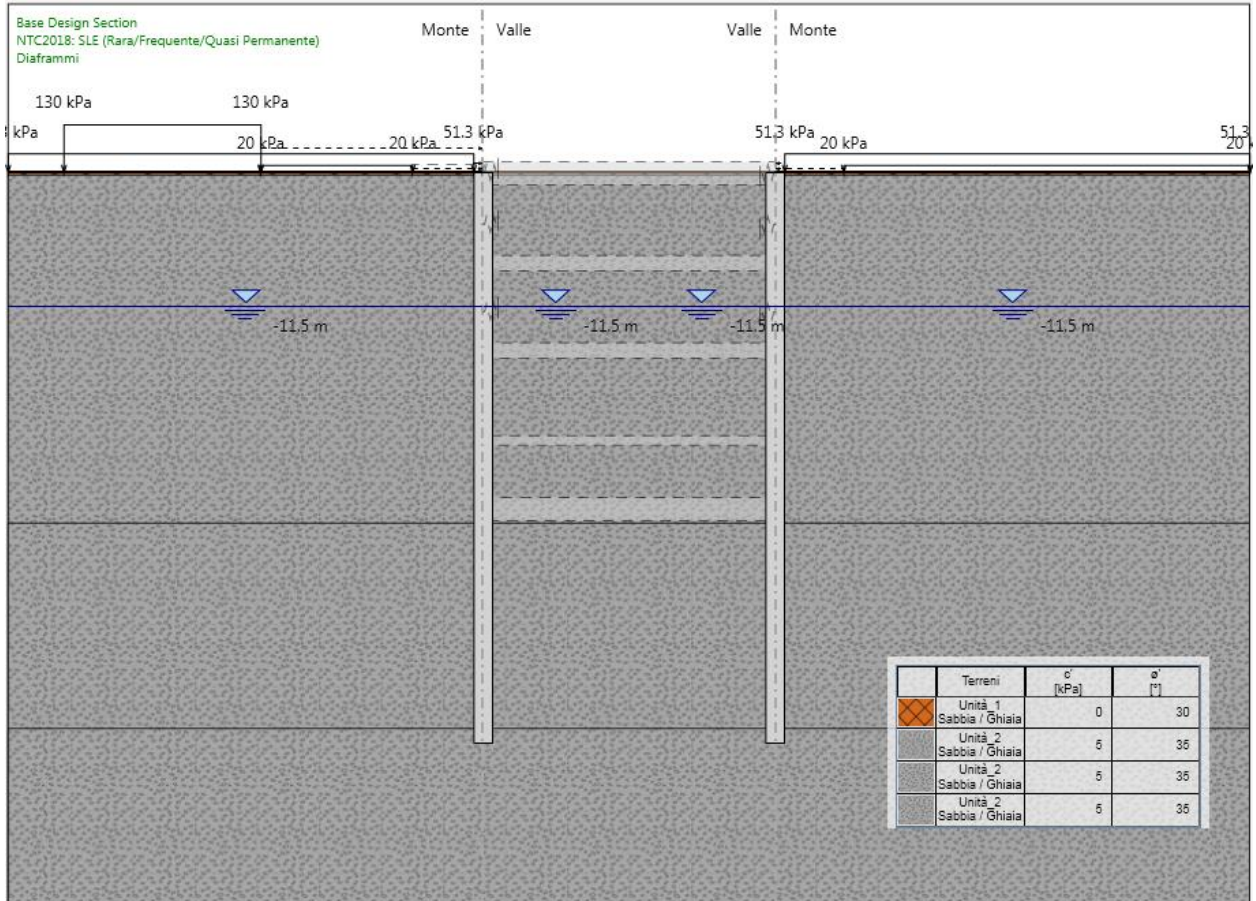
Figura 151.Fase 3: realizzazione diaframmi
