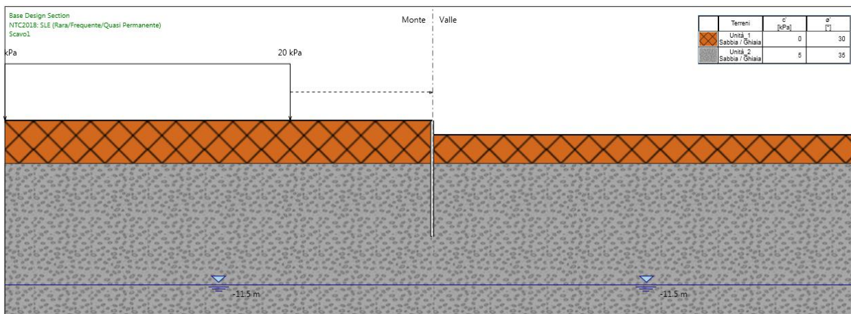
Figura 178.Fase 4: scavo a -1.0 m
