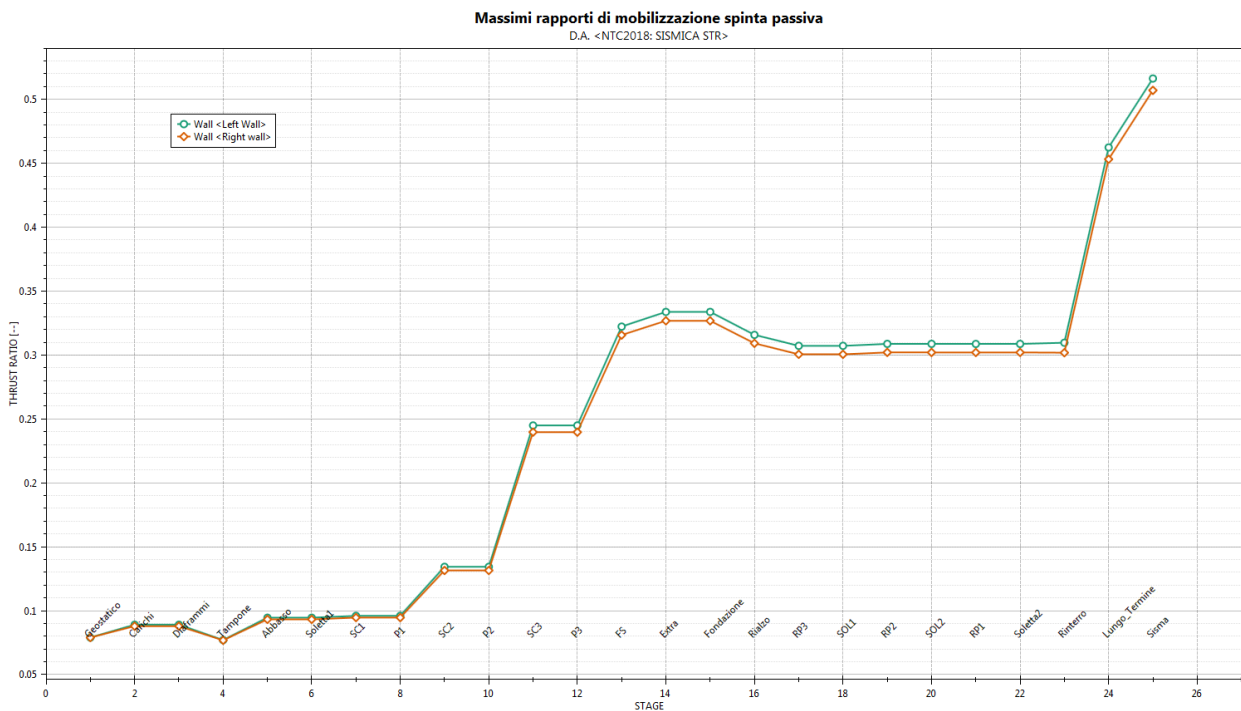
Figura 31. Resistenza passiva mobilitata in condizioni sismiche (A1+M1+R1 / SISMA)
