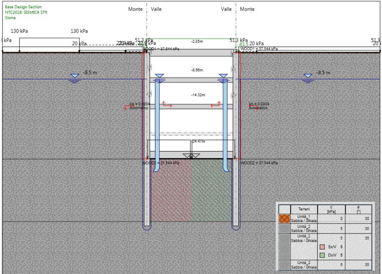
Figura 174.Fase 25 SLU/SLV: simulazione condizione sismica
