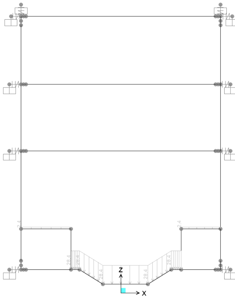
Figura 60.G2 carichi permanenti portati
