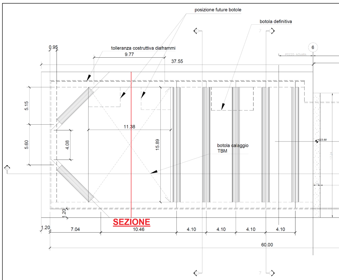
Figura 14. Sezione di calcolo – vista in pianta
