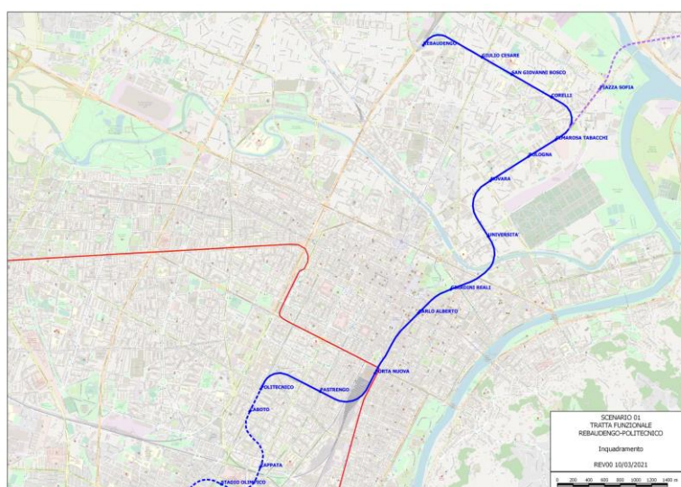
Figura 1. Key-plan della linea 2 – tratta funzionale Politecnico-Rebaudengo
