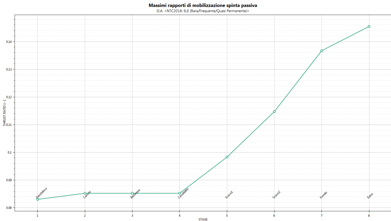
Figura 23. Resistenza passiva mobilitata in condizioni di esercizio (SLE)
