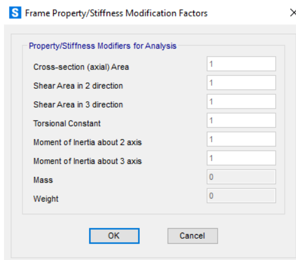
Figura 30. Proprietà meccaniche della sezione della copertura del modello
