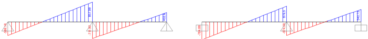
Figura 104.Taglio schema (SLU)
