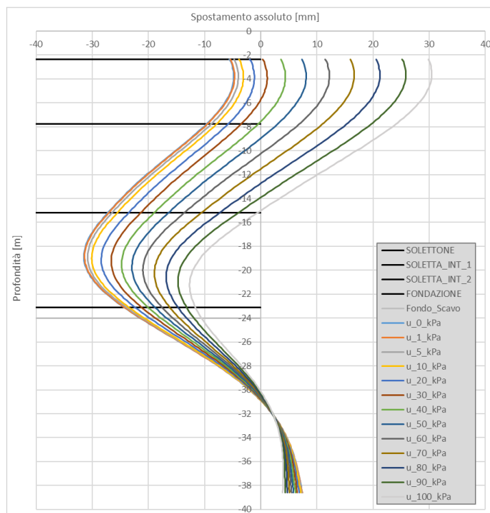
Figura 33. Grafico spostamento assoluto-profondità paratie
