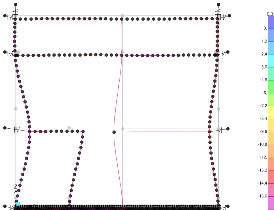
Figura 60.DEFORMATA SLU
