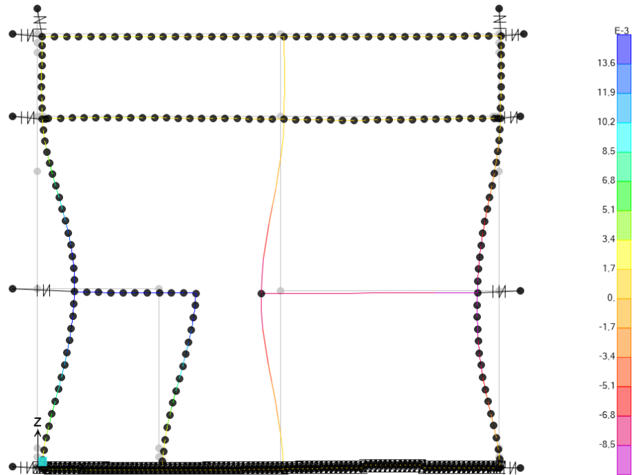
Figura 61.DEFORMATA SLV
