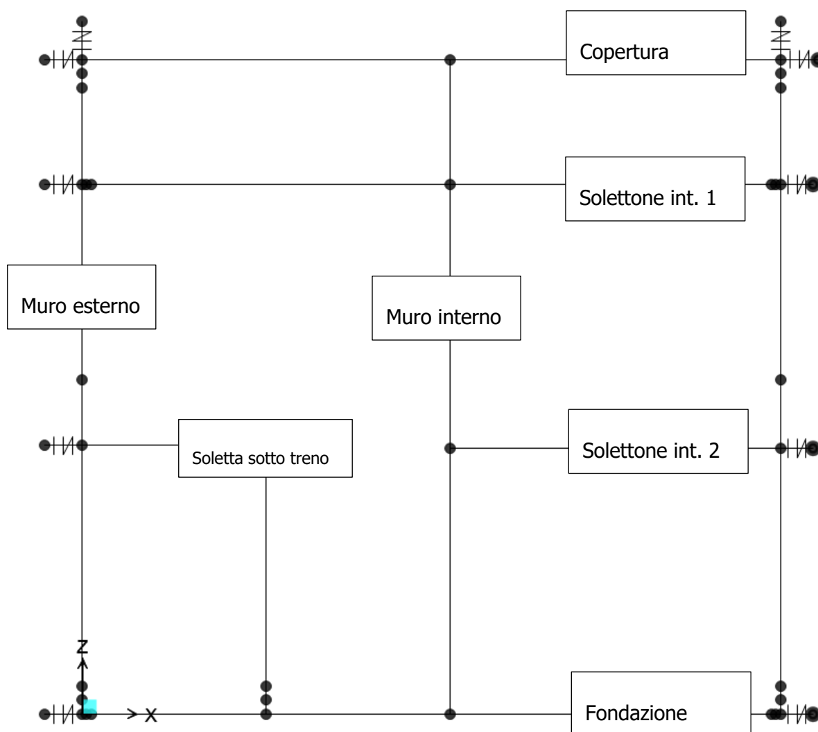
Figura 64. Legenda delle componenti strutturali
