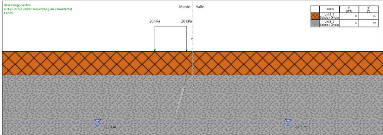
Figura 120.Fase 2: applicazione carico stradale
