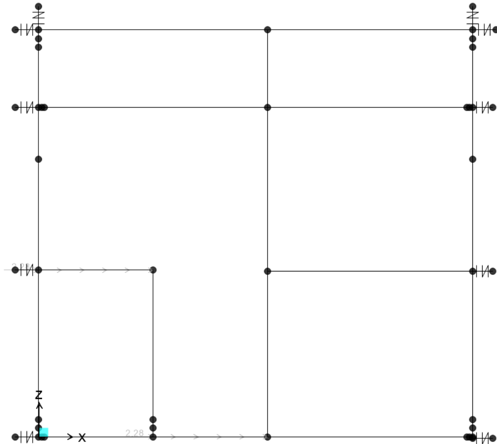
Figura 45.S2 inerzia sismica dei permanenti portati
