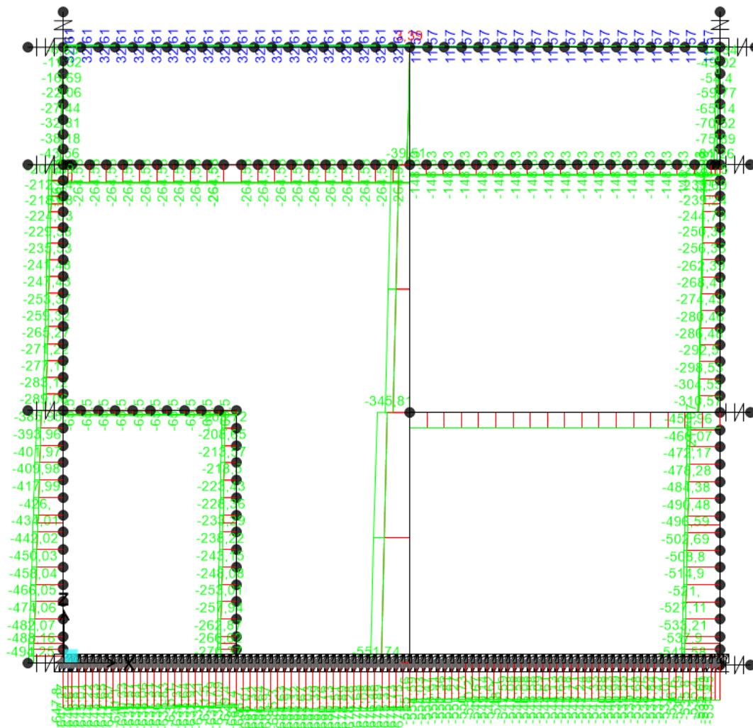
Figura 53.ENV N RARA
