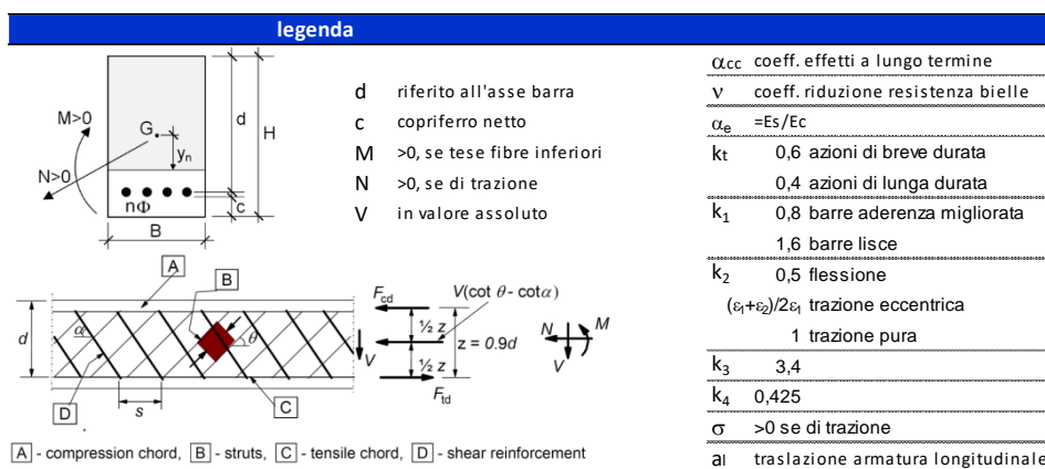
Figura 107. Convenzioni adottate per la verifica sezione in c.a.
