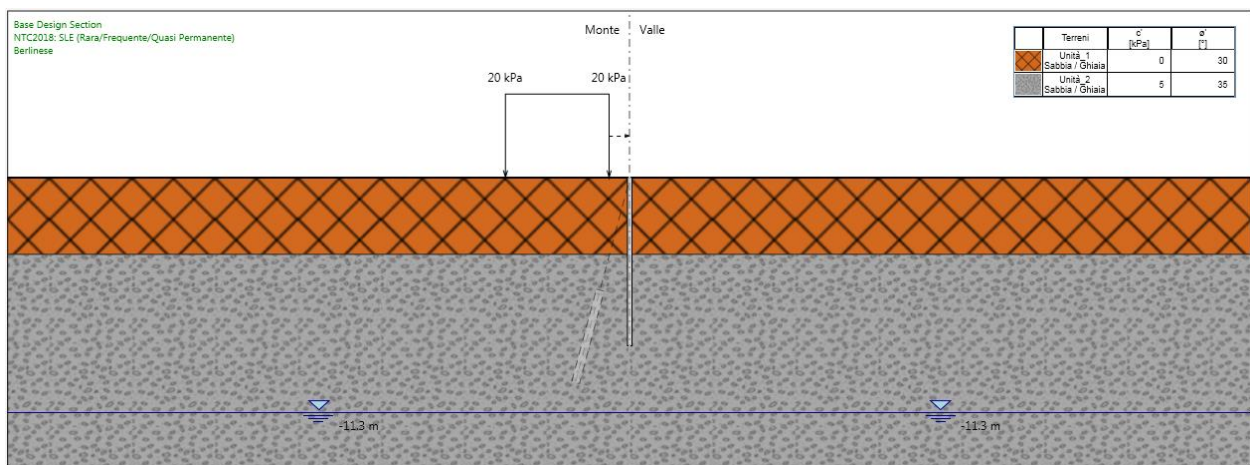
Figura 121.Fase 3: realizzazione berlinese di micropali
