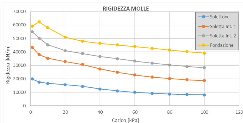
Figura 34. Andamento delle rigidezze
