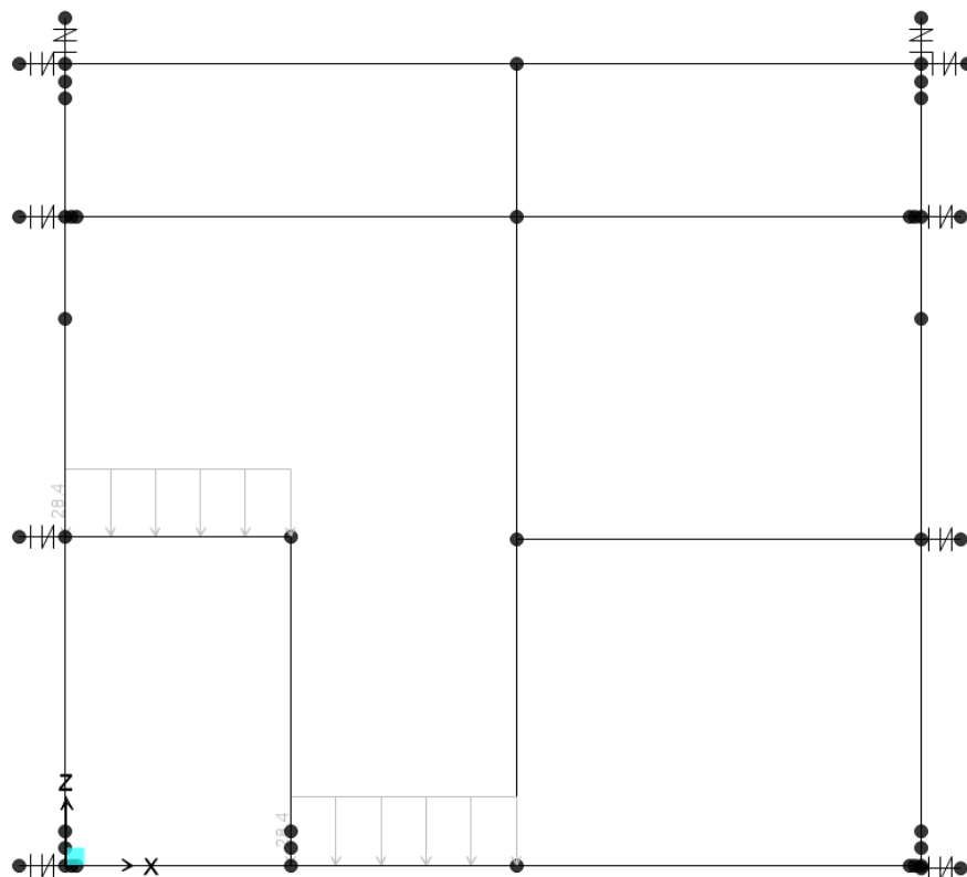
Figura 36.G2 carichi permanenti portati
