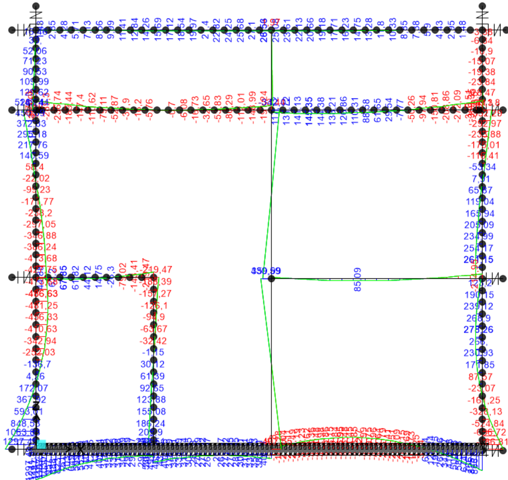
Figura 57.ENV M QUASI PERMANENTE
