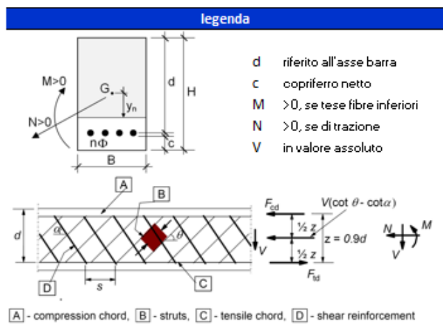
Figura 22. Verifica di resistenza strutturale della trave di coronamento in c.a.
