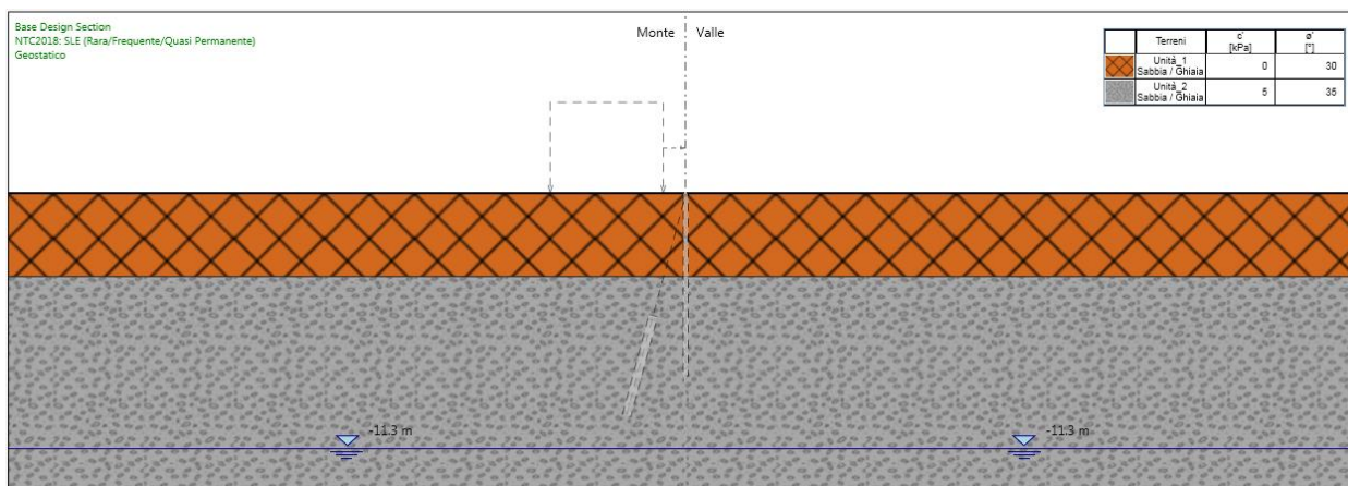
Figura 119.Fase 1: condizione geostatica
