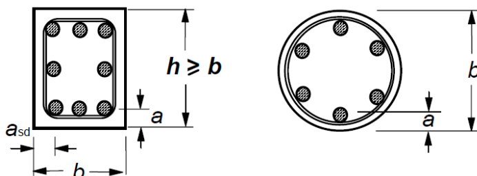
Figura 115. Sezioni degli elementi strutturali e distanza dall'asse a (UNI EN 1992-1-2:2005)
