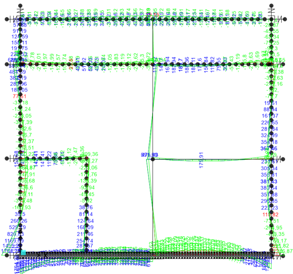
Figura 46.ENV M SLU/SLV
