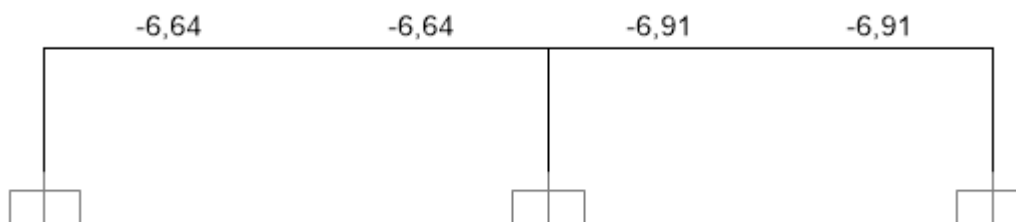
Figura 98. Modello portale soggetto a ritiro
