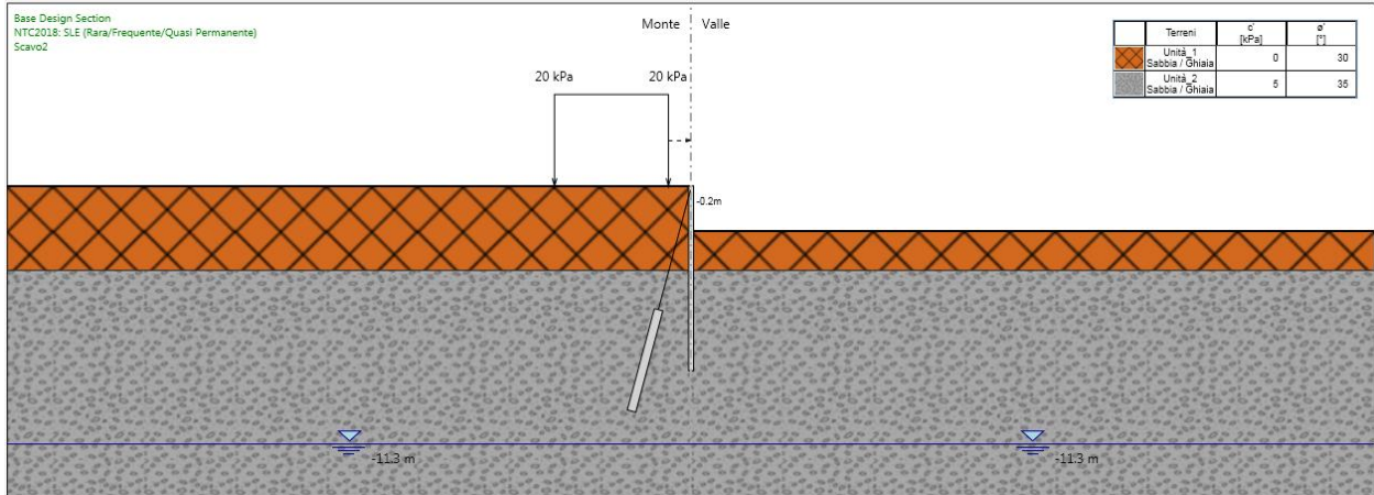
Figura 124.Fase 6: scavo a -2.0 m
