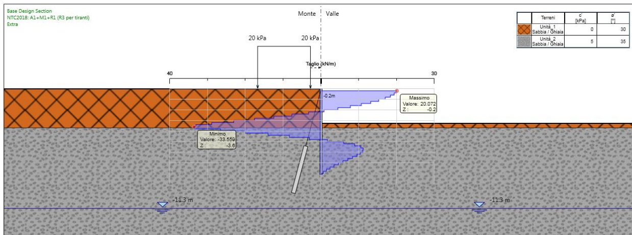
Figura 14. Involuppo del taglio sulla berlinese provvisoriale (A1+M1+R1)
