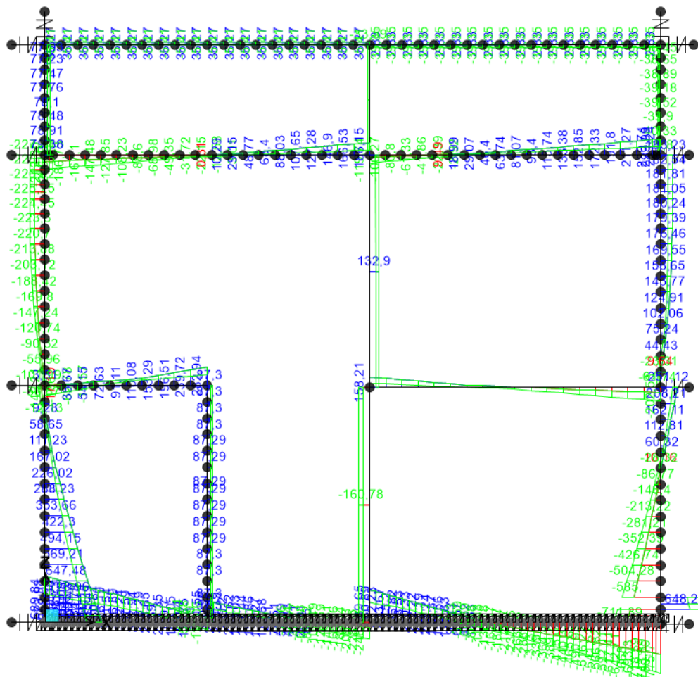
Figura 49.ENV V SLU/SLV
