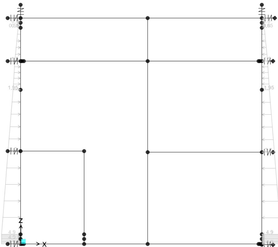
Figura 38.N SLU (terre)
