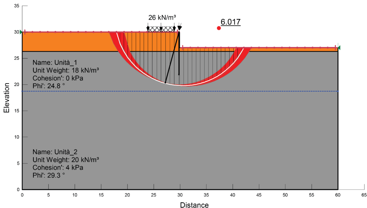
Figura 25.Verifica di stabilità globale della berlinese provvisoria in condizioni statiche
