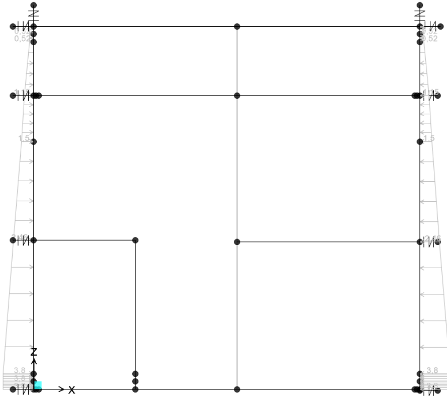
Figura 37.N sle (terre)
