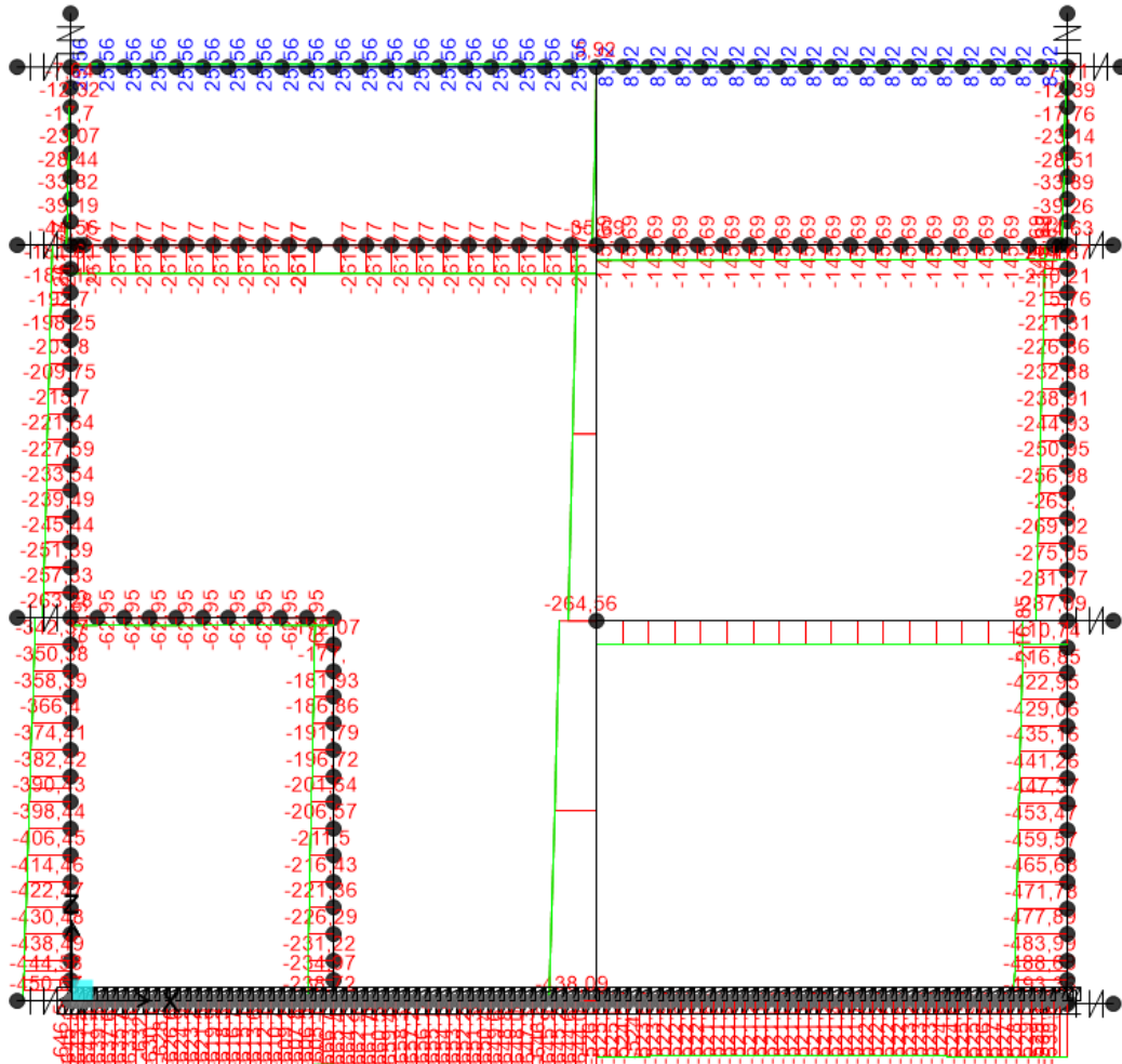
Figura 59.ENV N QUASI PERMANENTE
