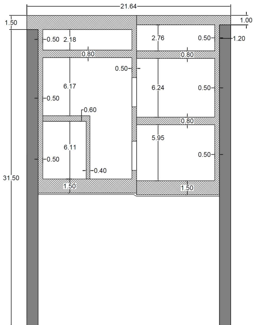
Figura 3. Esempio di sezione trasversale del pozzo Cimarosa / Tabacchi
