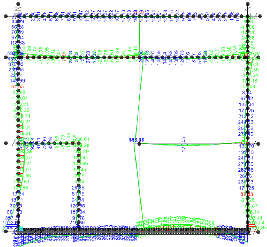
Figura 51.ENV M RARA
