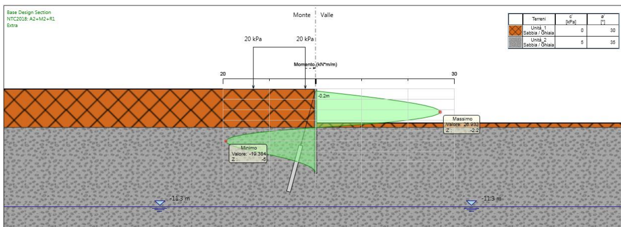
Figura 15. Involuppo dei momenti flettenti sulla berlinese provvisoriale (A2+M2+R1)
