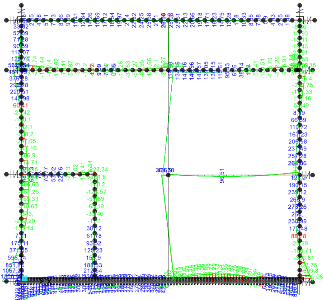
Figura 54.ENV M FREQUENTE
