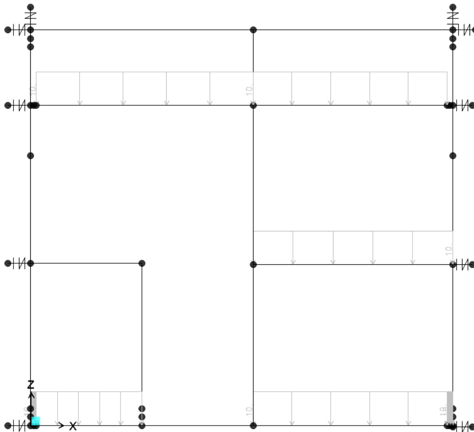
Figura 42.Q locali tecnici
