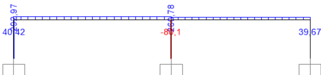
Figura 99. Trazione agente in soletta conseguente al ritiro
