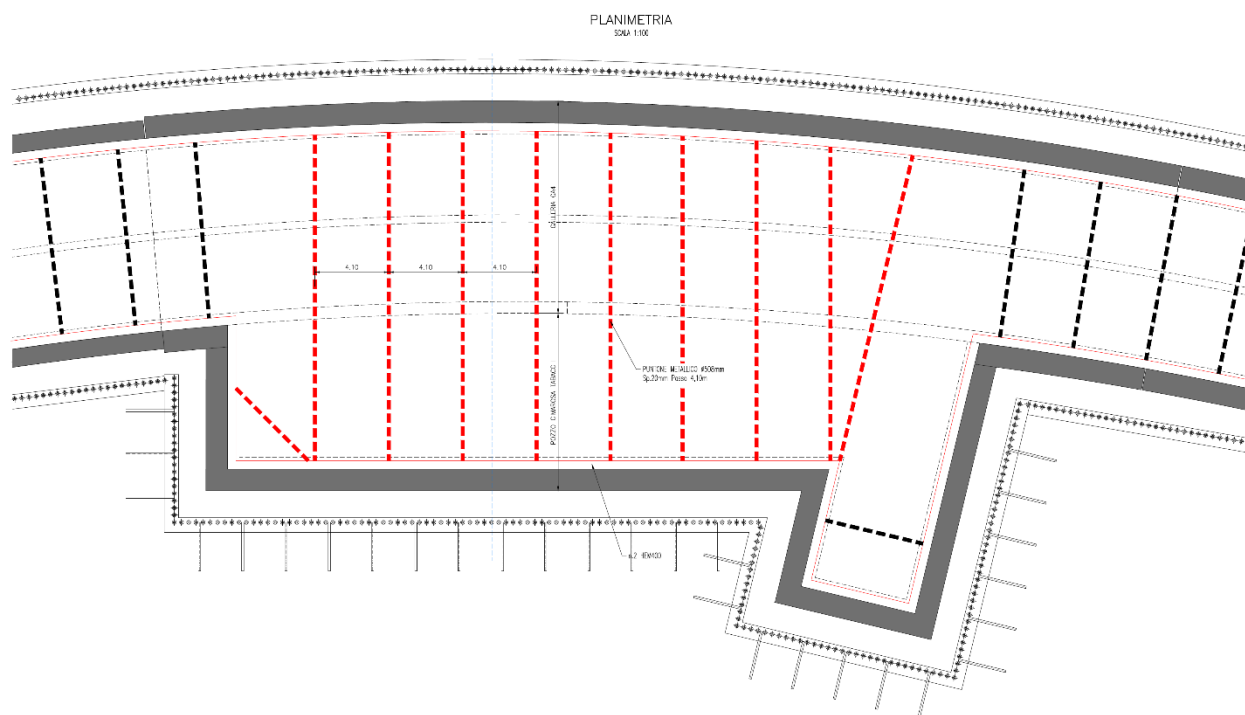
Figura 1. Planimetria pozzo Cimarosa / Tabacchi
