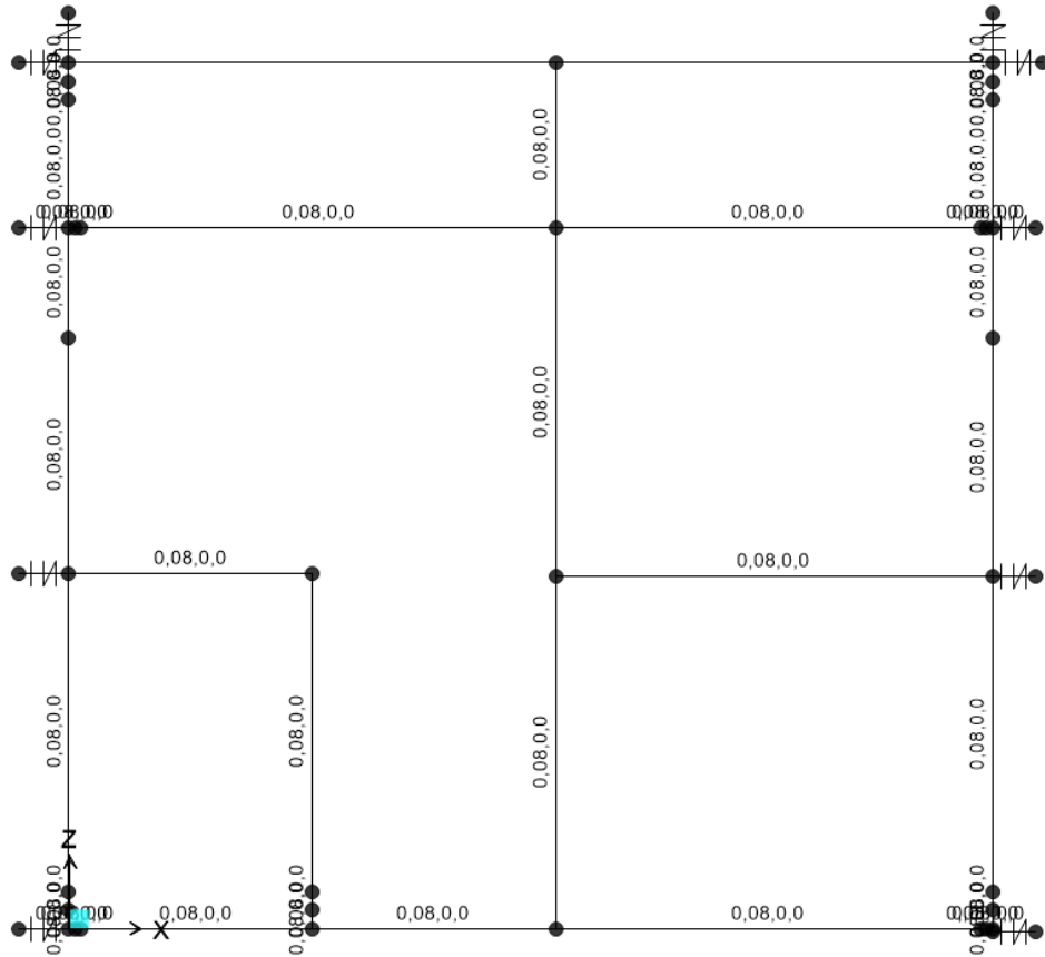
Figura 44.S3 inerzia sismica della struttura
