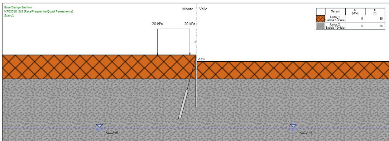
Figura 123.Fase 5: scavo a -1.0 m
