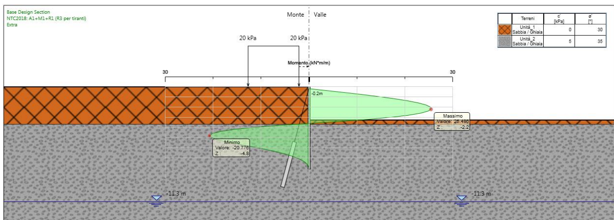
Figura 13. Involuppo dei momenti flettenti sulla berlinese provvisoria (A1+M1+R1)
