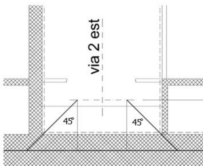
Figura 27. Distribuzione del carico sulla soletta
