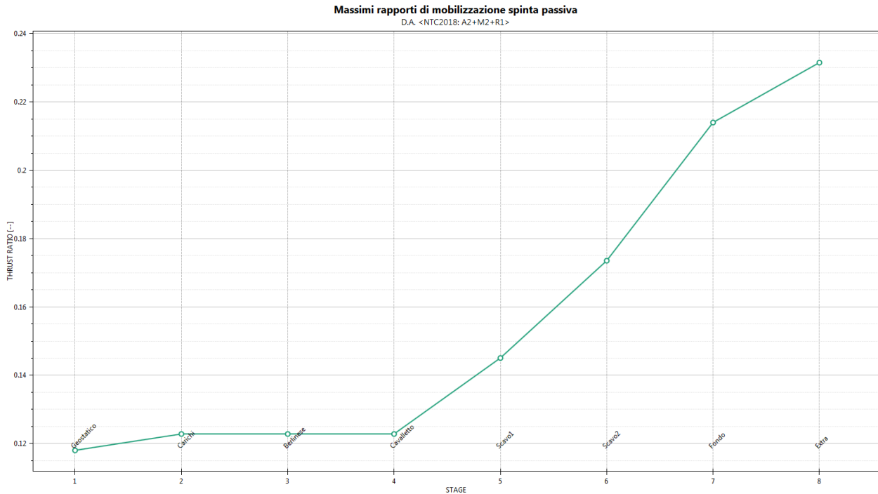
Figura 24. Resistenza passiva mobilitata in condizioni di stato limite ultimo (A2+M2+R1)
