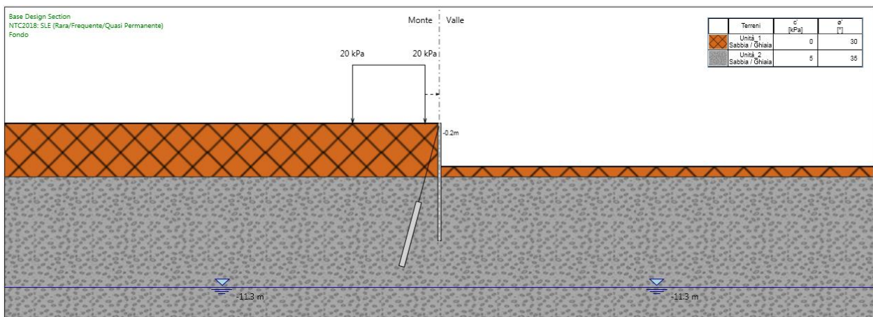
Figura 125.Fase 7: scavo a -3.0 m (fondo scavo)
