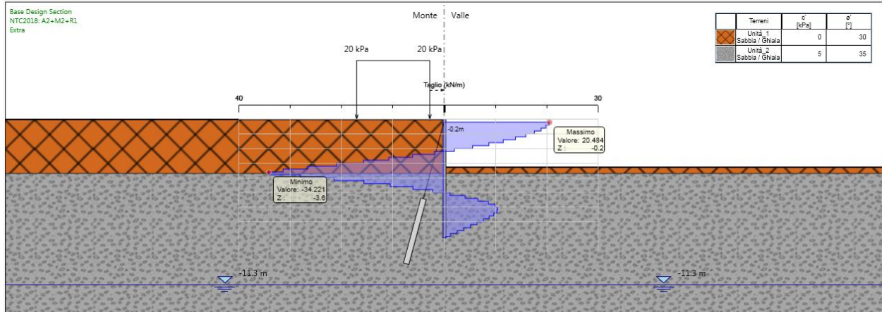
Figura 16. Involuppo del taglio sulla berlinese provvisoria (A2+M2+R1)
