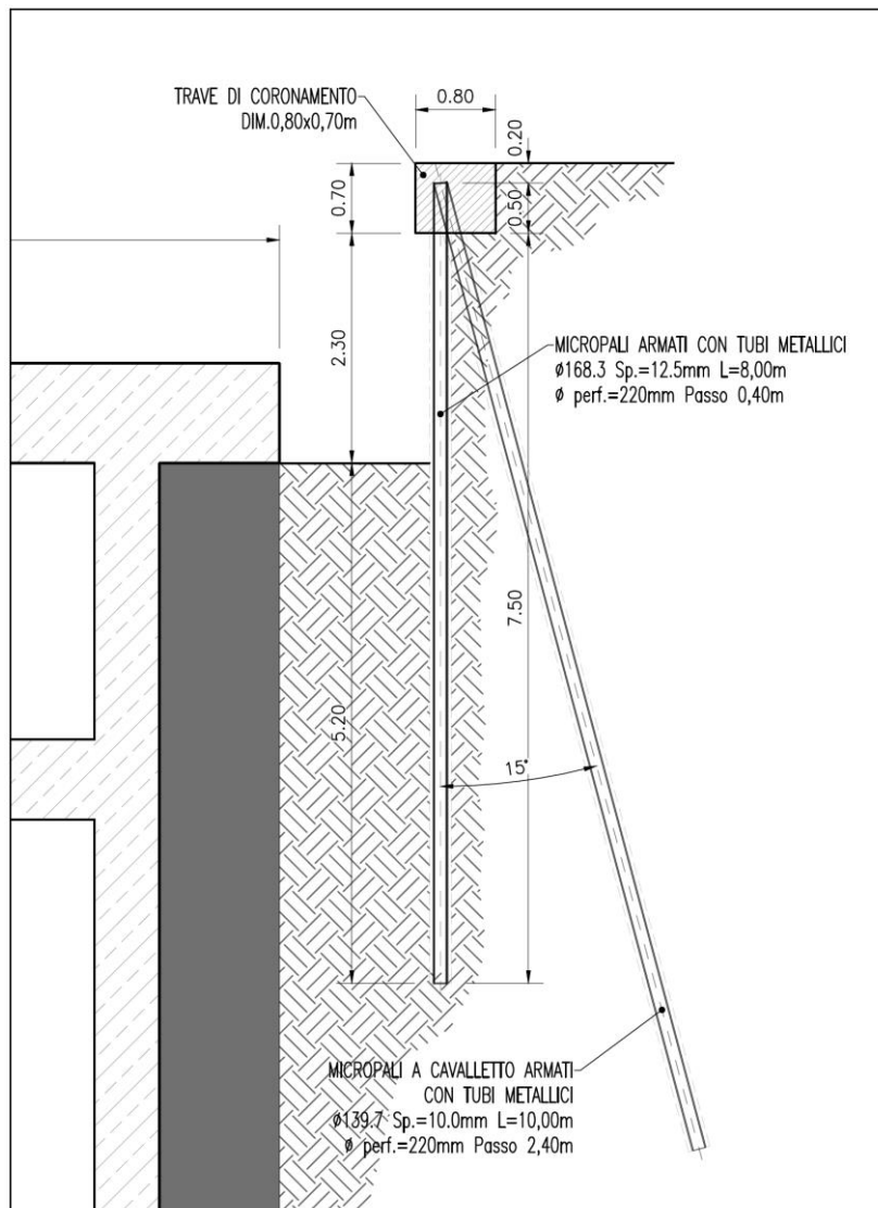
Figura 11. Rappresentazione grafica della berlinese oggetto di studio
