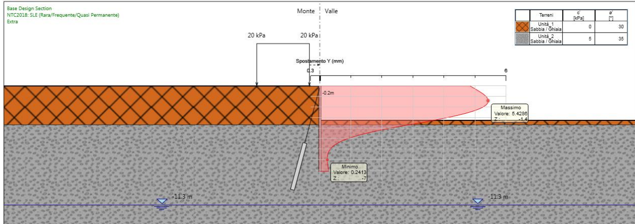
Figura 12. Involuppo degli spostamenti sulla berlinese provvisoria (SLE)
