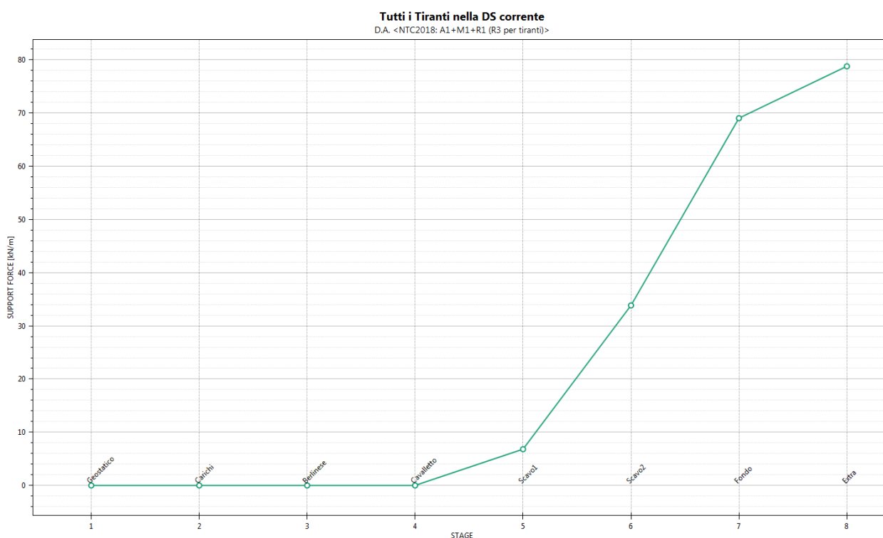
Figura 19. Andamento delle azioni nei micropali a cavalletto al variare delle fasi di calcolo (A1+M1+R3)
