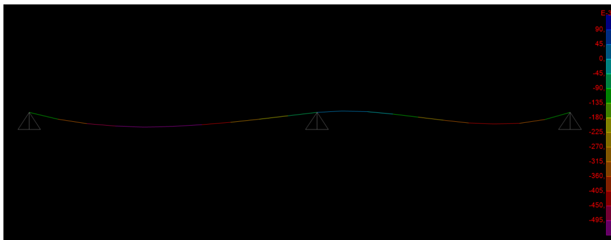
Figura 106. Deformata della soletta di copertura (SLE Rara)
