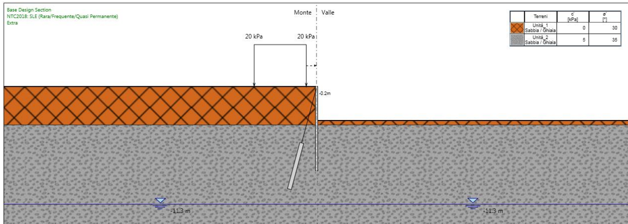
Figura 126.Fase 8: extra scavo da NTC 2018
