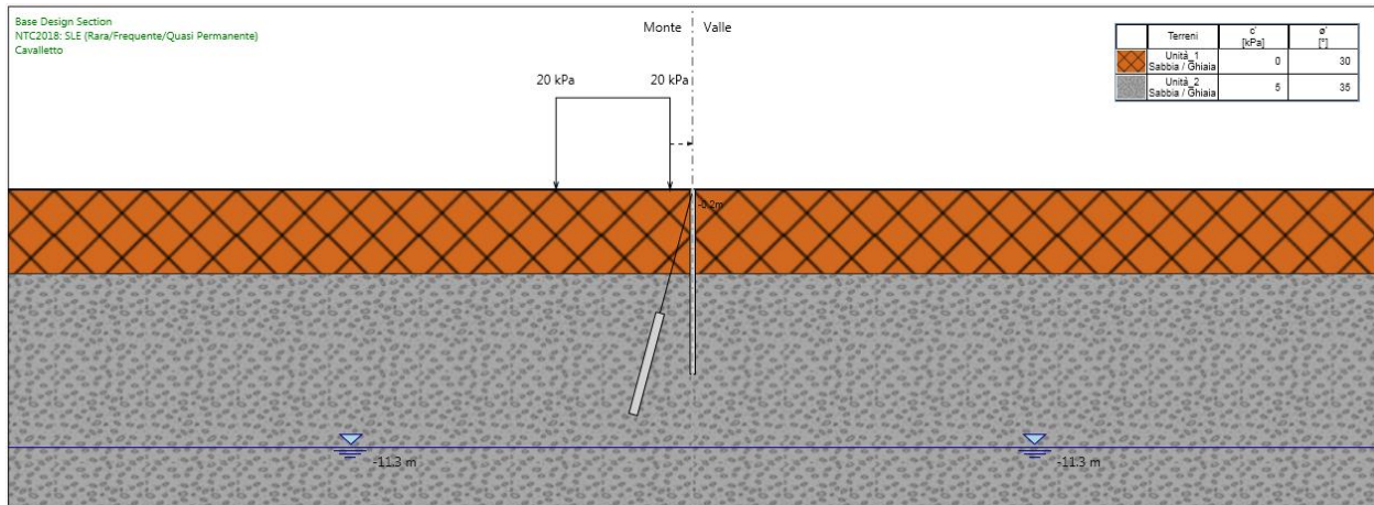
Figura 122.Fase 4: realizzazione micropali a cavalletto
