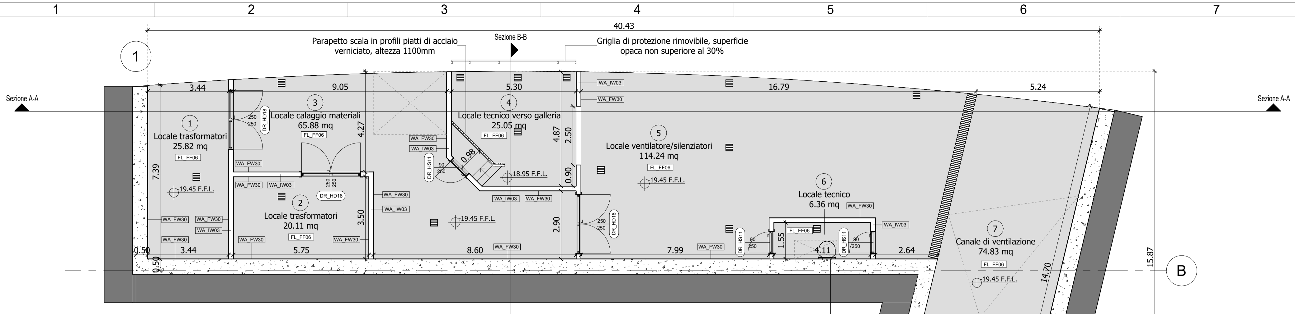
1 Piano secondo interrato (livello -2) 1 : 100
