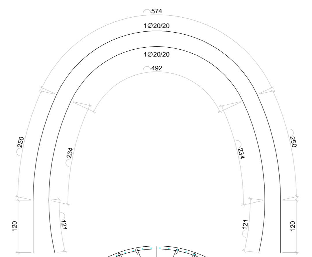
SEZIONE TRASVERSALE DI ARMATURA GALLERIA DI RACCORDO 1:50
