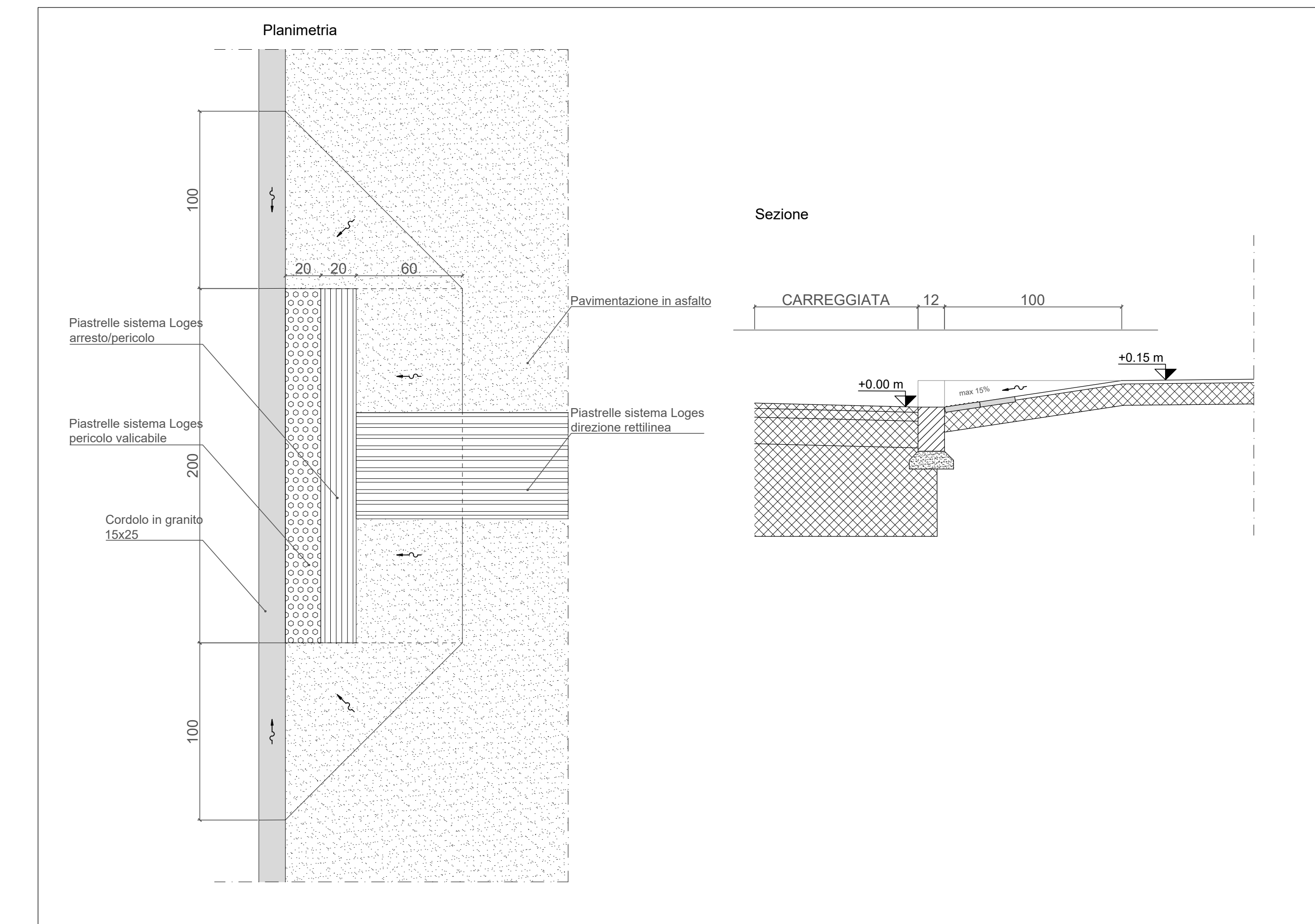
Particolare scivolo per abbattimento barriere architettoniche | Planimetria e sezione Scala 1:20
