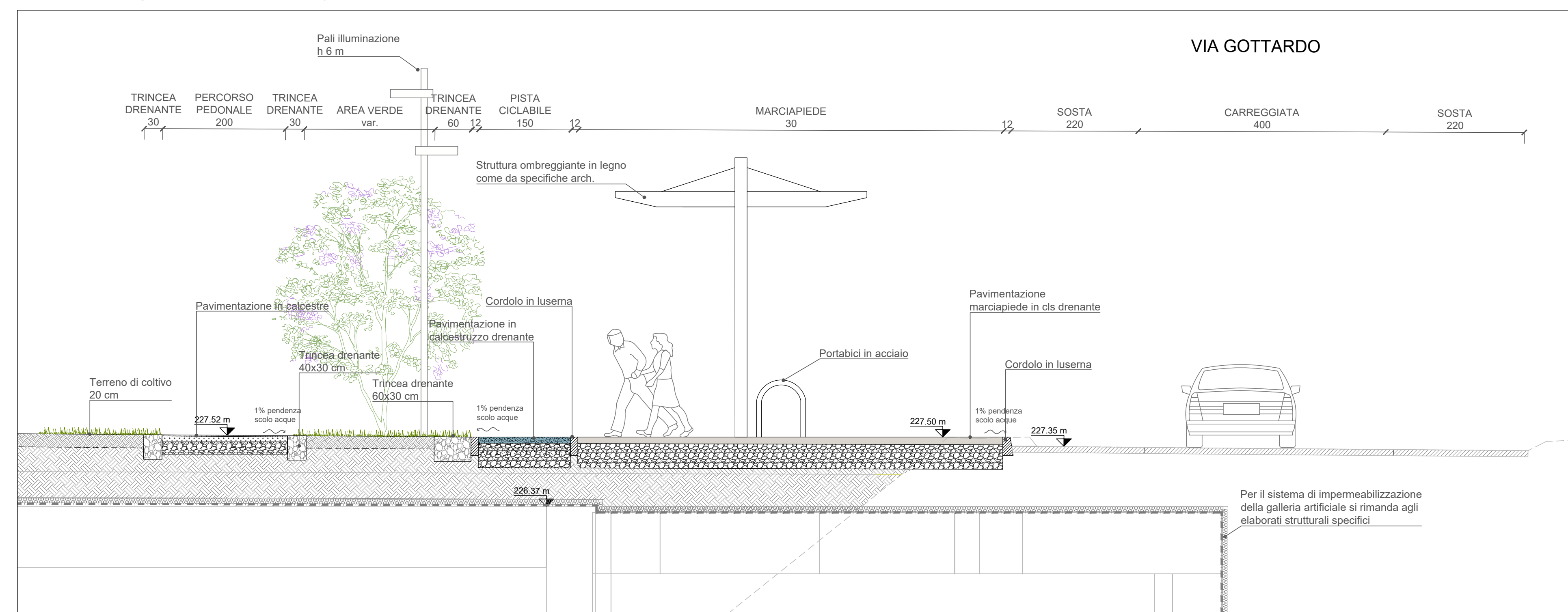
Sezione tipologica pozzo intertratta | Scala 1:50
