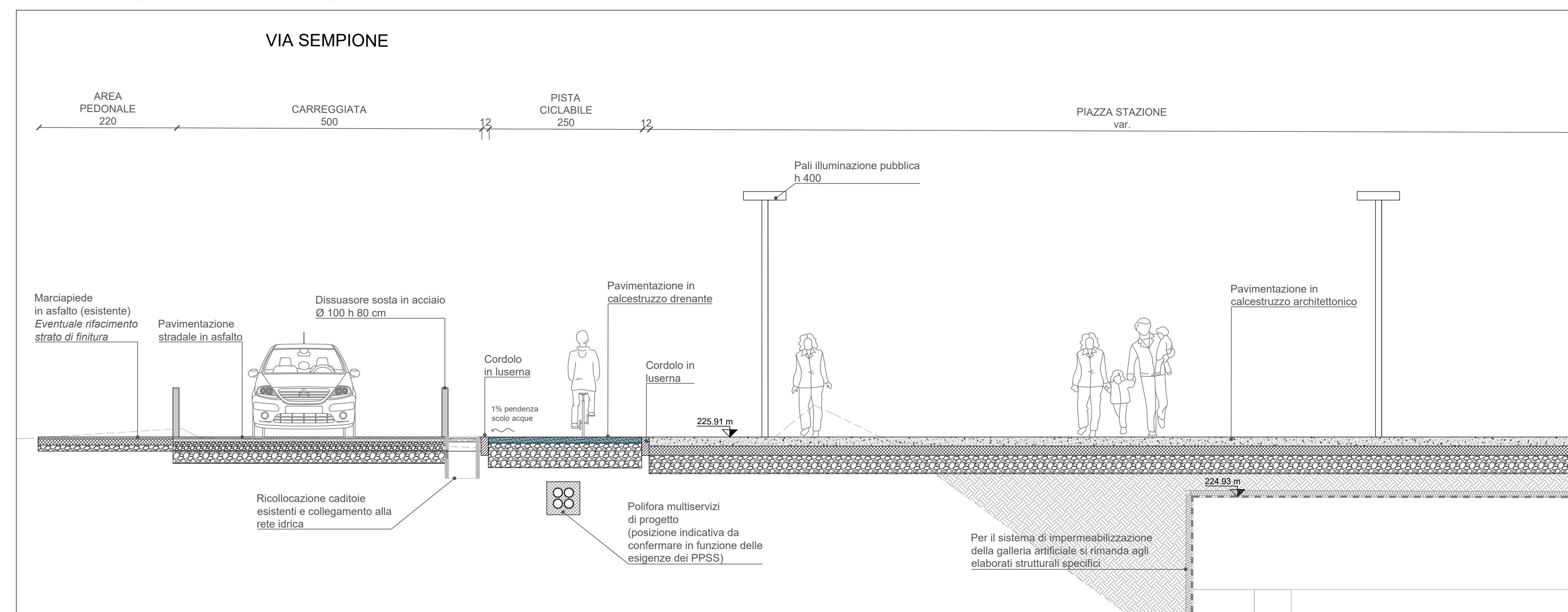
Sezione tipologica piazzale stazione | Scala 1:50
