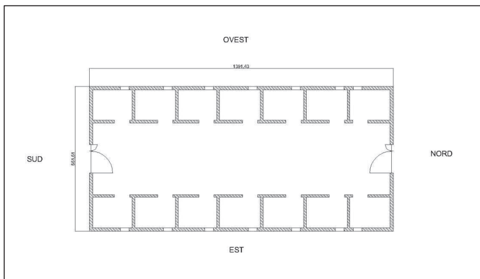
Pianta Box Canile
