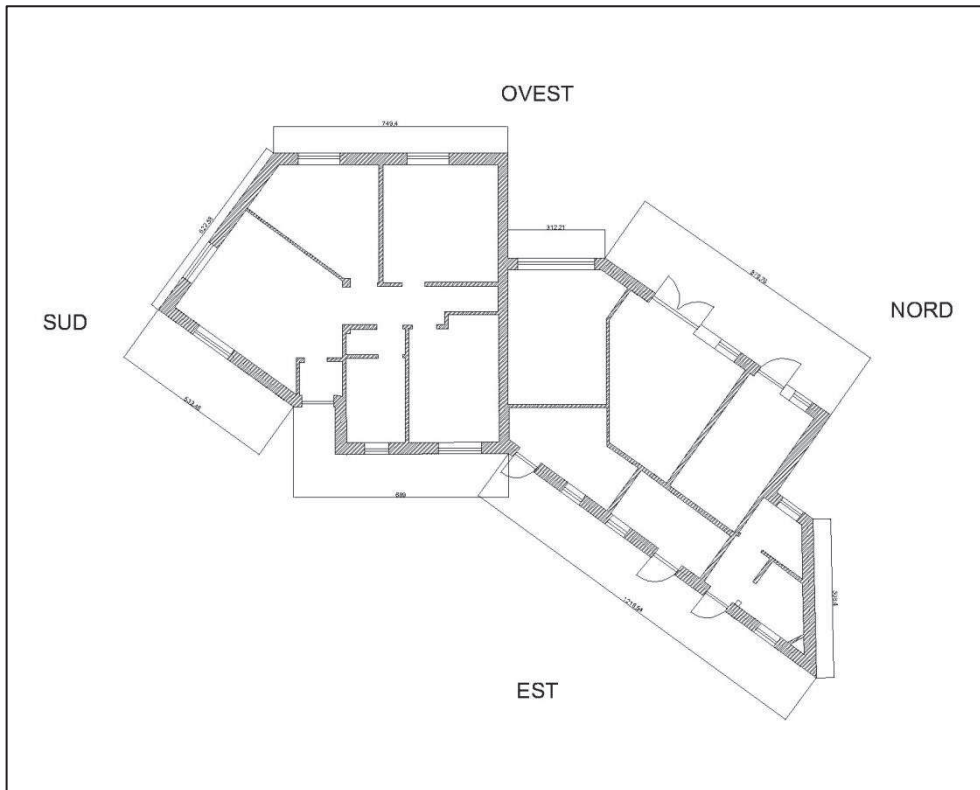
Pianta Edificio Gattile
