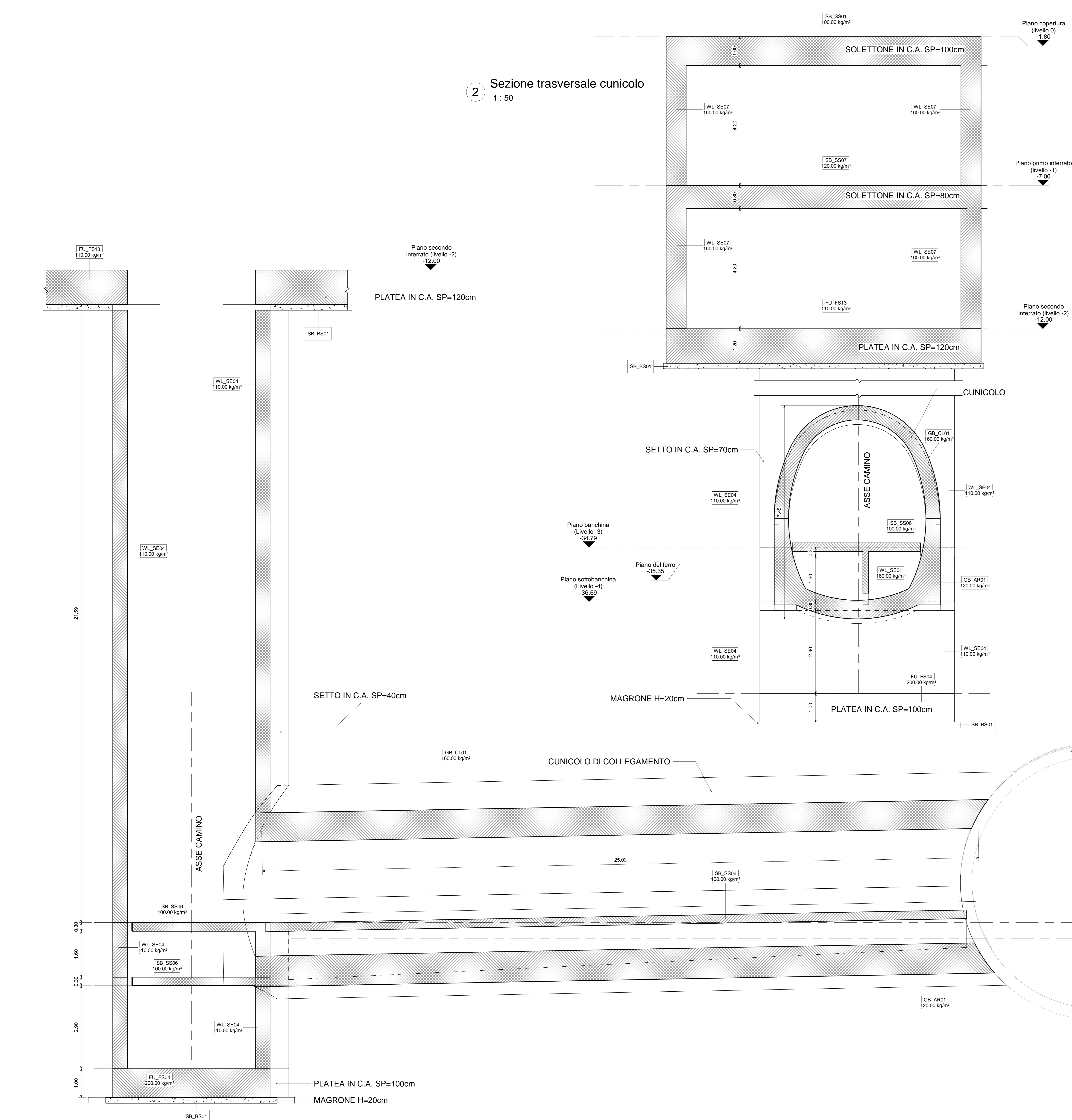
1 Sezione longitudinale cunicolo 1 : 50
