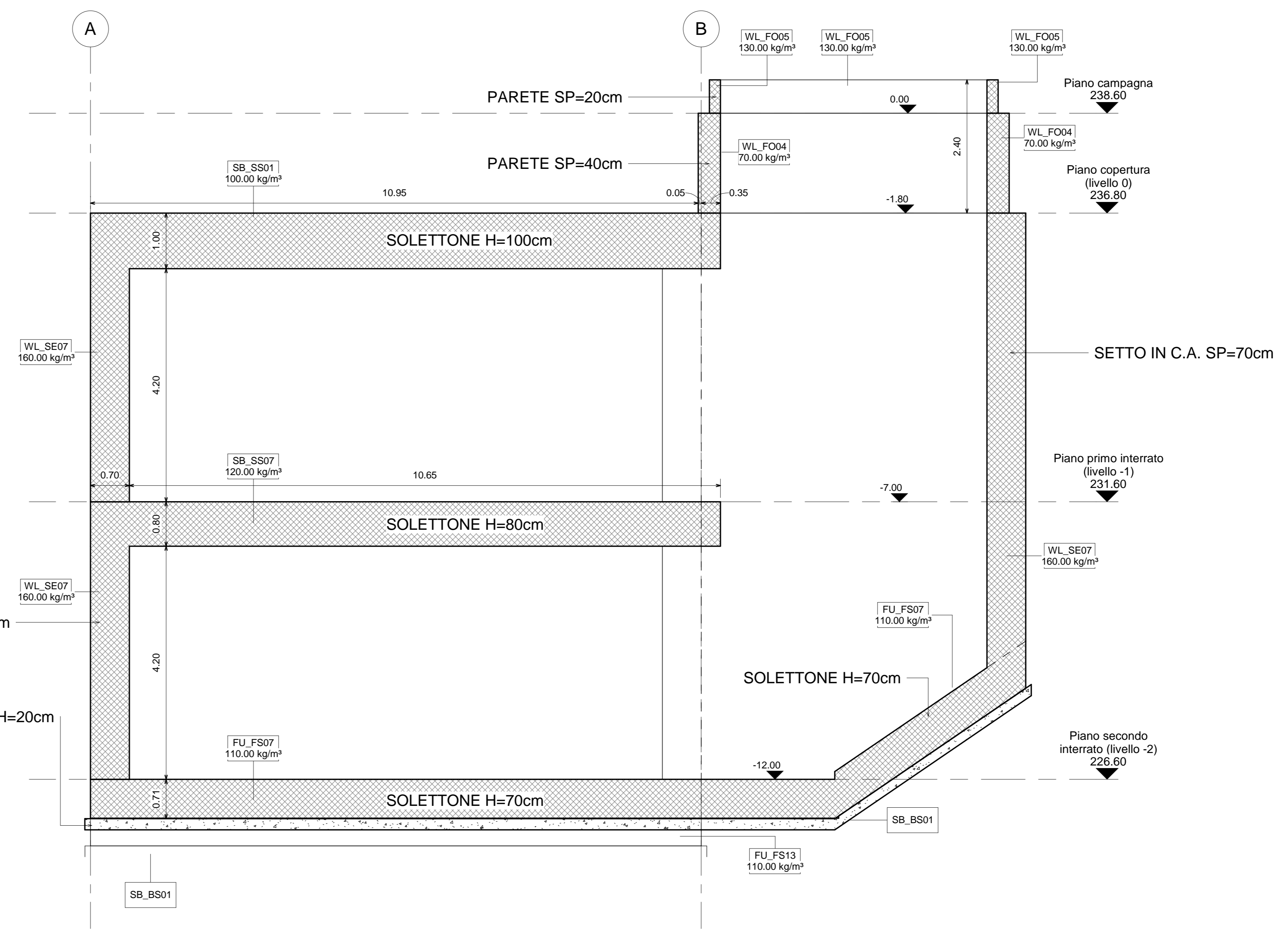
2 Sezione 4 1 : 50
