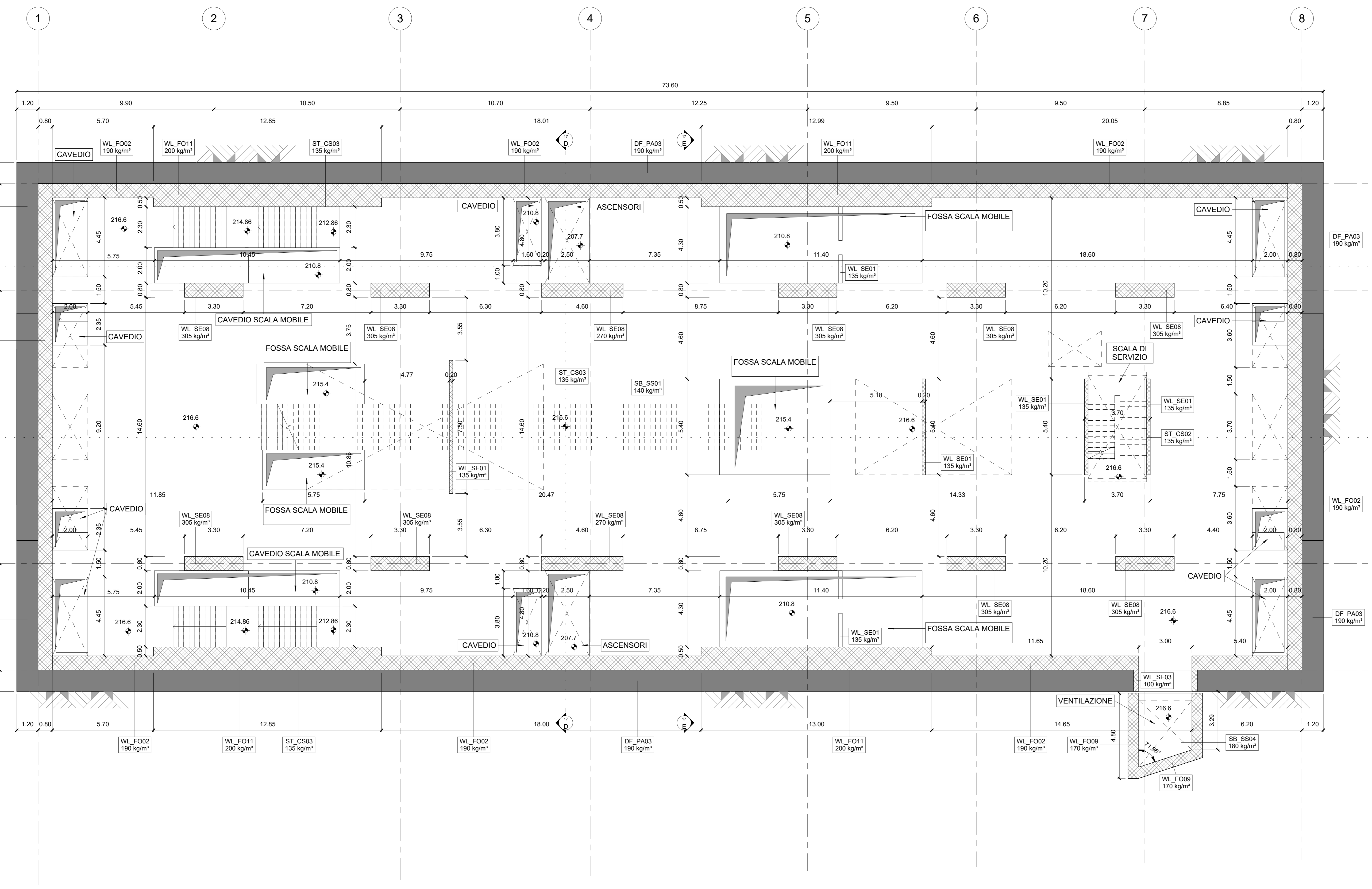
1 PIANTA MEZZANINO INFERIORE 1:100
