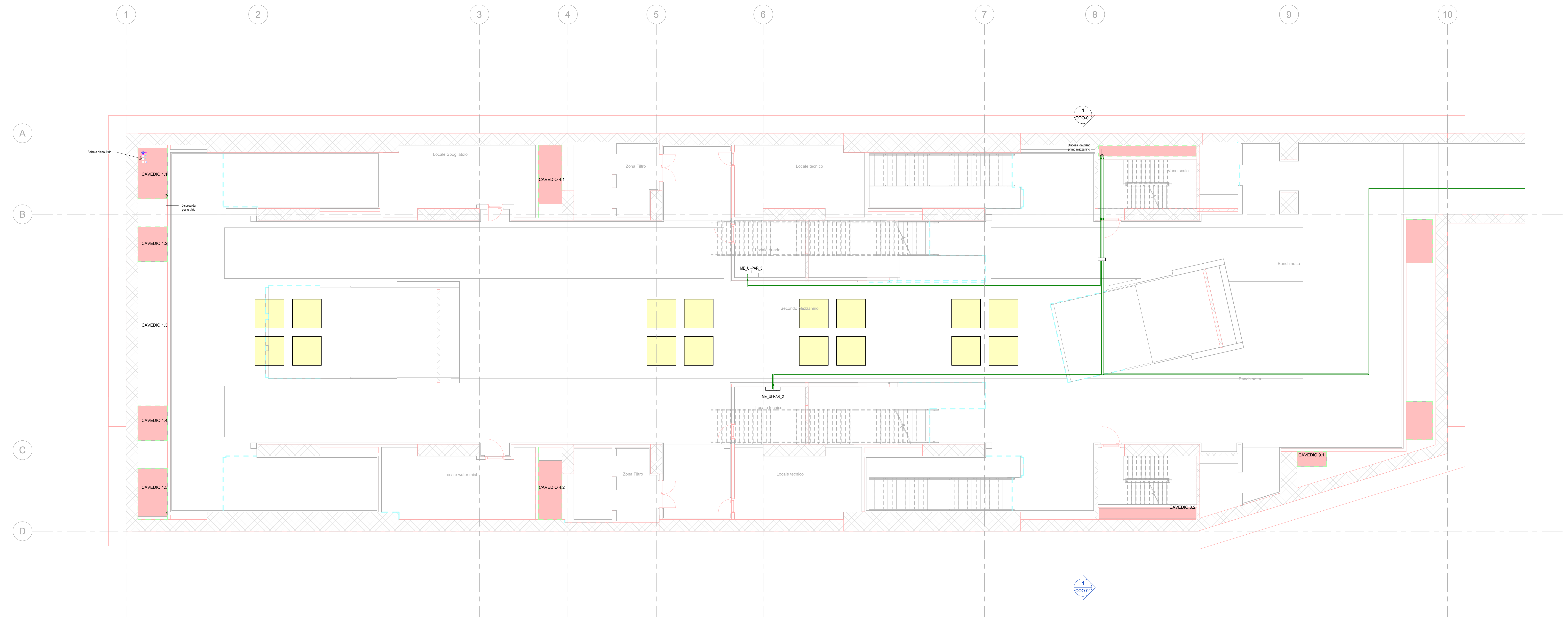
1 TR_Piano mezzanino (livello -3) 1 : 100
