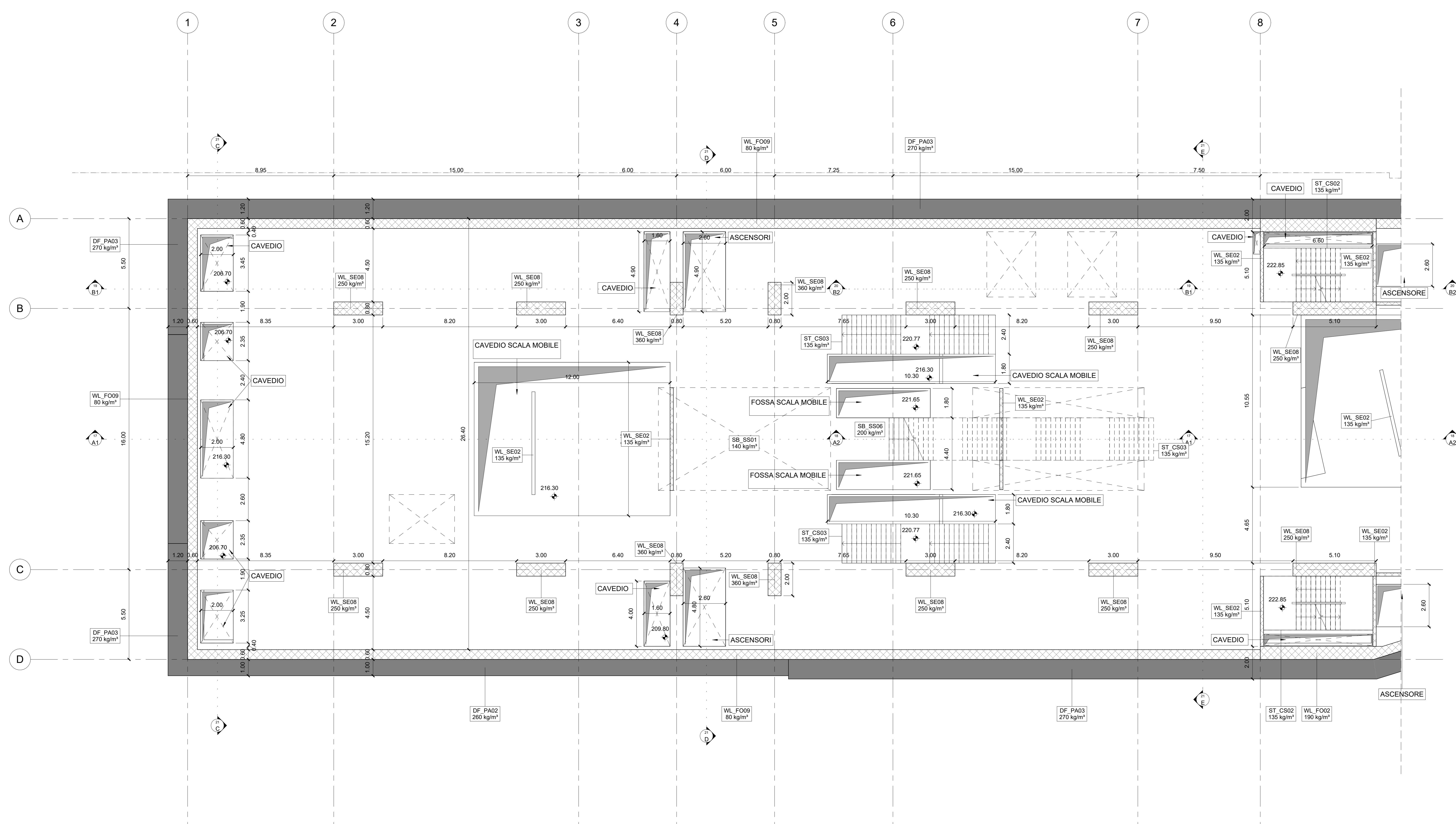
1 PIANO MEZZANINO SUPERIORE 1/2 1:100
