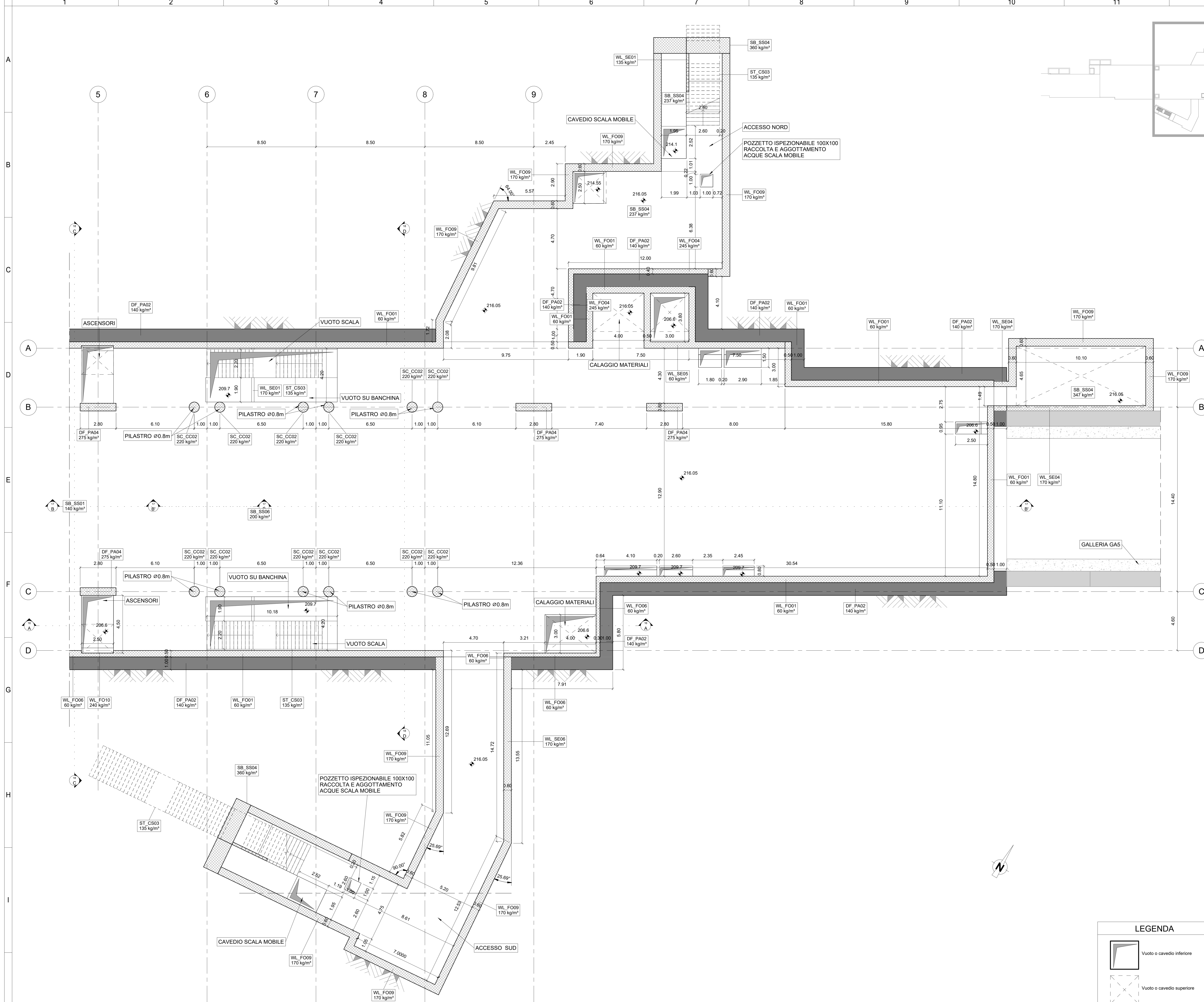
1 PIANTA ATRIO 2/2 1:100
