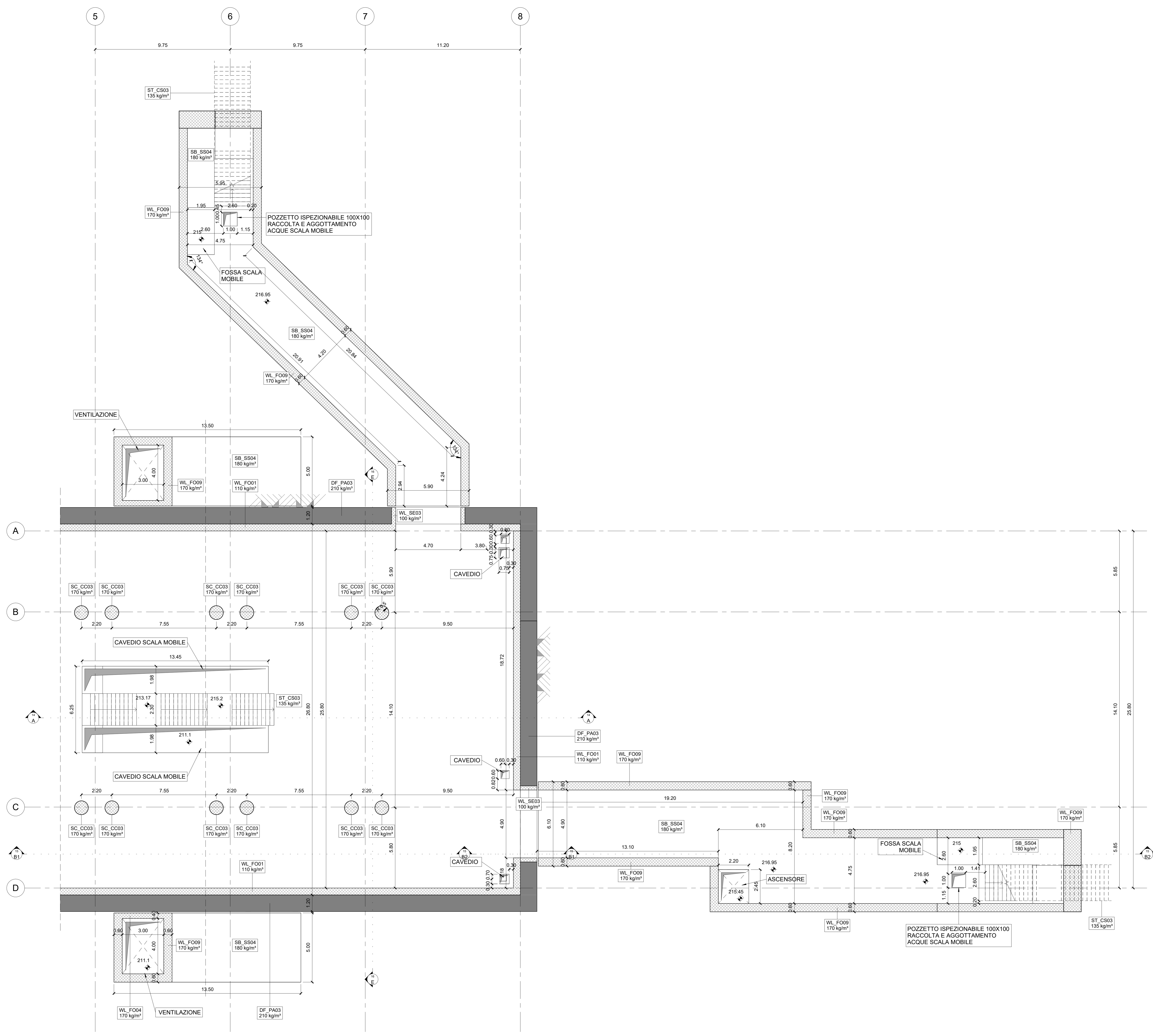
1 PIANO ATRIO 2/2 1 : 100
