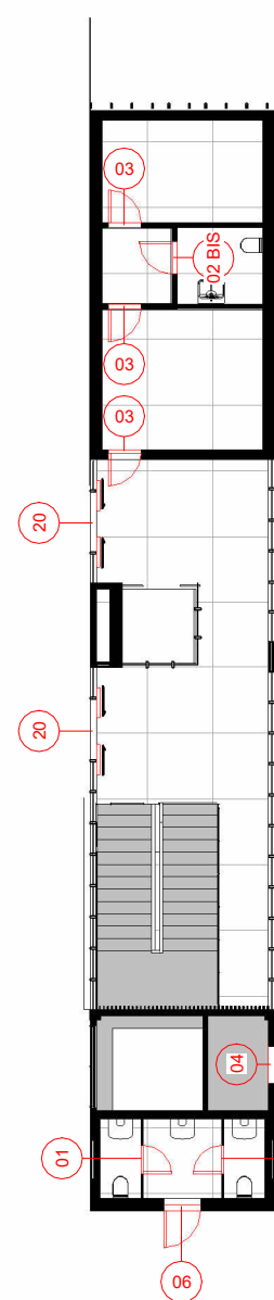
CORPO SCALA A LIVELLO +0 1 : 200
