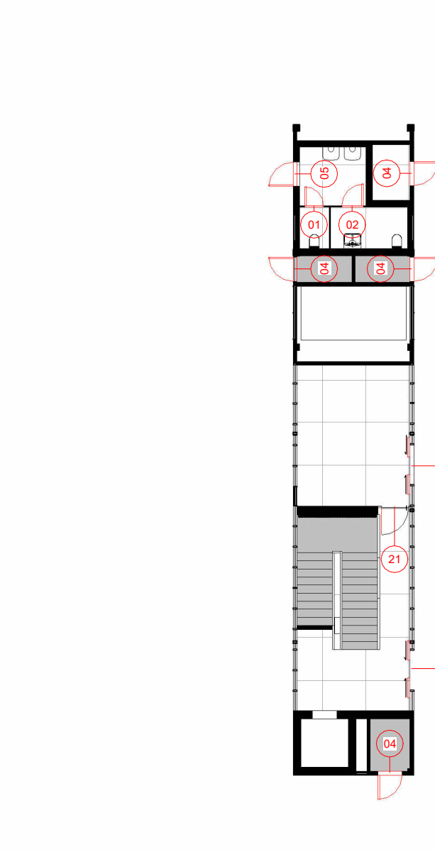
CORPO SCALA C LIVELLO +0 1 : 200
