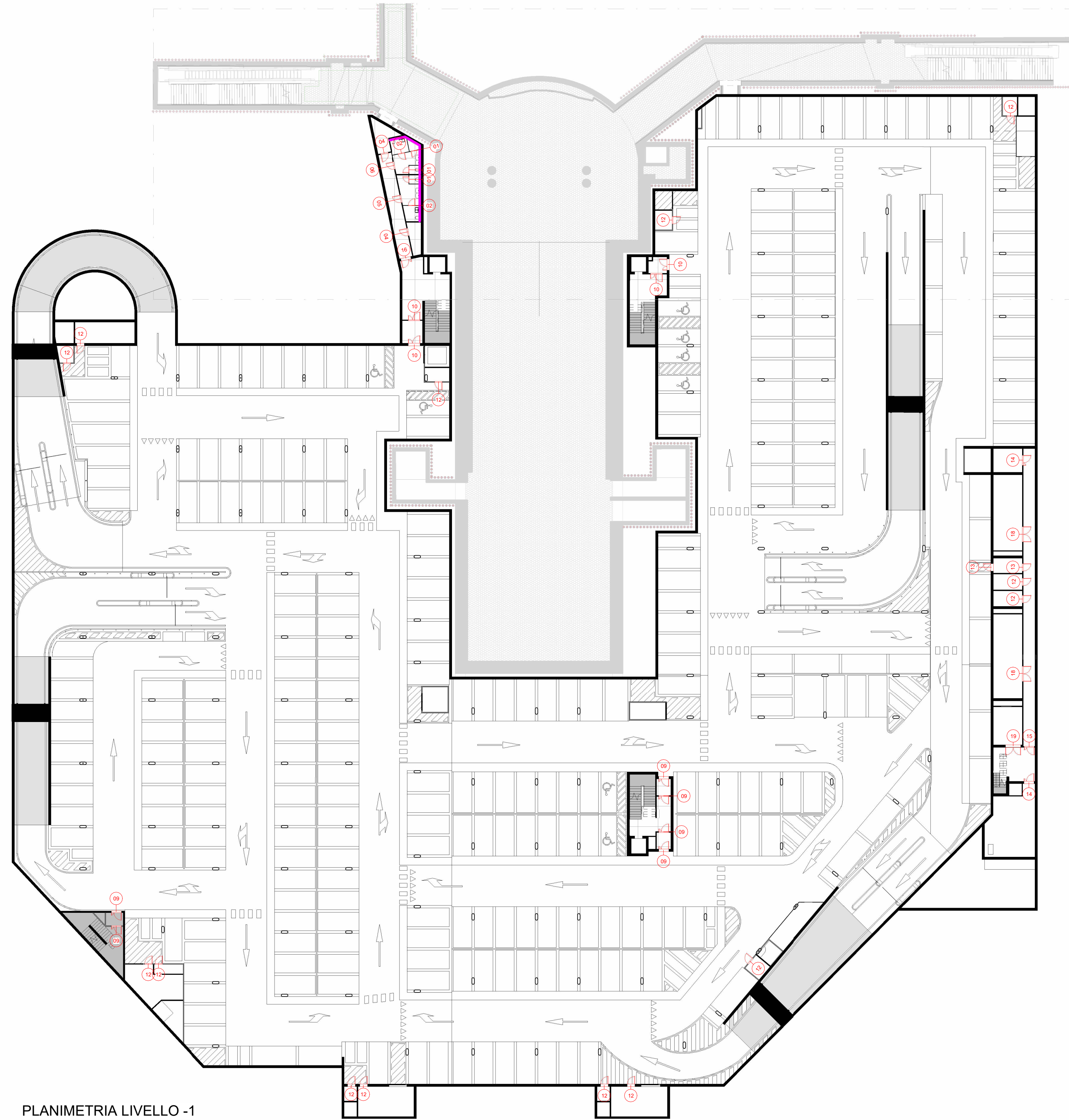
PLANIMETRIA LIVELLO -1 1 : 300
