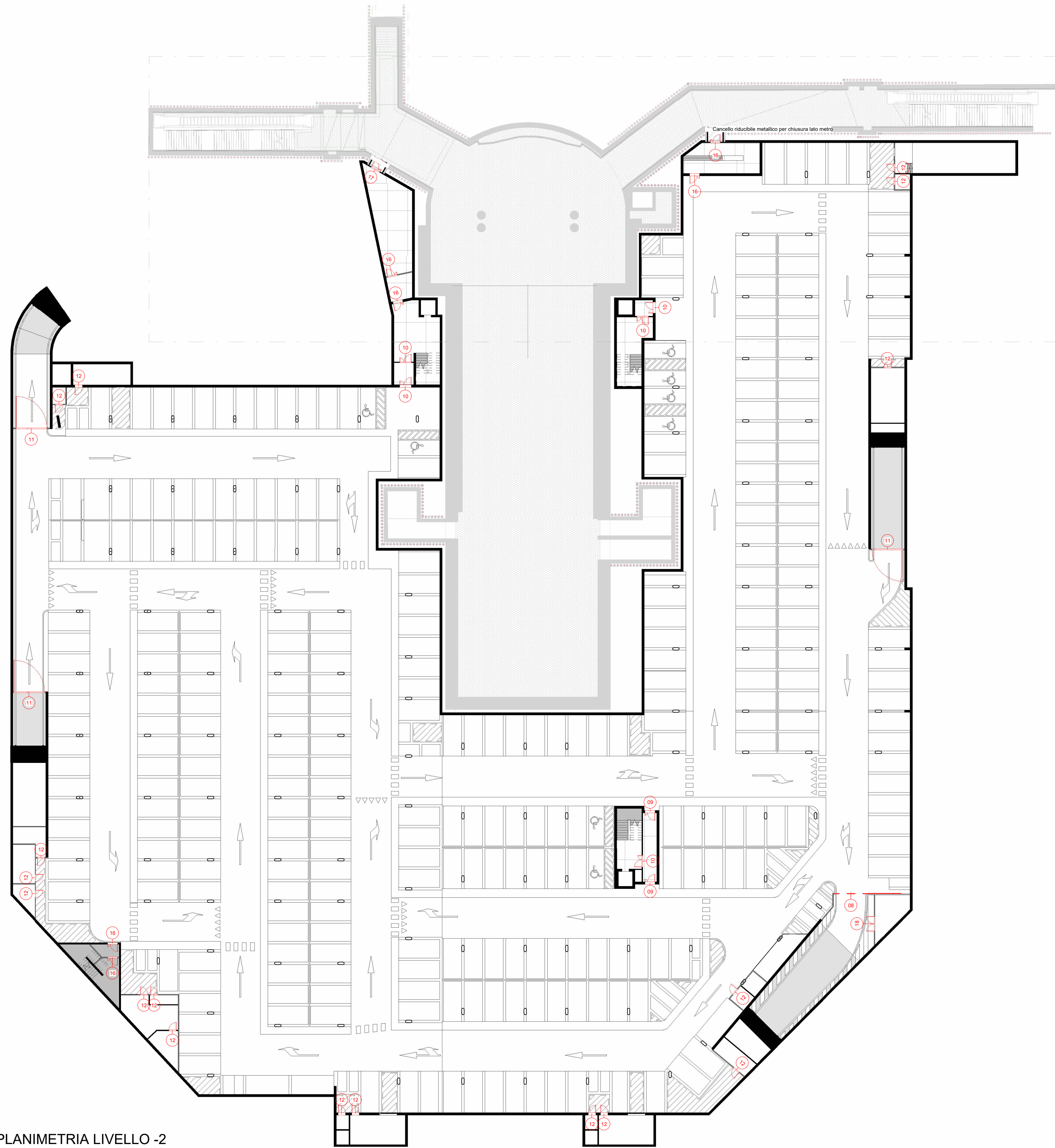
PLANIMETRIA LIVELLO -2 1 : 300
