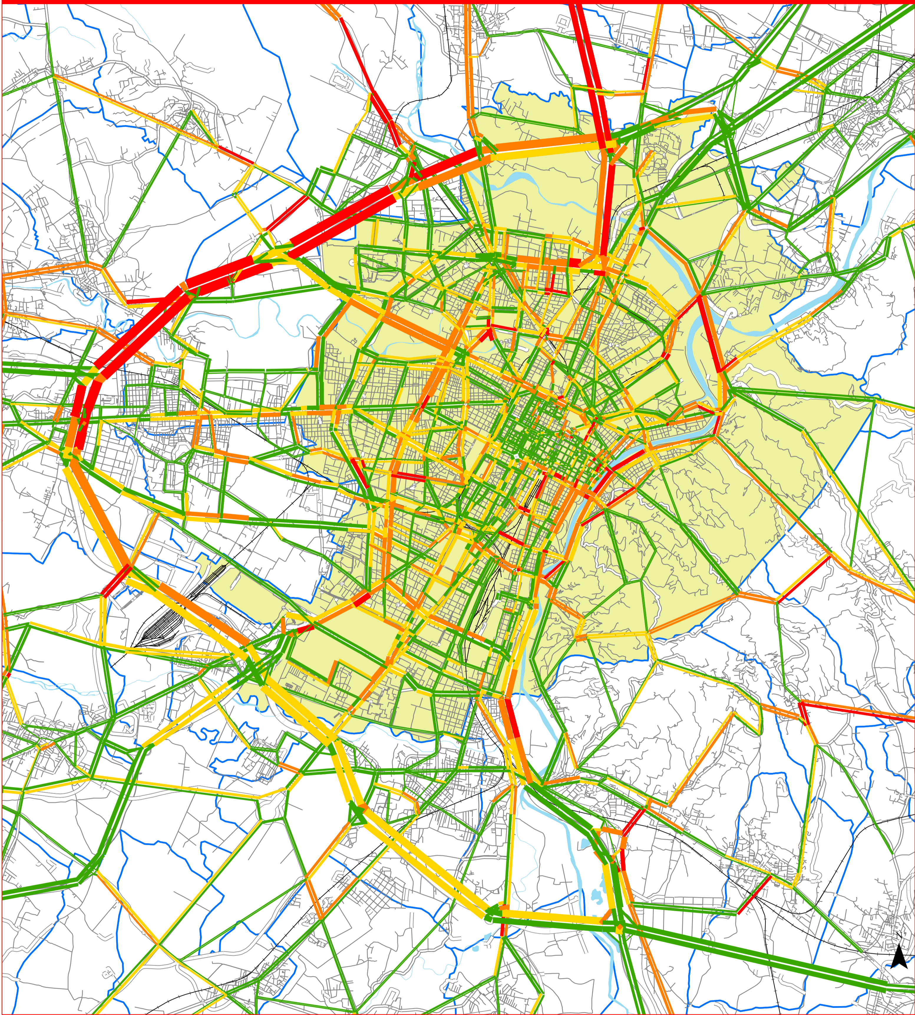
FLUSSI DI TRAFFICO E CRITICITA' GIORNATA STANDARD 2008 - ORA DI PUNTA DEL POMERIGGIO (17.00 - 18.00)
